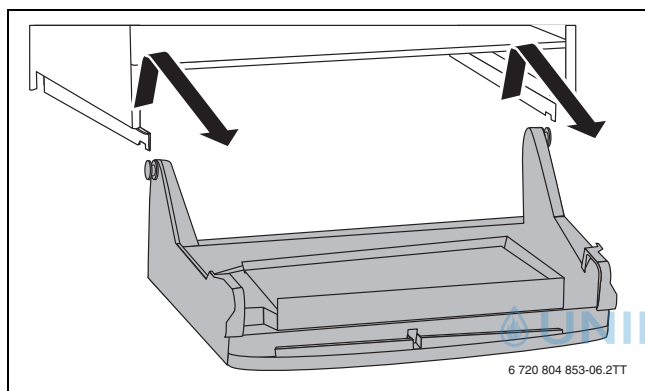
Bild 65 Steuergerät aushängen
