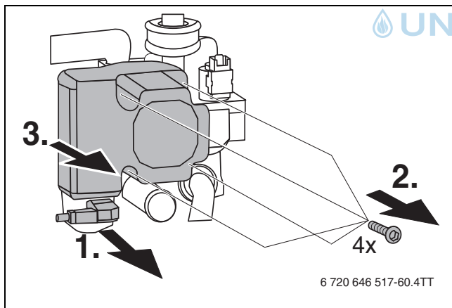
Bild 61 Heizungspumpe ausbauen
