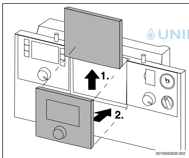
Bild 26 Abdeckung entfernen und Heizungsregler montieren
