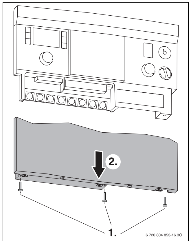
Bild 62 Abdeckung entfernen
