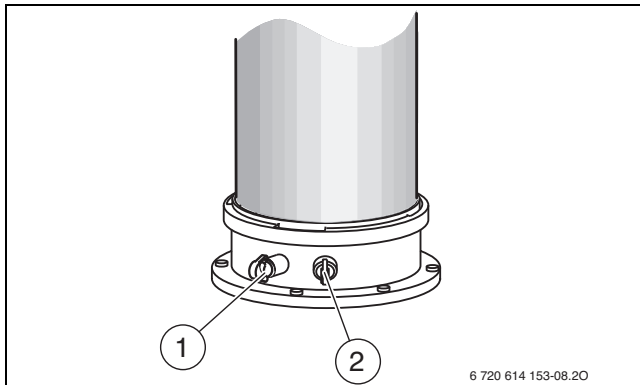
Bild 40 Abgasmessstutzen und Verbrennungsluft-Messstutzen
