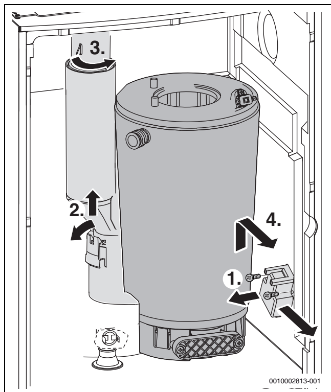
Bild 68 Wärmeblock ausbauen
