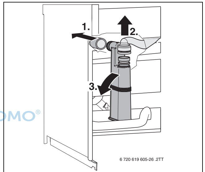
Bild 50 Kondensatsiphon ausbauen
