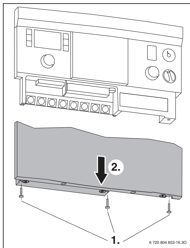
Bild 27 Abdeckung entfernen
