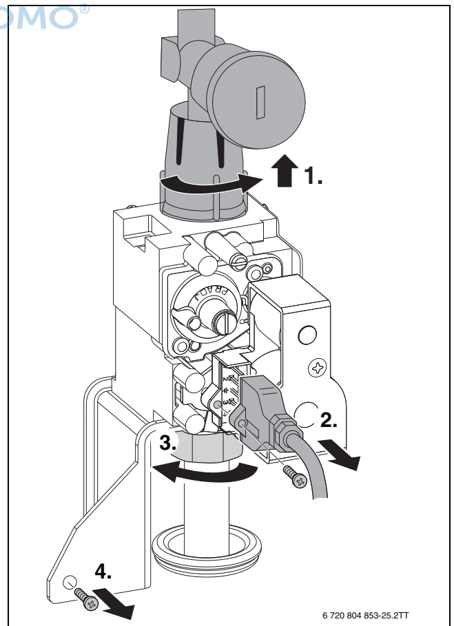
Bild 59 Gasarmatur ausbauen
