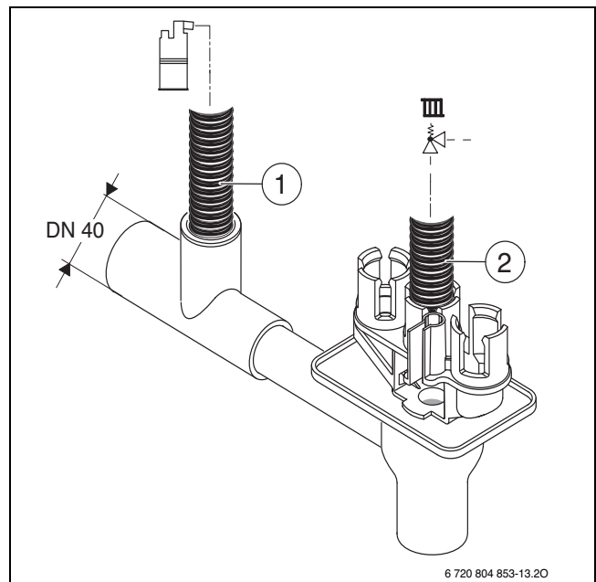
Bild 22 Kondensatschlauch und Schlauch vom Sicherheitsventil am Siphon montieren
