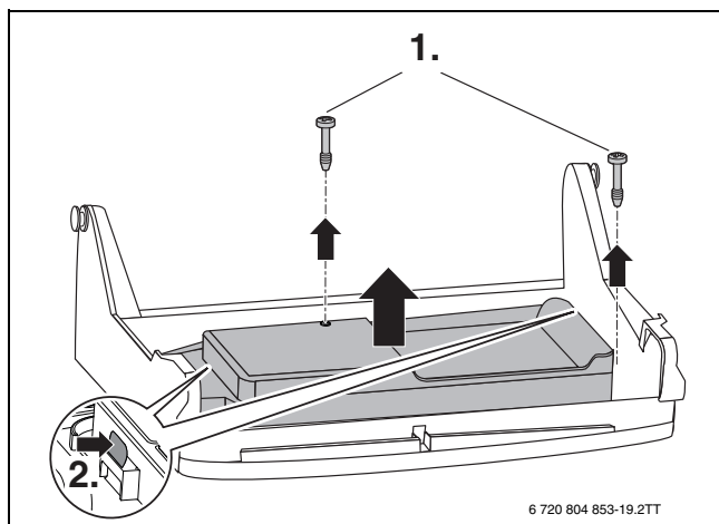
Bild 64 Abdeckung entfernen
