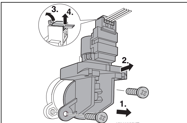
Bild 57 3-Wege-Ventil ausbauen
