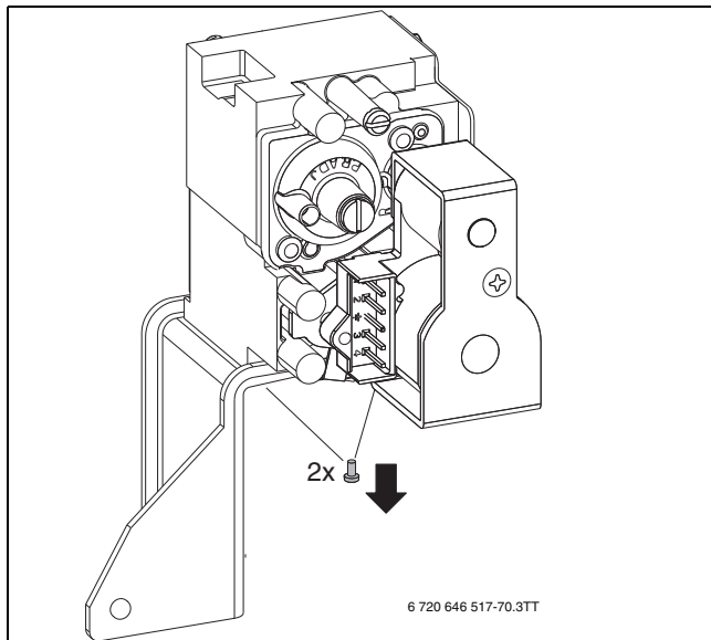
Bild 60 Gasarmatur ausbauen
