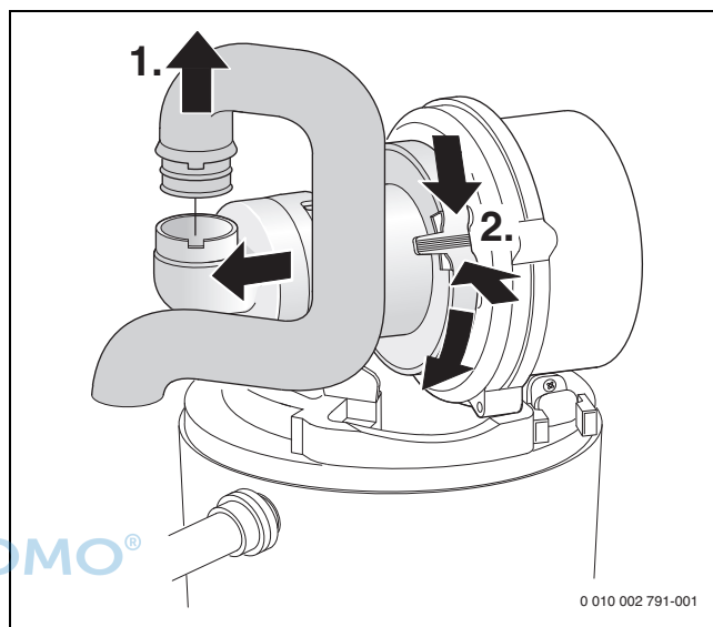
Bild 42 Saugrohr und Mischeinrichtung ausbauen
