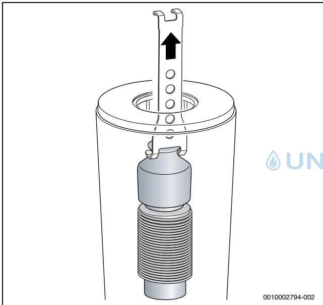
Bild 45 Oberen Verdrängungskörper herausnehmen
