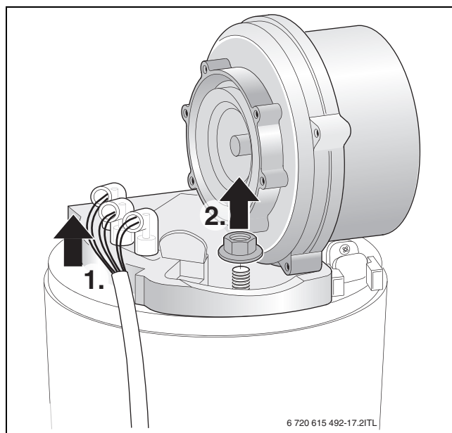
Bild 43 Gebläse herausnehmen
