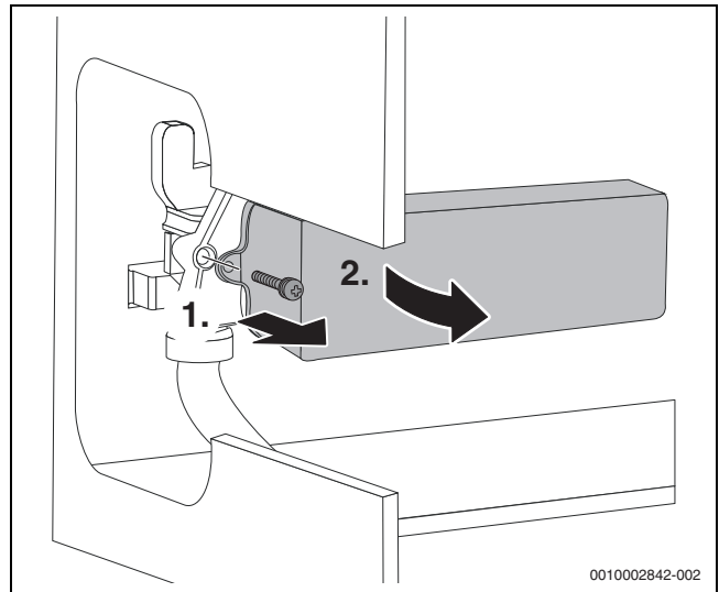
Bild 54 Plattenwärmetauscher ausbauen
