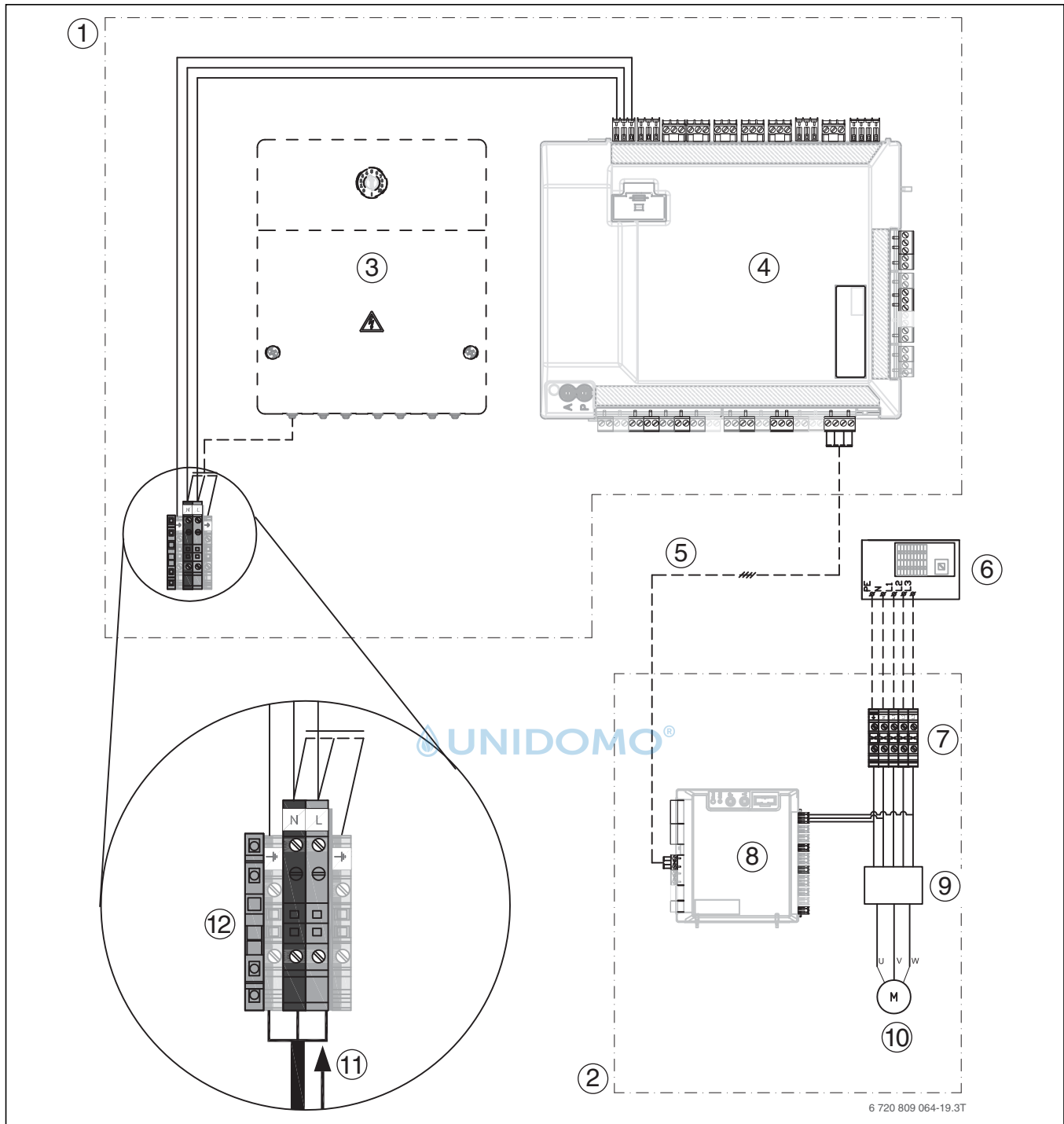
Bild 30 Inneneinheit mit externem Zuheiz – Überblick
