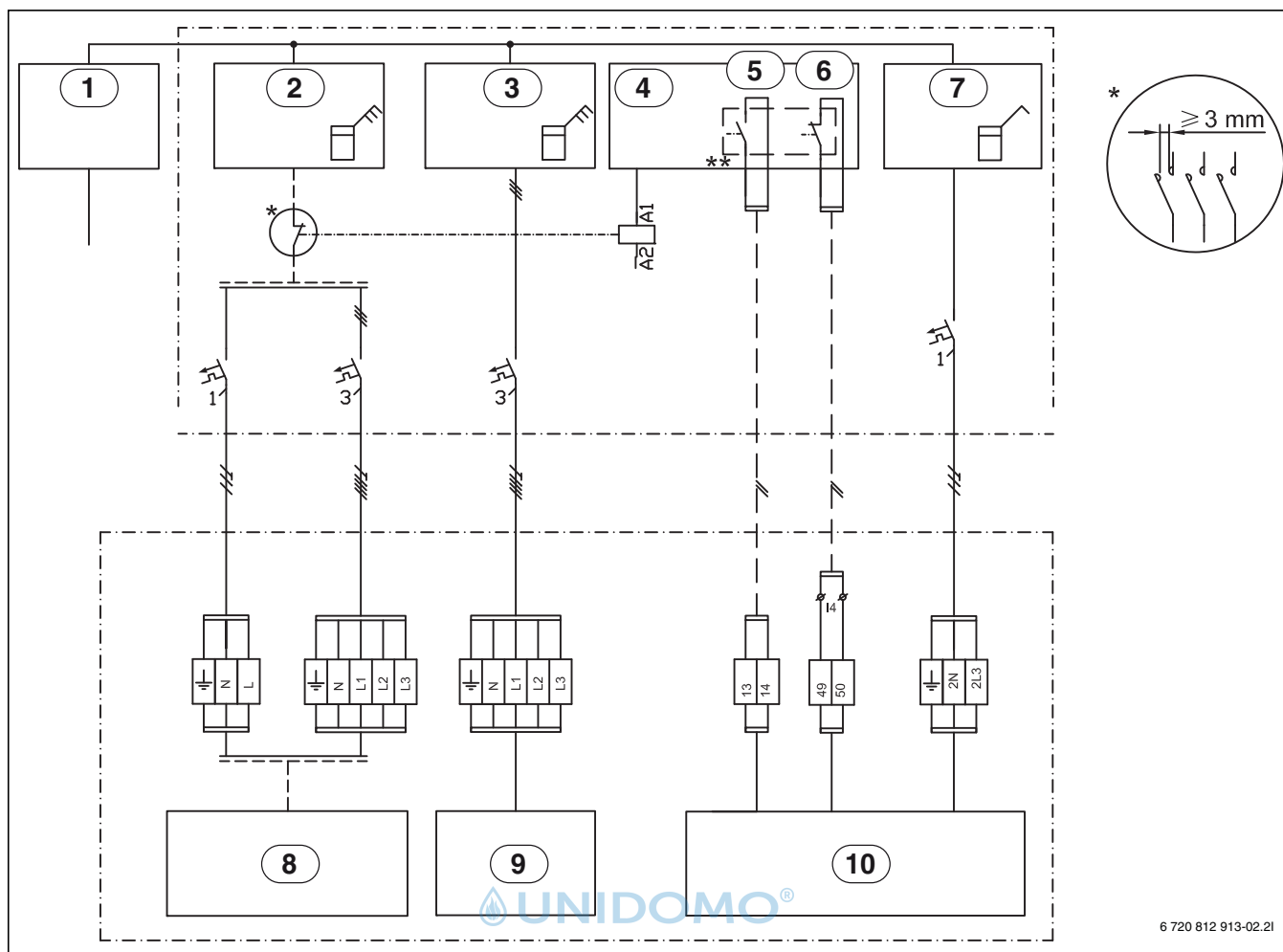
Bild 57 EVU Typ 2
