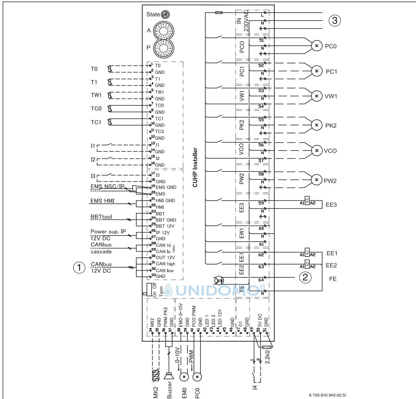
Bild 42 Schaltplan Installationsmodul
