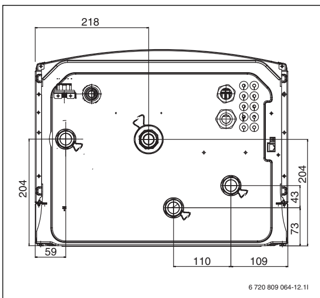
Bild 37 Inneneinheit mit elektrischem Zuheizer ACE, Abmessungen in mm (Ansicht von unten)
