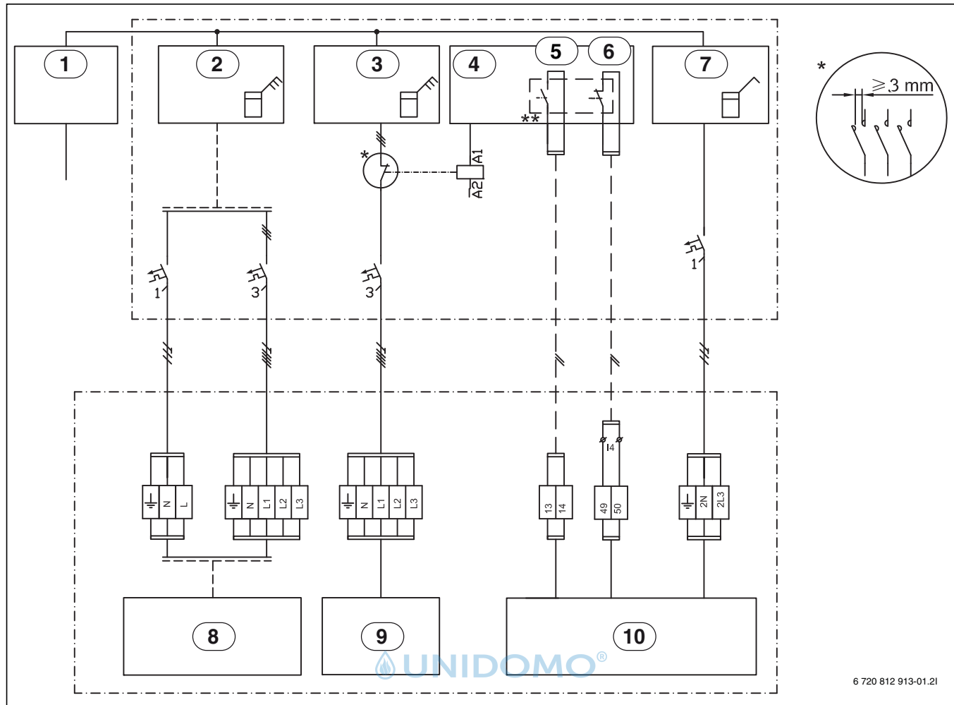
Bild 58 EVU Typ 3
