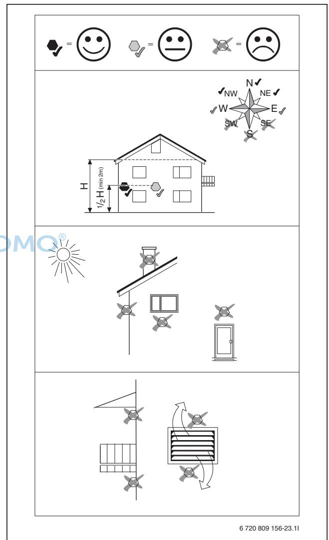
Bild 13 Anbringung von Außentemperaturfühlern
