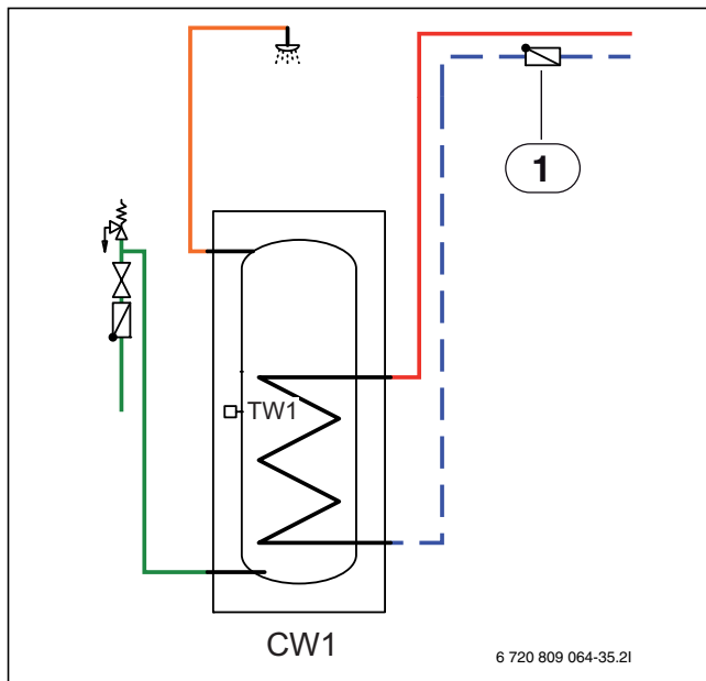
Bild 10 Heißwassererzeuger
