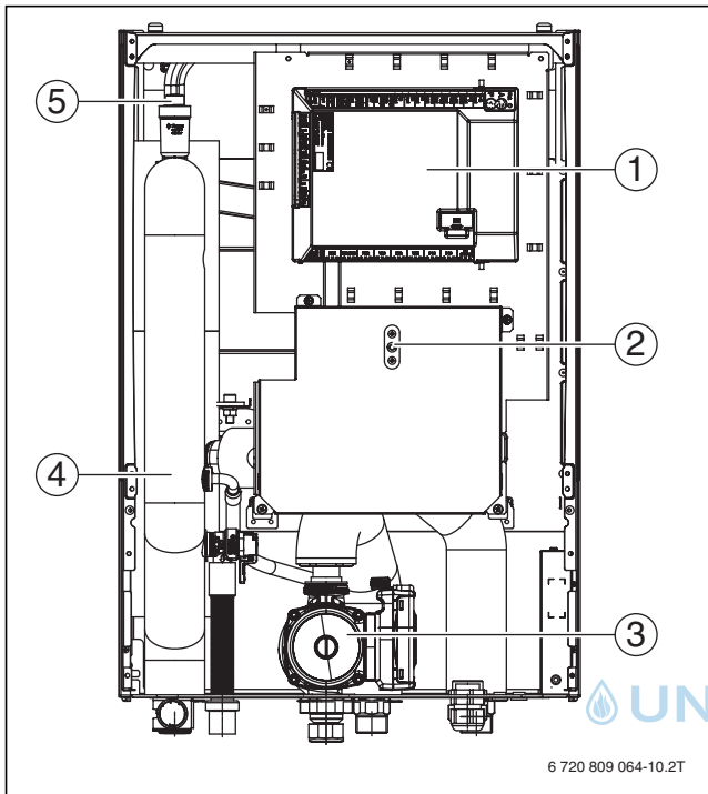
Bild 36 Inneneinheit mit elektrischem Zuheizer ACE
