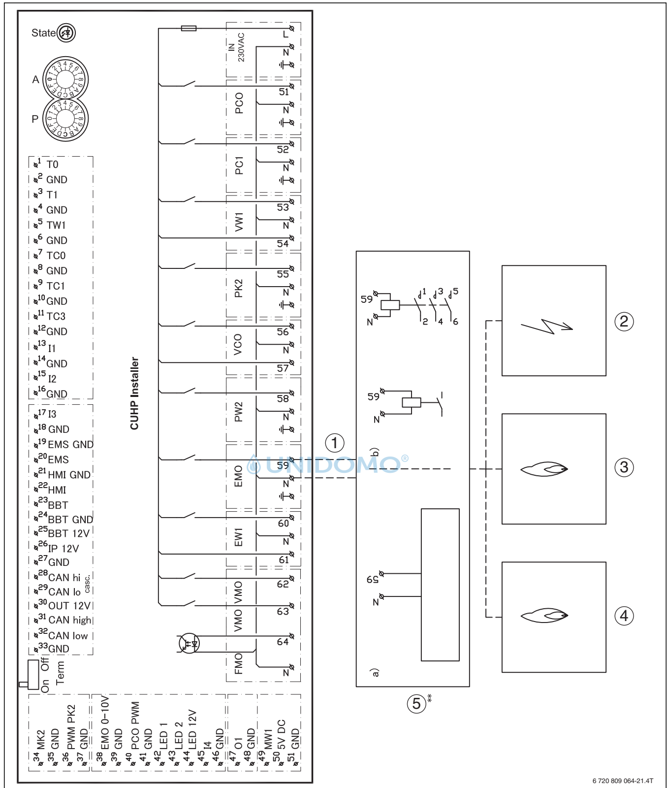
Bild 25 Schaltplan Installationsmodul, Start/Stop
