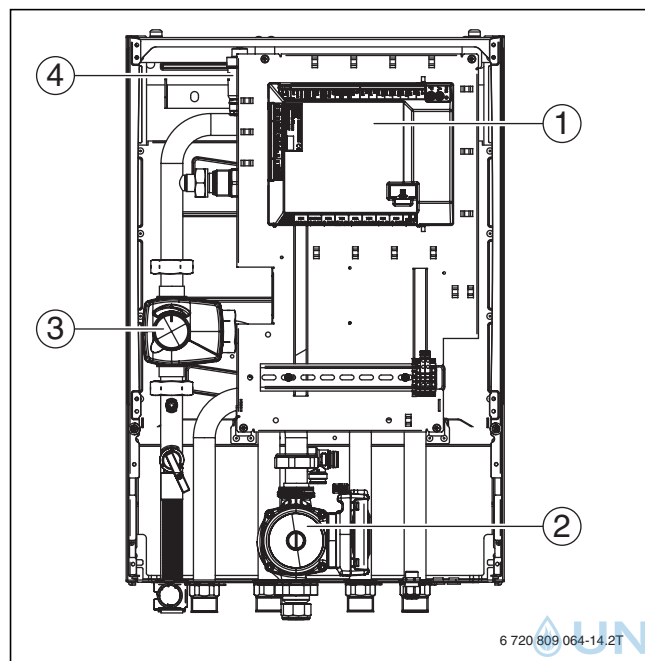
Bild 18 Innenmodul für den bivalenten Betrieb ACB
