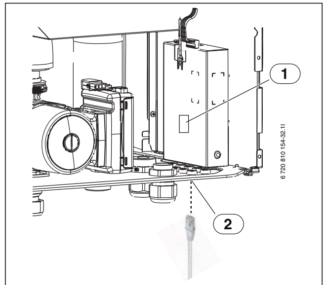
Bild 62 IP-Modul
