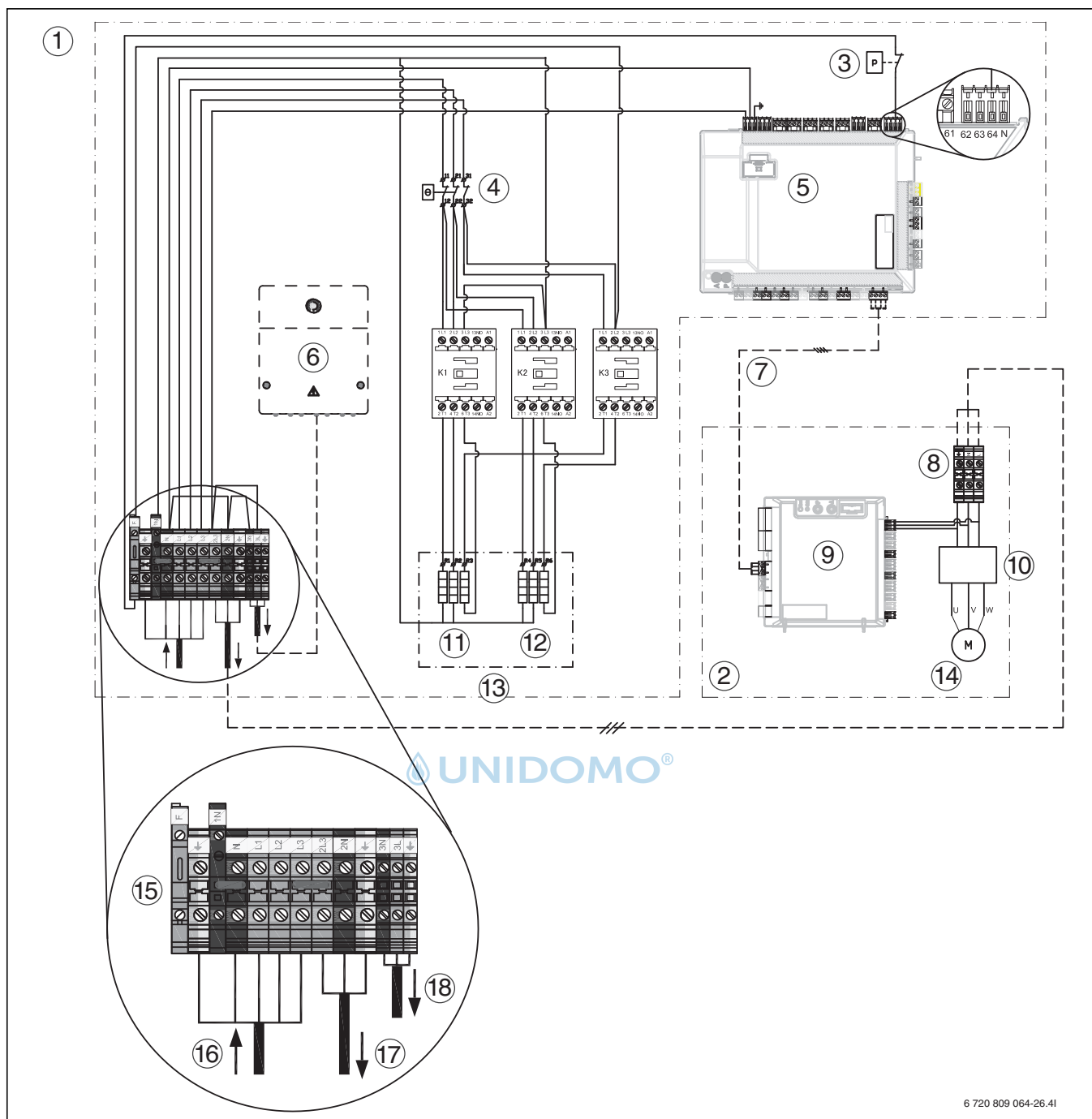
Bild 45 Einphasige Wärmepumpe und dreiphasiger integrierter elektrischer Zuheizer
