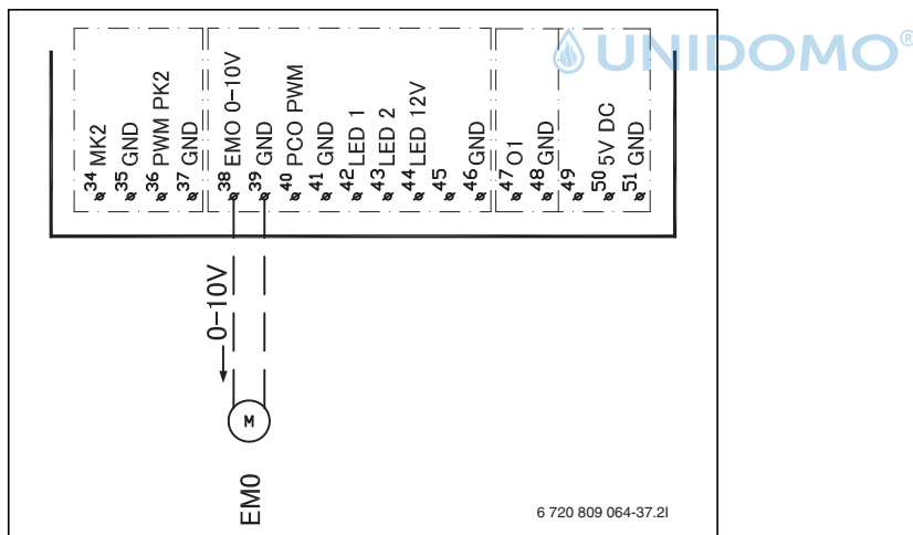
Bild 23 0- bis 10-V-Ansteuerung für Heizkessel
