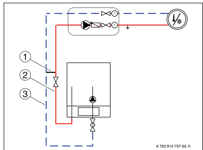
Bild 2 Inneneinheit mit Heizkreis und Bypass
