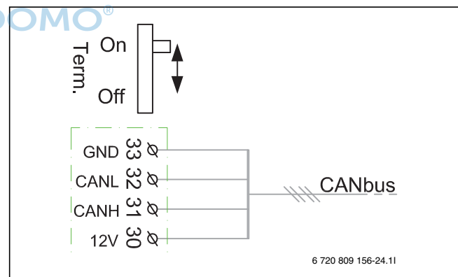
Bild 14 CAN-BUS-Terminierung
