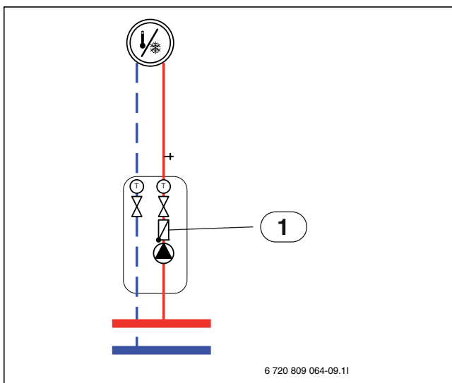
Bild 6 Heizkreis
