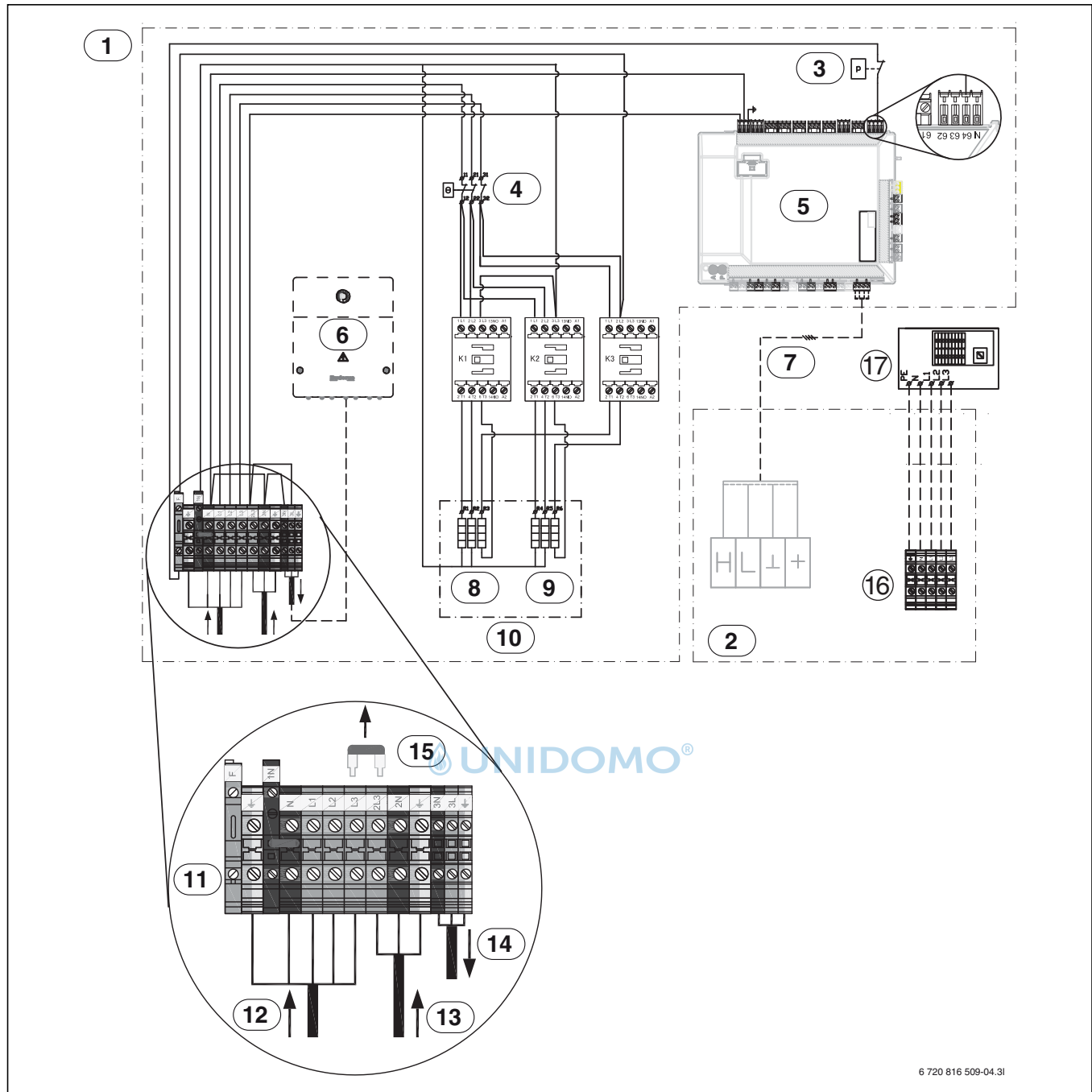
Bild 54 EVU, Wärmepumpe SAO-2 HT und integrierter elektrischer Zuheizer
