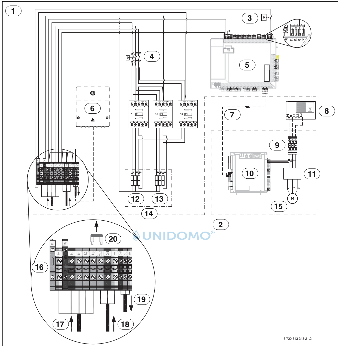
Bild 52 EVU, Einphasige Wärmepumpe und dreiphasiger integrierter elektrischer Zuheizer
