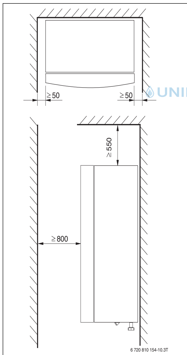
Bild 9 Mindestabstände
