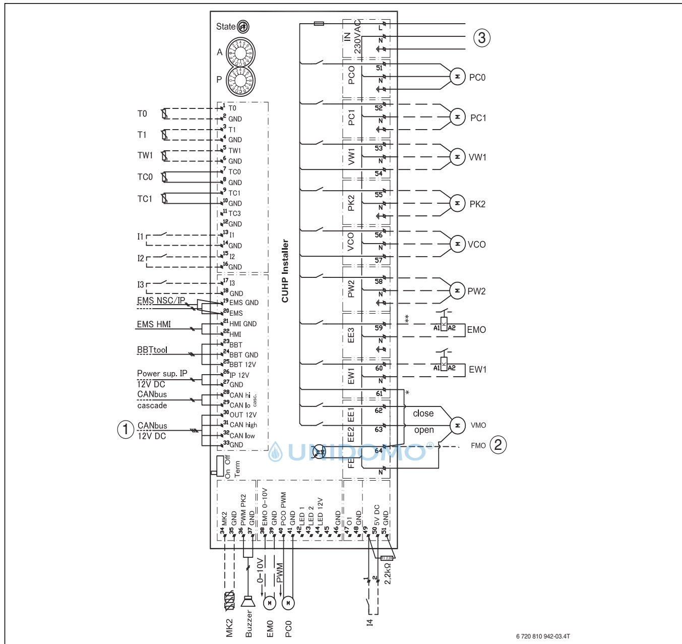
Bild 24 Schaltplan Installationsmodul
