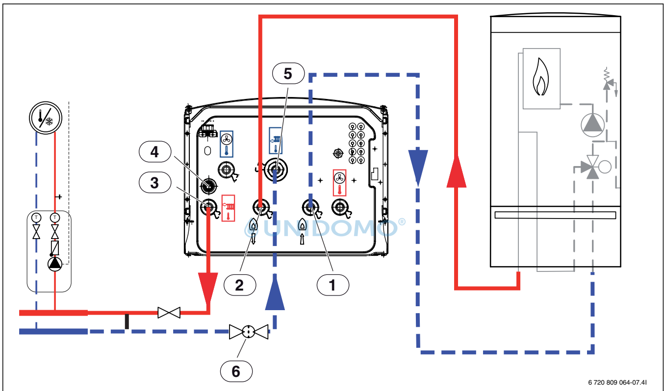
Bild 21 Anschluss der Inneneinheit für den bivalenten Betrieb ACB an die Heizungsanlage und den Zuheizer
