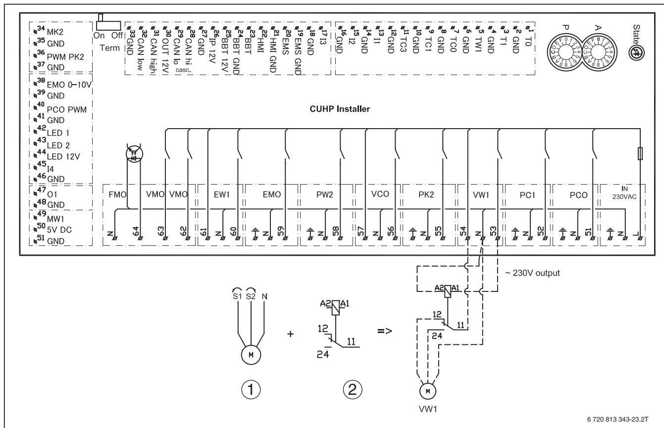
Bild 43 Alternative Installation 3-Wege-Ventil
