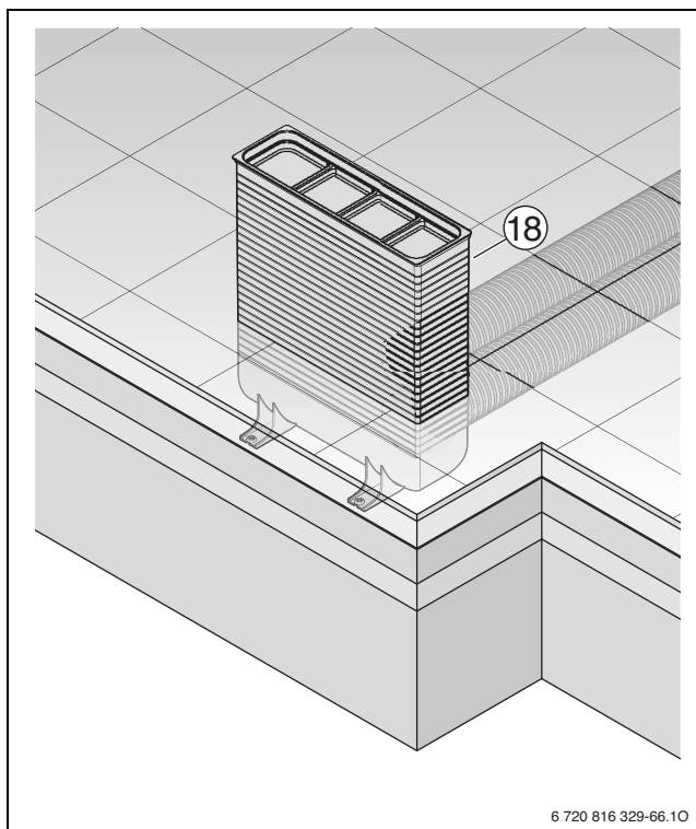
Fig. 87 RRU 75-2 + AG/...
