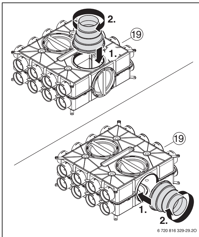
Fig. 47 VK 160
