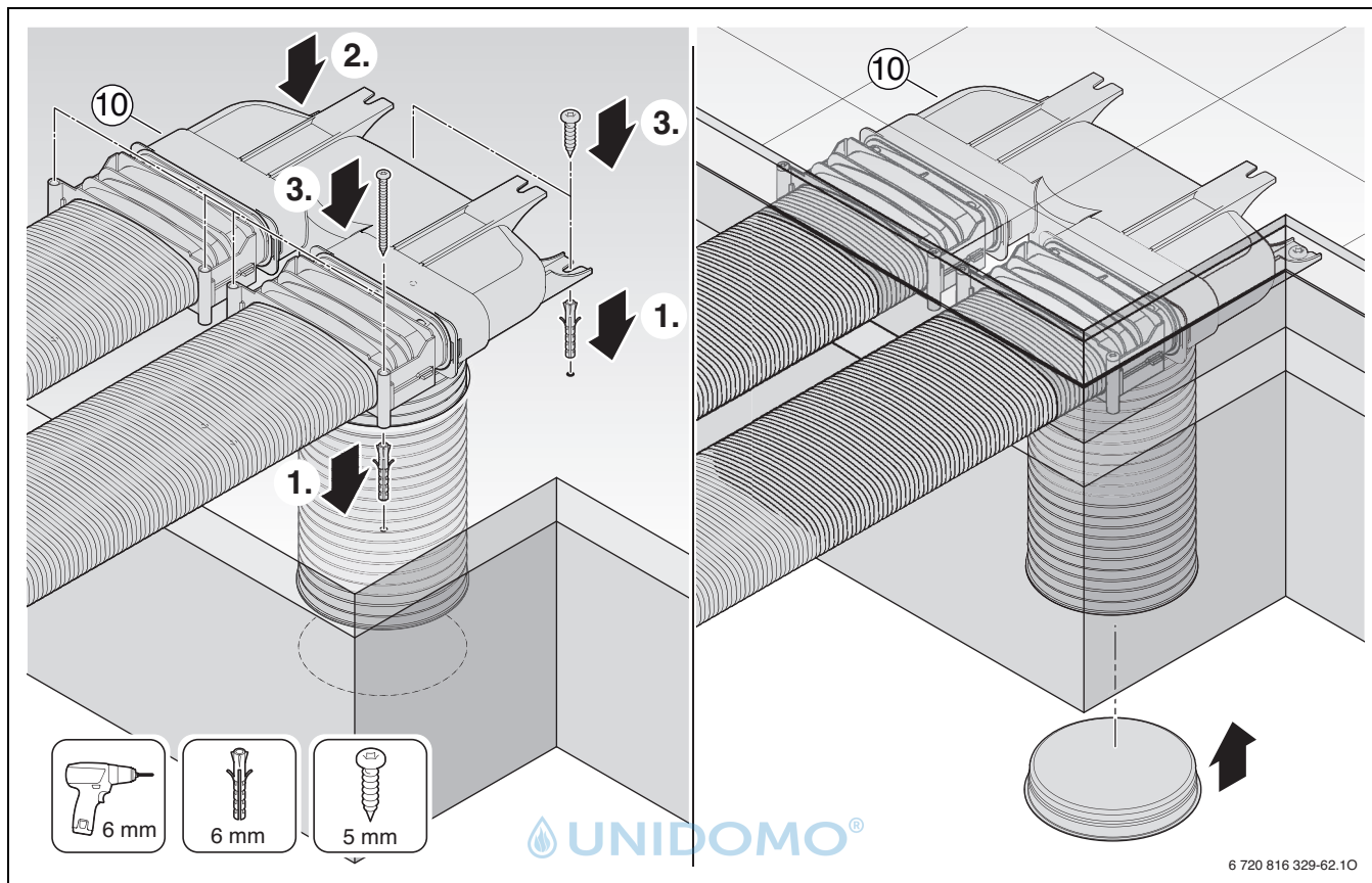
Fig. 69 FKU 140-3
