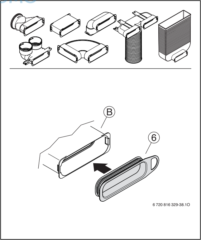
Fig. 75 FKS 140 + FKV.../FKB.../FKU.../RRB 75-3
