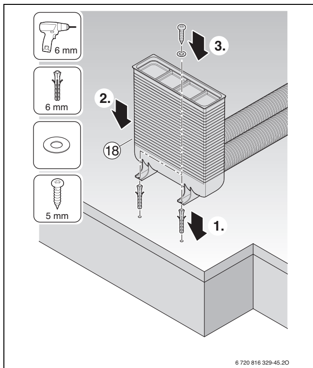
Fig. 86 RRU 75-2
