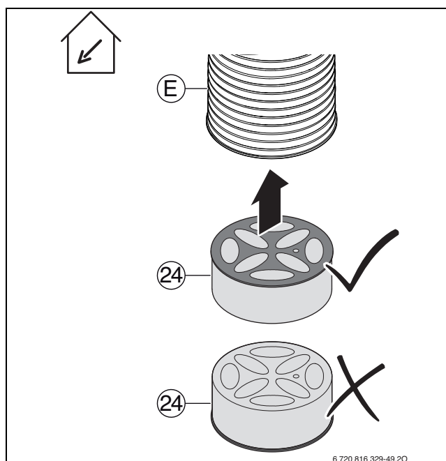
Fig. 71 FKU 140-3 + SDE
