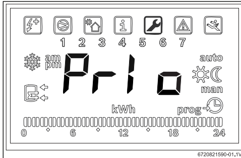
Bild 24 Untermenü "Prio"
