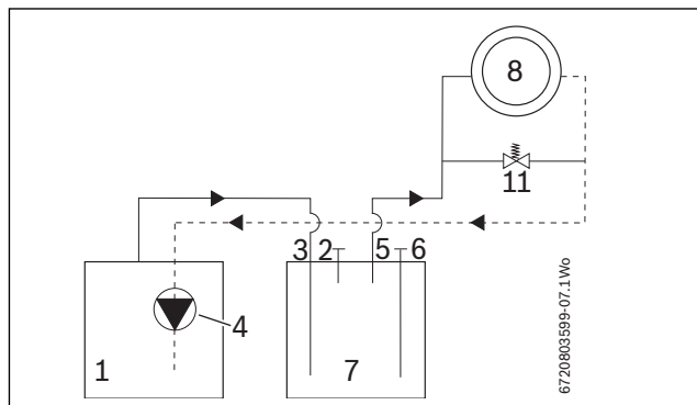
6. ábra Működési vázlat: a puffertároló soros csatlakoztatása a hőszivattyúra
