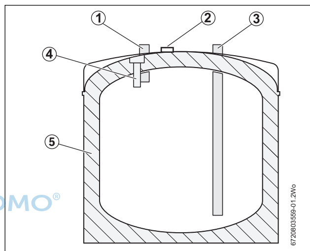
Afb. 1 Primair buffervat
