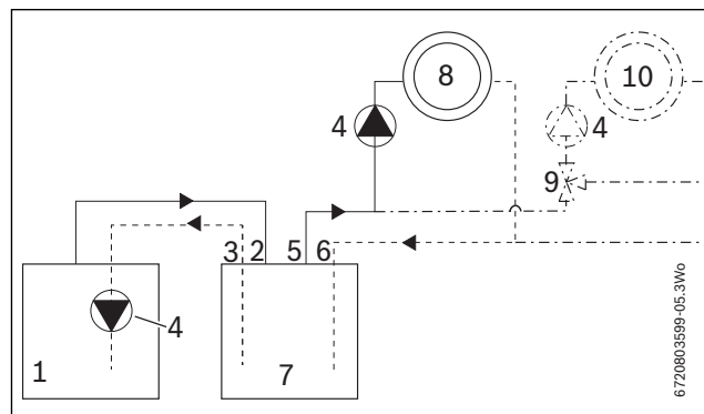
5. ábra Működési vázlat: a puffertároló párhuzamos csatlakoztatása a hőszivattyúra
