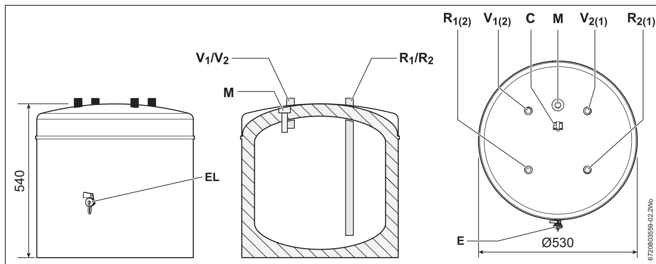
Fig. 2 Raccordements et dimensions (dimensions en mm)
