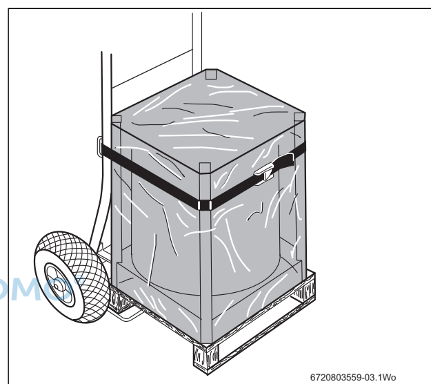
Sl.3 Transport međuspremnika tople vode kolicima za kotao
