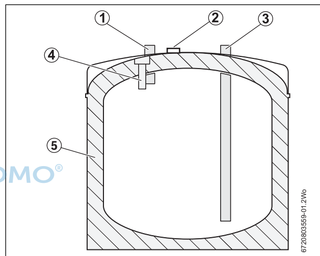
Fig. 1 Primær bufferbeholder
