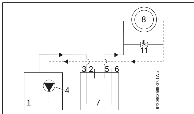
Joon. 6 Talitluskeem: Varumahuti jadaühendus soojuspumbaga
