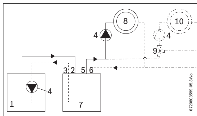
Fig. 5 Funktionsskema: Parallelt tilslutning af bufferbeholderen til varmepumpen
