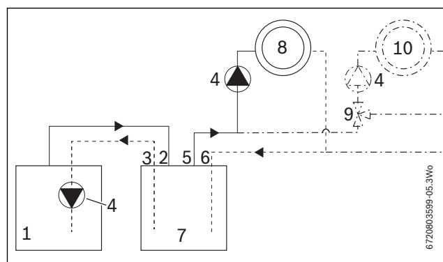
Fig. 5 Esquema de función: conexión paralela del acumulador a la bomba de calor
