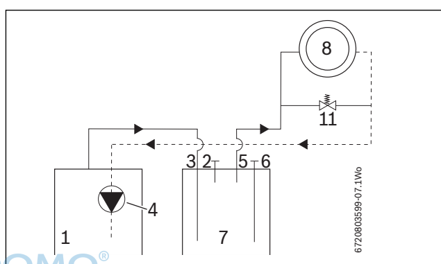
Fig. 6 Funktionsskema: Seriel tilslutning af bufferbeholderen til varmepumpen
