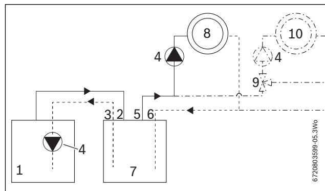
Joon. 5 Talitluskeem: Varumahuti rööpühendus soojuspumbaga
