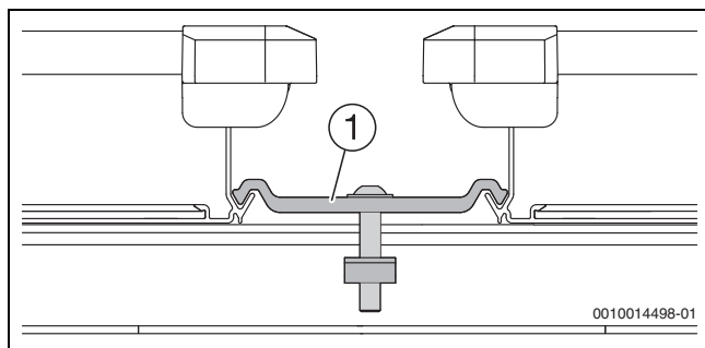
Bild 43 Doppelseitiger Kollektorspanner
