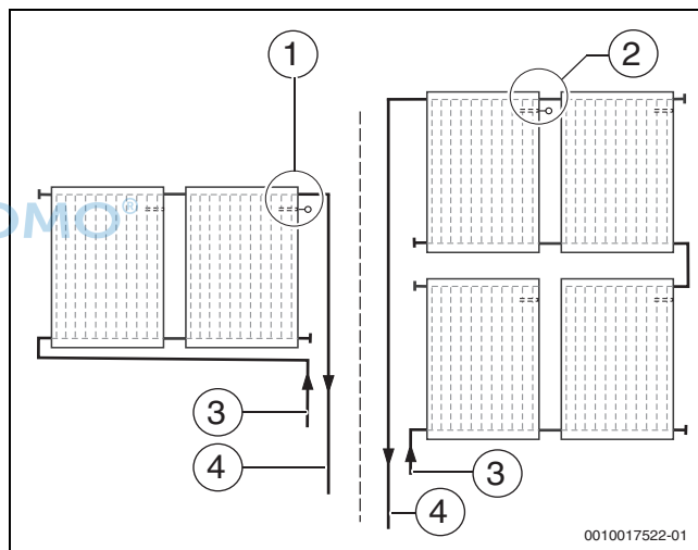
Bild 46 Position des Kollektortemperaturfühlers
