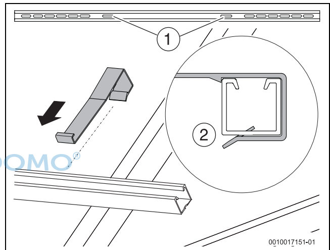
Bild 33 Abrutschsicherung an Profilschiene unten montieren
