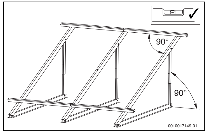
Bild 32 Profilschienen und Kollektorstützen ausrichten
