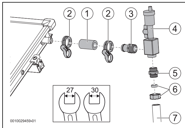
Bild 54 Vorlauf mit Entlüfter über Dach
