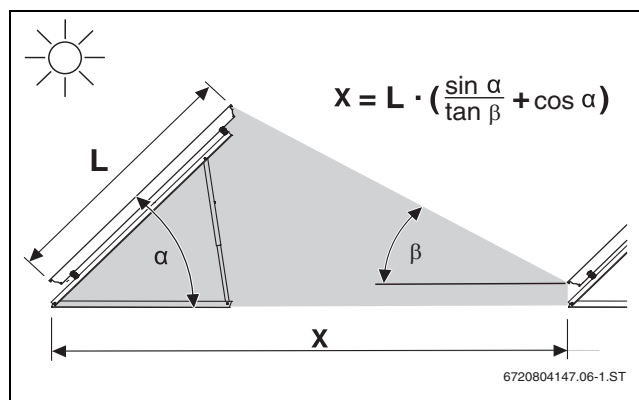
Bild 14 Abstand und Verschattung, Flachdachmontage
