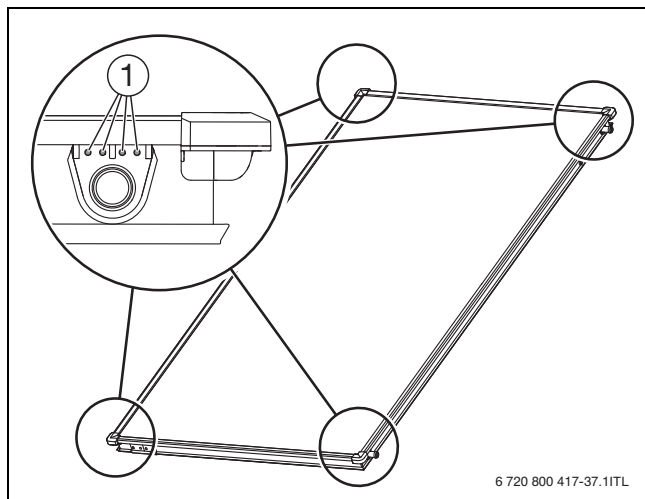
Bild 58 Belüftungsöffnungen
