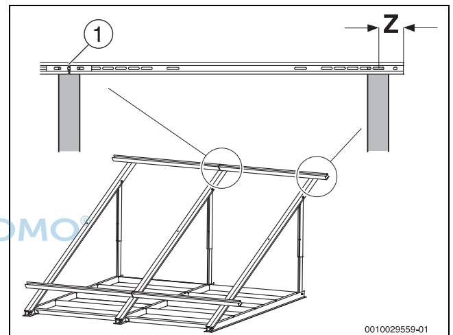
Bild 29 Profilschienen positionieren
