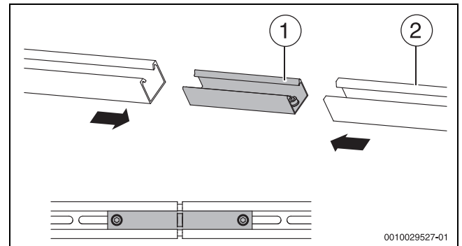
Bild 28 Profilschienen verbinden
