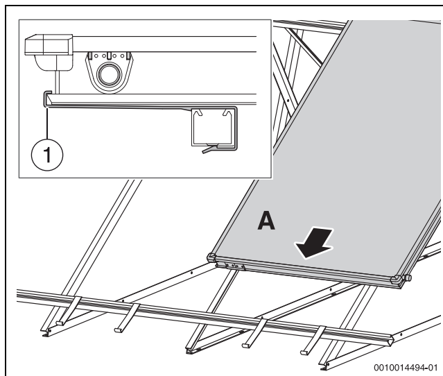
Bild 39 Kollektor in die Abrutschsicherungen gleiten lassen
