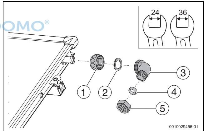
Bild 51 Winkeltülle montieren
