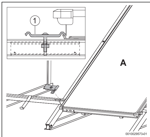
Bild 41 Doppelseitigen Kollektorspanner einlegen
