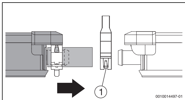
Bild 42 Linken Kollektor an den rechten Kollektor schieben
