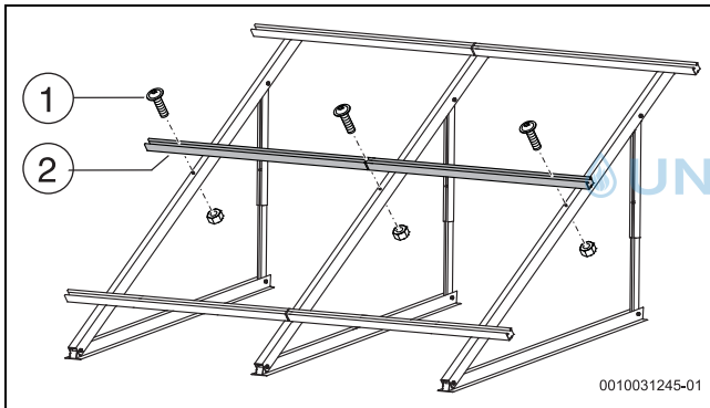
Bild 31 Zusätzliche Profilschienen montieren (hier: 2 Kollektoren)
