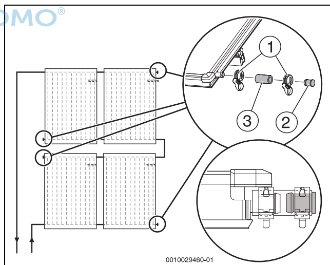
Bild 55 Zusätzlichen Solarschlauch montieren
