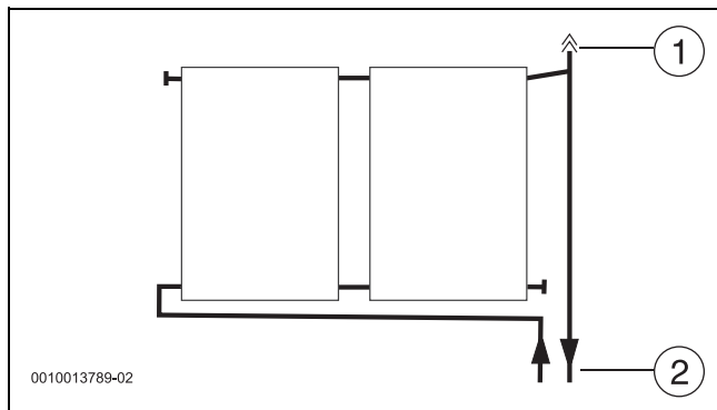
Bild 52 Hydraulischer Anschluss mit Entlüfter (Vorlauf rechts)
