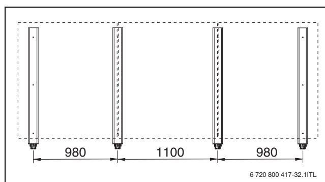
Bild 20 3 Kollektoren (Maße in mm)
