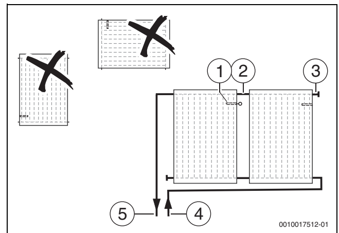
Bild 10 Kollektoren anordnen
