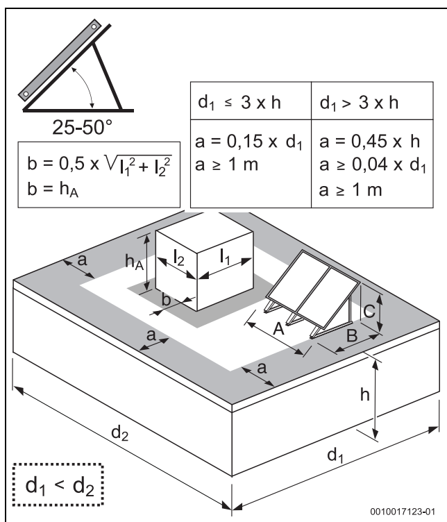
Bild 15 Bei Maß a ist der größere Wert maßgebend; bei [b] ist der kleinere Wert maßgebend (Anstellwinkel Kollektoren 25°-50°)
