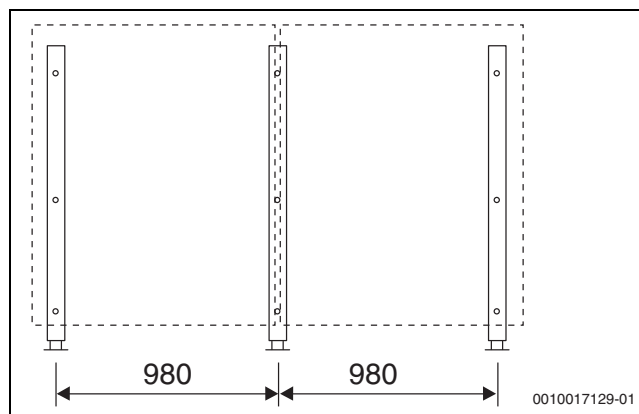
Bild 19 2 Kollektoren (Maße in mm)
