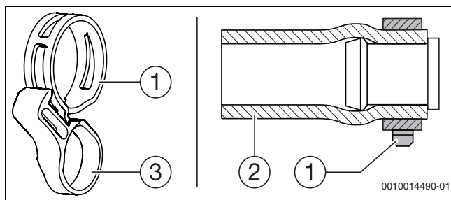
Bild 34 Sicherung von Solarschläuchen (hier: mit Stopfen)
