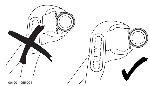
Bild 35 Federbandschelle ohne Sicherungsring versetzen
