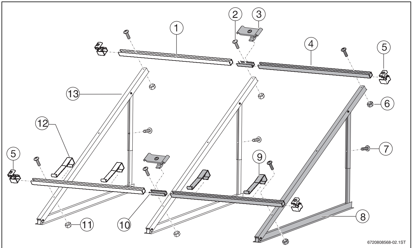
Bild 3 Montage-Set für 2 Kollektoren: 1 Montage-Set Grundaussführung, 1 Montage-Set Erweiterung (grau)
