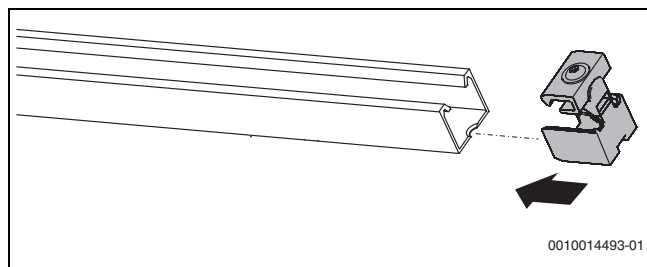
Bild 38 Kollektorspanner rechts montieren
