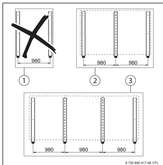
Bild 23 Feldweise Anordnung der Kollektoren
