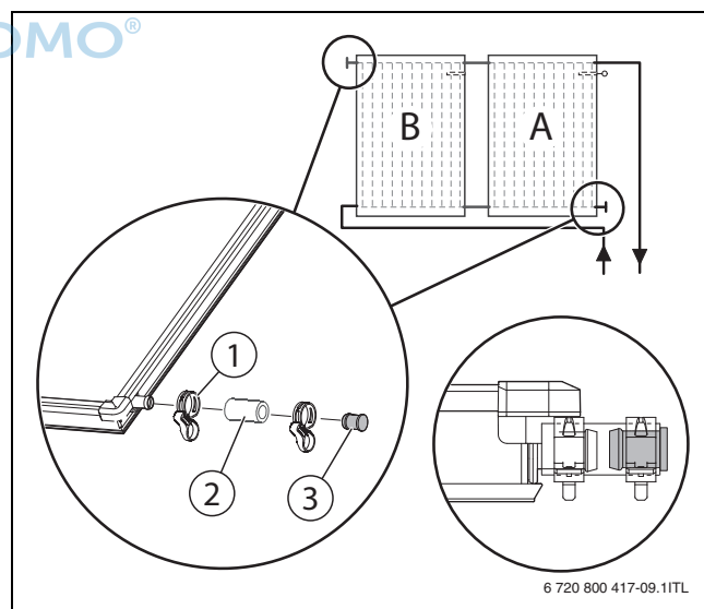
Bild 36 Stopfen montieren
