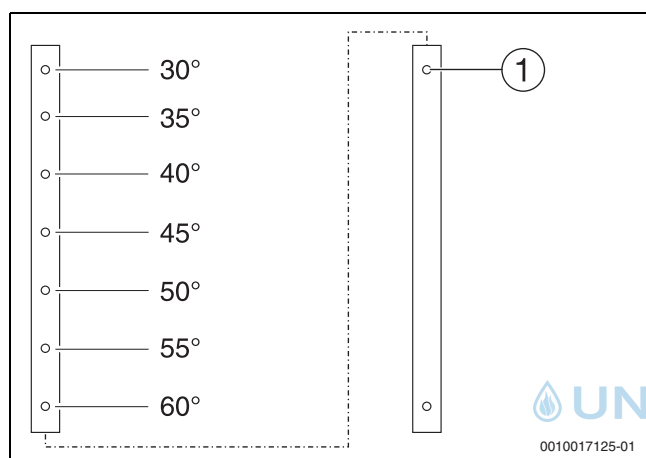
Bild 17 Teleskopschienen montieren
