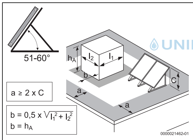
Bild 16 Bei Maß a ist der größere Wert maßgebend; bei [b] ist der kleinere Wert maßgebend (Anstellwinkel Kollektoren 51°-60°)
