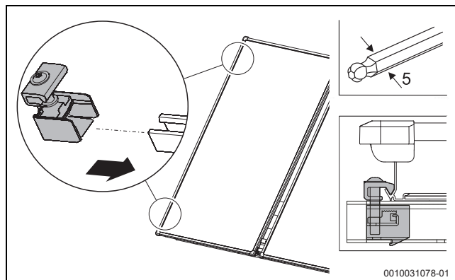
Bild 45 Kollektorspanner links montieren
