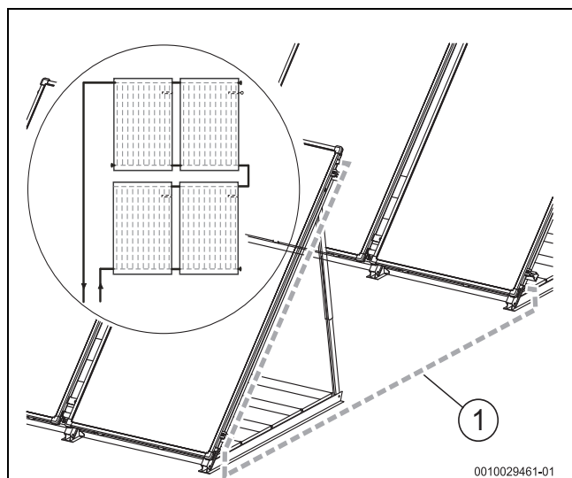
Bild 56 Bauseitige Rohrleitung montieren
