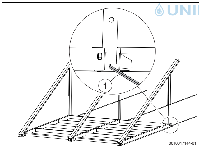
Bild 27 Kollektorstützen mit Seilsicherung
