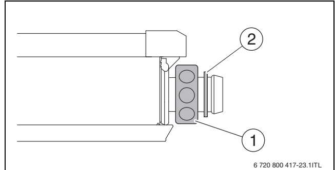
Bild 50 Anschluss der Rohrleitung vorbereiten
