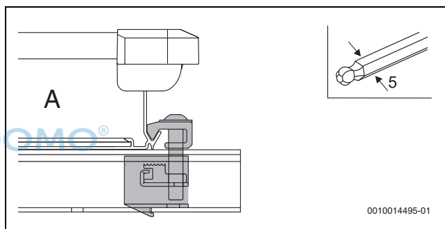
Bild 40 Kollektorspanner festdrehen
