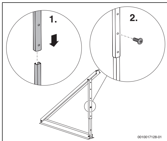
Bild 18 Teleskopschienen montieren
