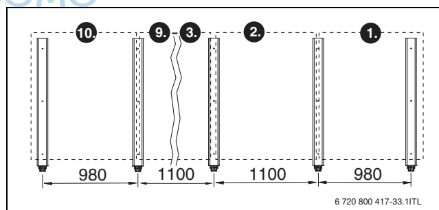
Bild 21 &gt; 3 senkrechte Kollektoren (Maße in mm)
