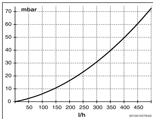
Bild 2 Druckverlustkurve (Wasser-Glykol-Gemisch)
