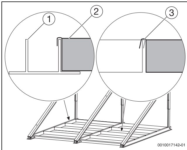
Bild 26 Kollektorstützen mit Beschwerungswannen für 2 Kollektoren
