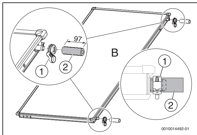
Bild 37 Verbindungs-Set am zweiten Kollektor und alle weiteren montieren
