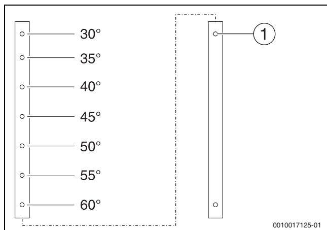
Bild 22 Teleskopschienen montieren
