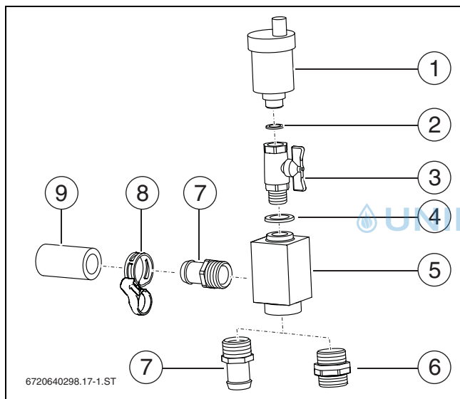
Bild 53 Lieferumfang Entlüfter-Set (Zubehör)
