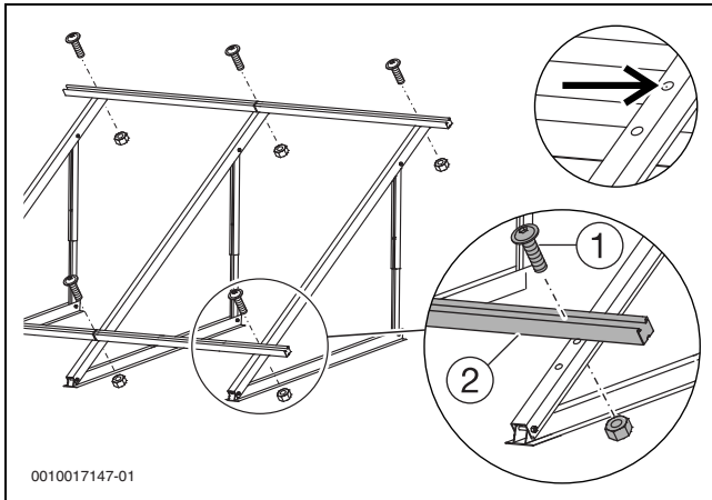
Bild 30 Profilschienen montieren
