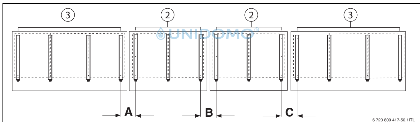
Bild 24 Beispiel 10 Kollektoren mit Beschwerungswannen: Feldkombination 3 + 2 + 2 + 3
