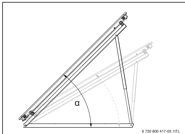
Bild 12 Anstellwinkel der Kollektoren
