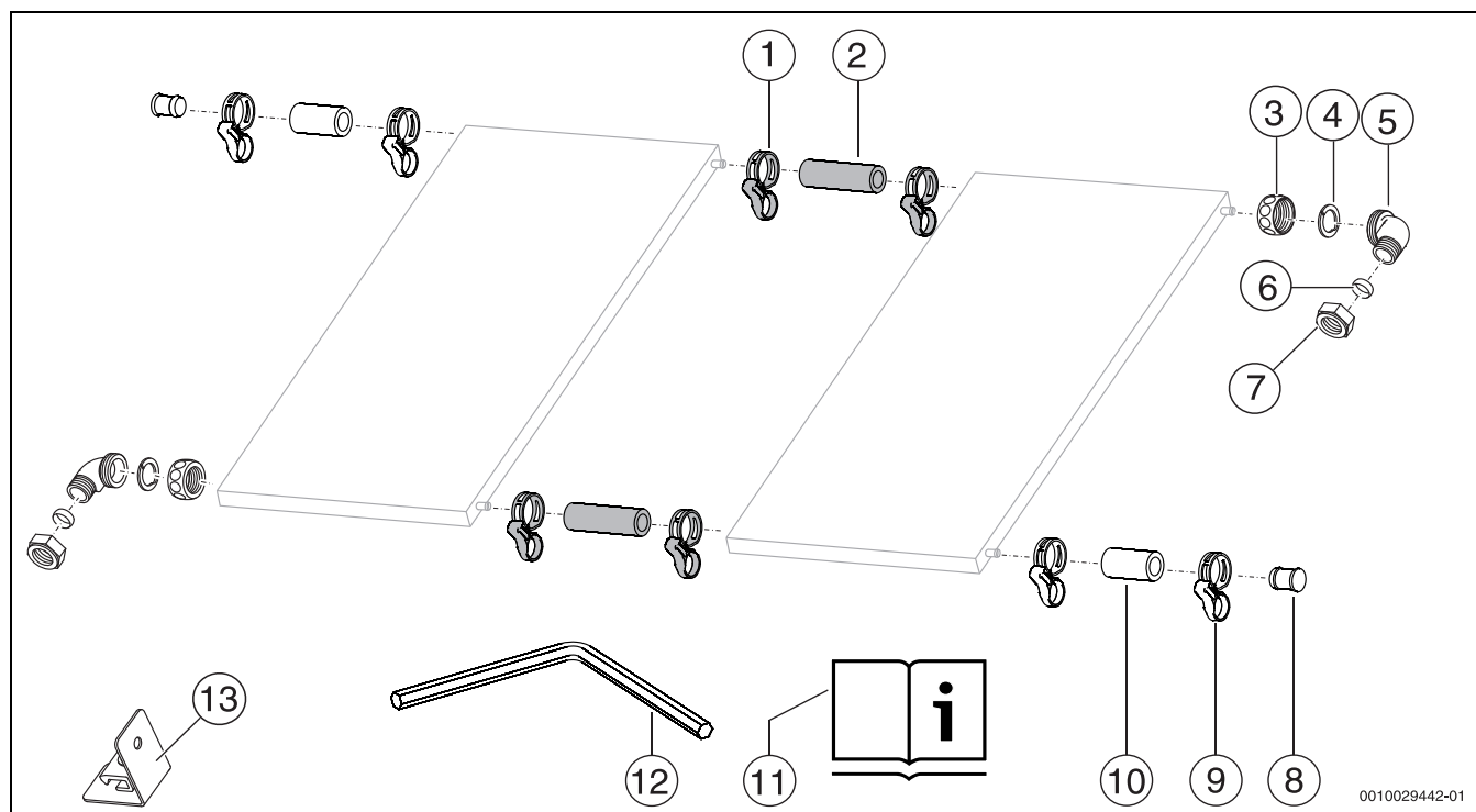
Bild 4 1 Anschluss-Set Flachdach und 2 Verbindungs-Sets (grau)
