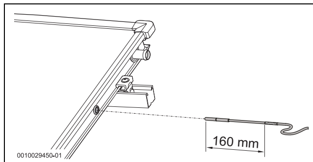
Bild 47 Kollektortemperaturfühler montieren
