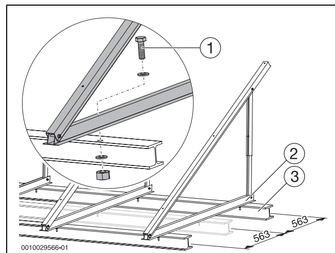
Bild 25 Kollektorstützen auf Doppel-T-Träger, Maße in mm
