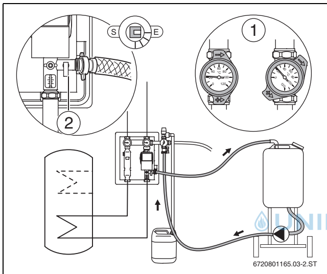
Bild 32 Spülen des Standardsystems
