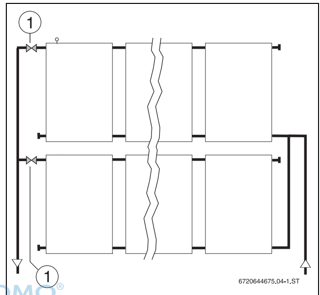
Bild 28 Spülen von parallel geschalteten Kollektorfeldern
