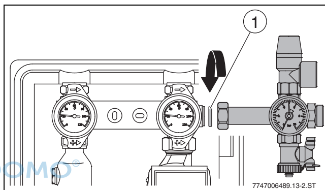
Bild 17 Sicherheitsgruppe montieren
