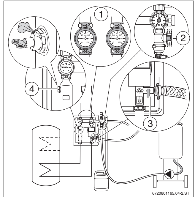
Bild 33 Füll- und Entleerhähne schließen und öffnen
