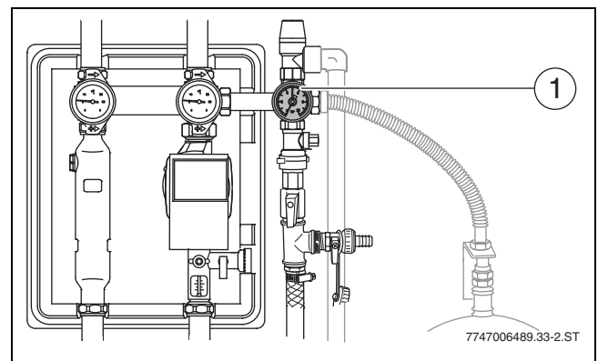
Bild 34 Manometeranzeige prüfen
