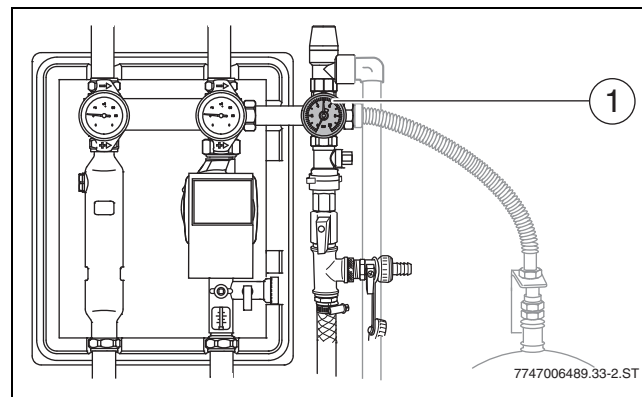
Bild 40 Manometeranzeige prüfen
