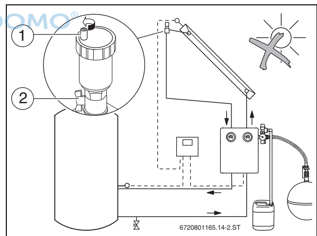
Bild 37 Entlüfter öffnen
