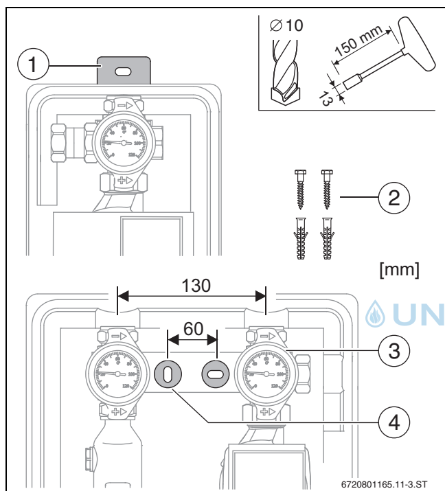
Bild 16 Montage der Station
