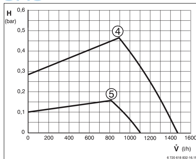
Bild 84 Proportionaldruck
