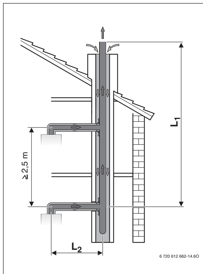
Bild 20 Mehrfachbelegung mit konzentrischem Rohr nach C 43x
