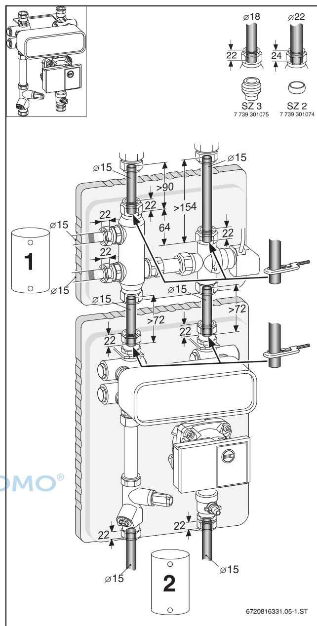
Fig. 5 SBT + SBU
