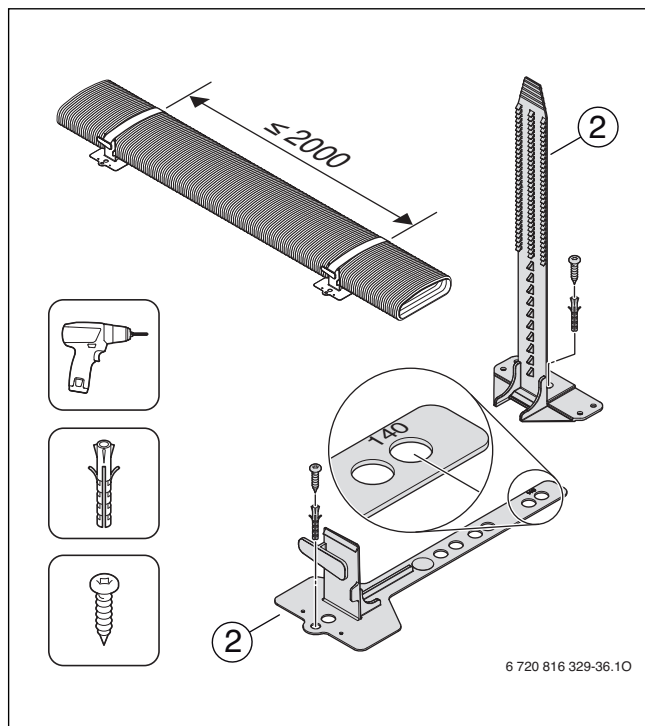
Fig. 37 FKH 140
