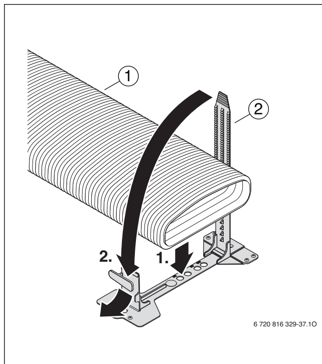
Fig. 38 FK 140 + FKH
