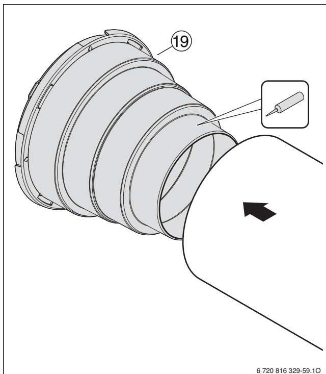
Fig. 29 VK 160
