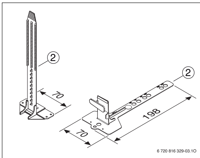
Fig. 22 FKH 140
