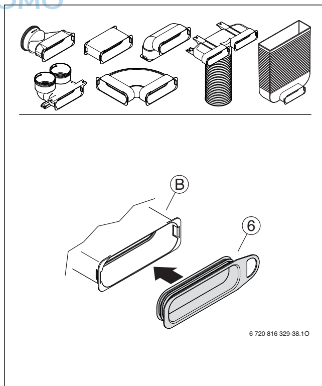
Fig. 47 FKS 140 + FKV.../FKB.../FKU.../RRB 75
