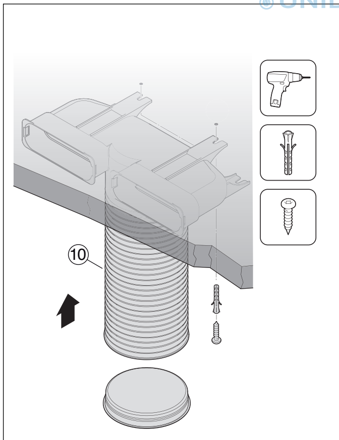
Fig. 43 FKU 140-1
