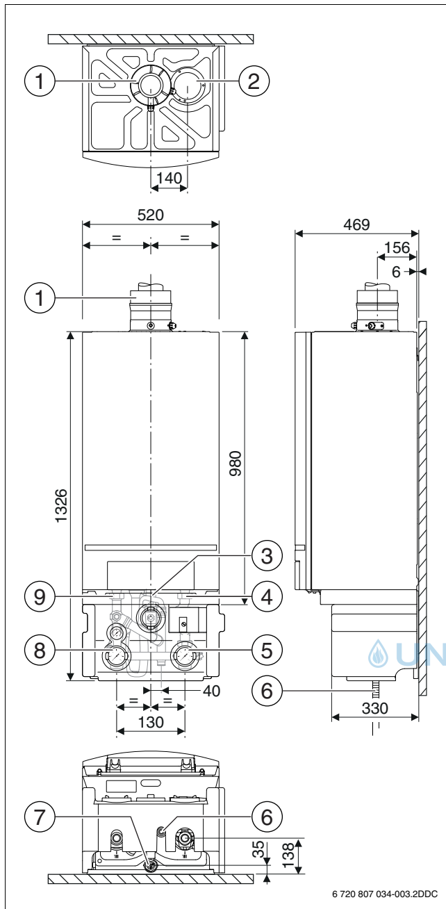
Bild 3 Abmessungen [mm]
