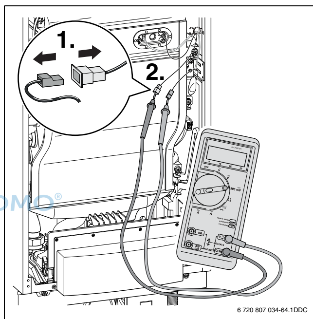
Bild 48 Anschluss des Multimeters
