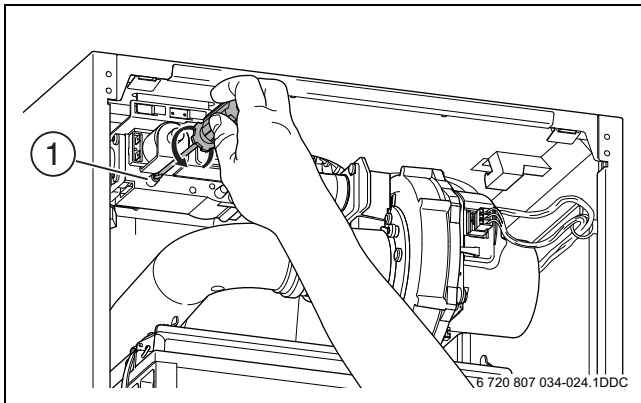
Bild 42 Öffnen des Brennerdrucknippels am Typ 100
