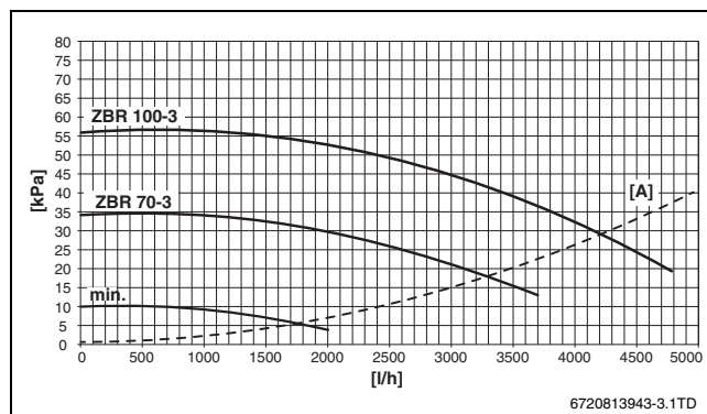
Bild 8 Restförderhöhe pro Typ, mit Anschluss-Set
