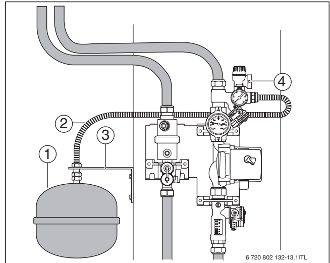
Bild 16 Ausdehnungsgefäß montieren
