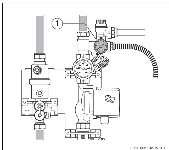
Bild 24 Manometeranzeige prüfen
