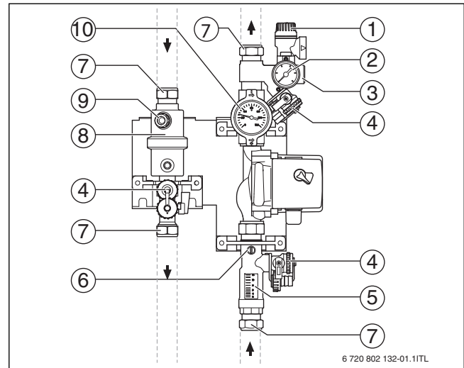
Bild 3 Solarstation ohne Isolierhaube und ohne integrierten Regler und Module
