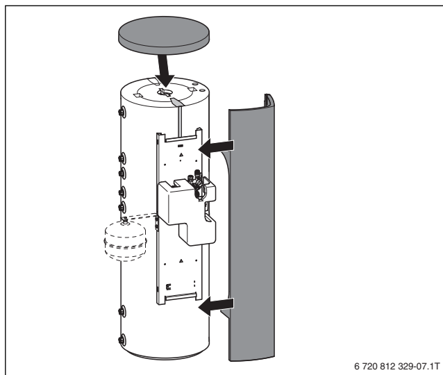
Bild 28 Verkleidung montieren und Deckel aufsetzen
