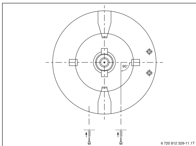
Bild 14 PVC-Verkleidungsmantel
