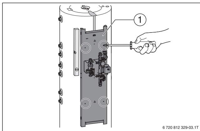
Bild 12 Montageplatte ausrichten
