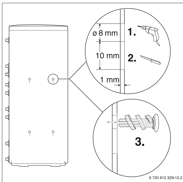
Bild 13 PS-Mantel vorbereiten
