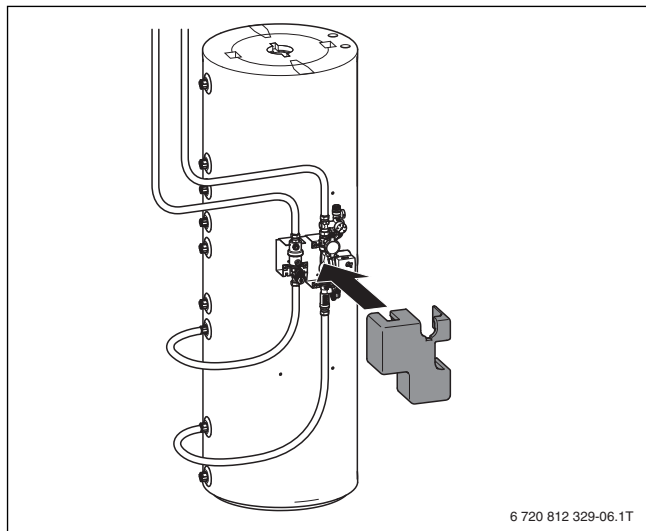
Bild 27 Isolierhaube aufsetzen
