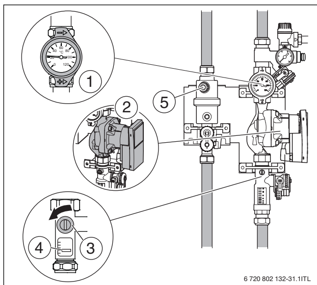
Bild 26 Solaranlage entlüften
