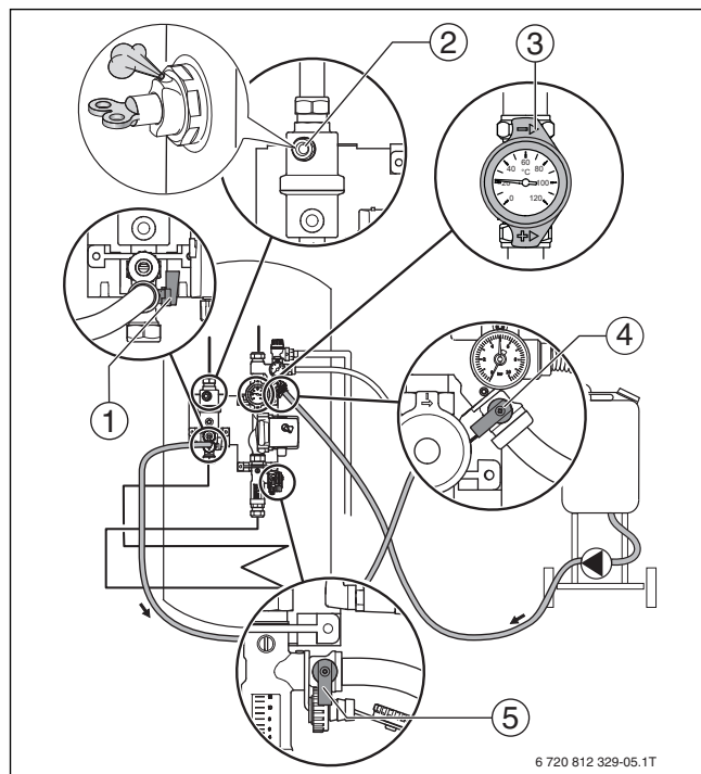
Bild 23 Füll- und Entleerhähne schließen und öffnen
