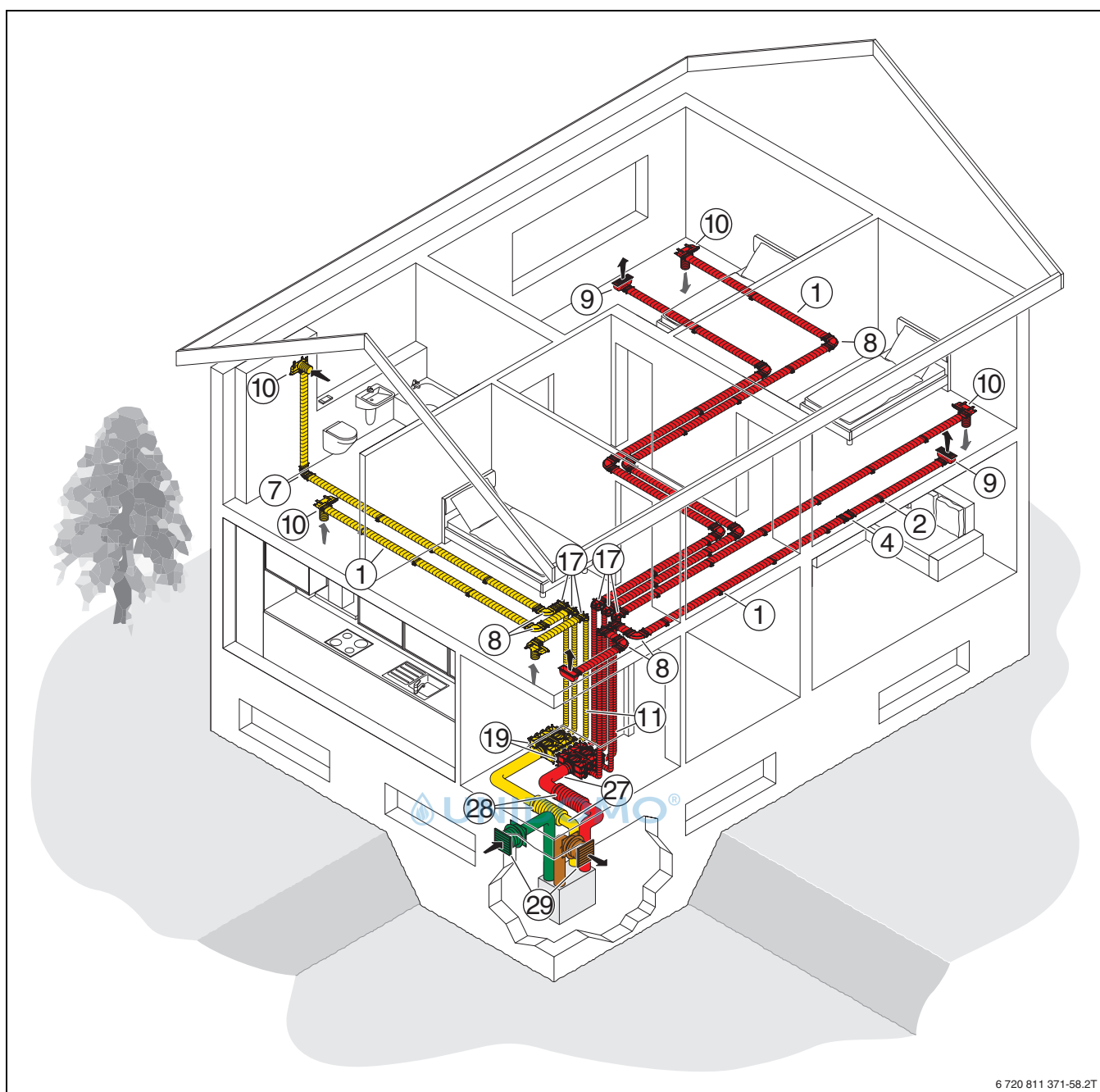
Bild 20 Anlagenbeispiel mit Zubehörten
