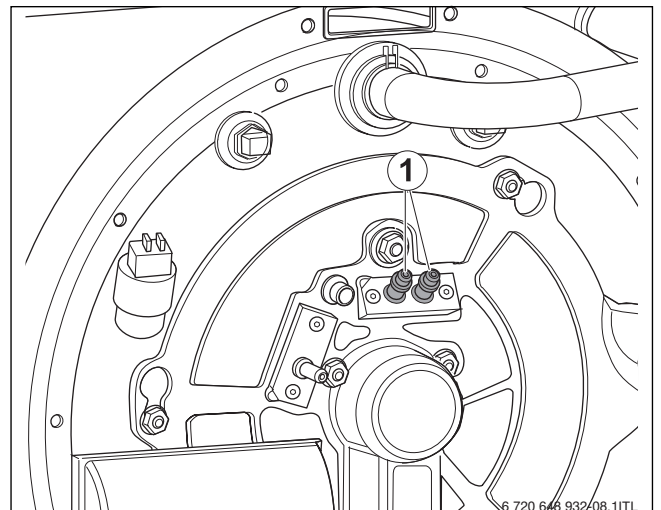
Fig. 5 Elettrodo accensione
