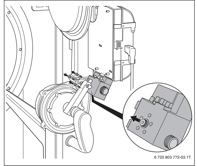
12. ábra Cserélje ki a gázfúvókát
