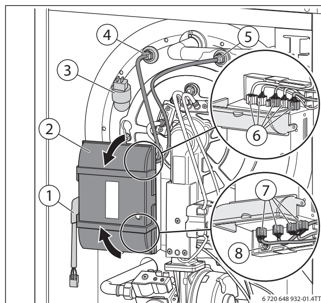
Fig. 3 Soltar os conectores
