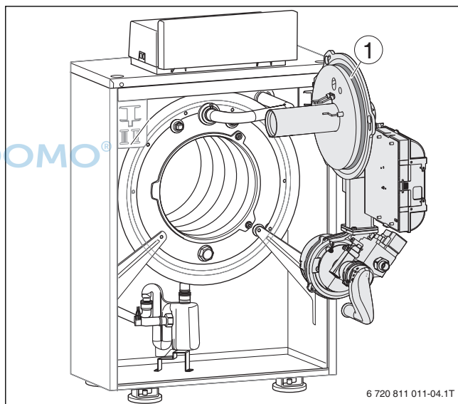
Afb. 13 O-ring branderhuis
