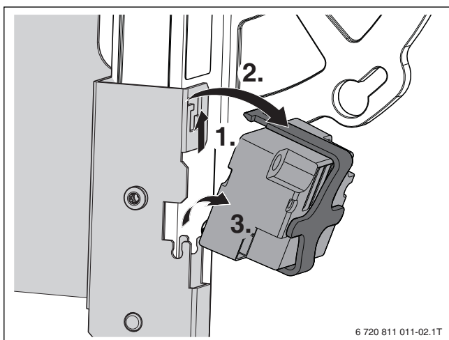
Afb. 6 Ontstekingstrafo verwijderen
