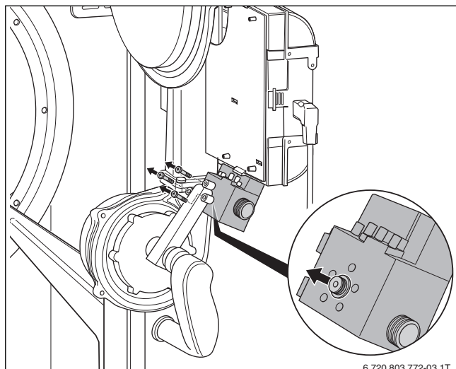
Bild 12 Gasdüse austauschen
