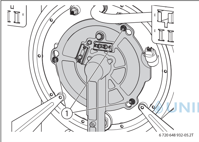
10. ábra Rögzítőanyák oldása
