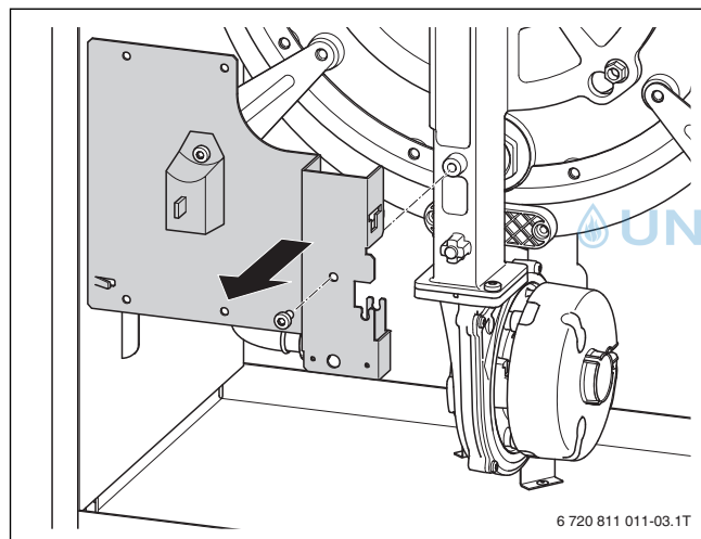
Fig. 7 Smontare la lamiera di fissaggio.
