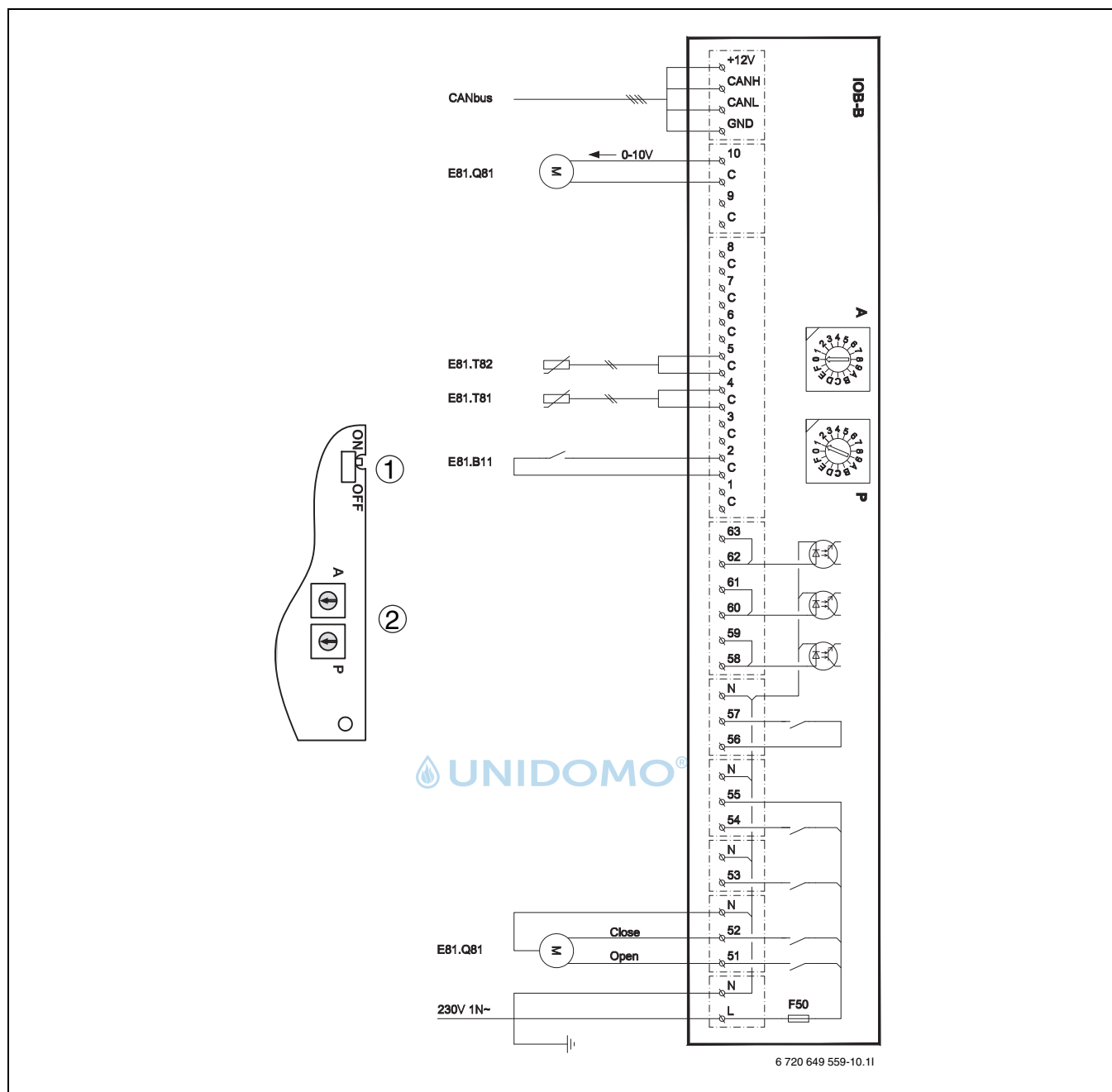
Bild 13 Schaltplan Schwimmbadsteuerung
