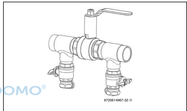
Bild 22 Befüll-einrichtung in Normalposition
