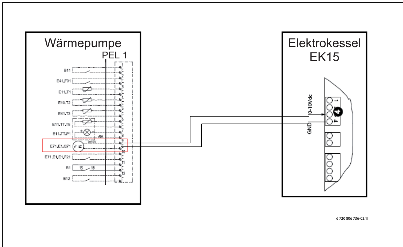
Bild 40 Anschluss der Wärmepumpe zum externen Elektroheizer EK15
