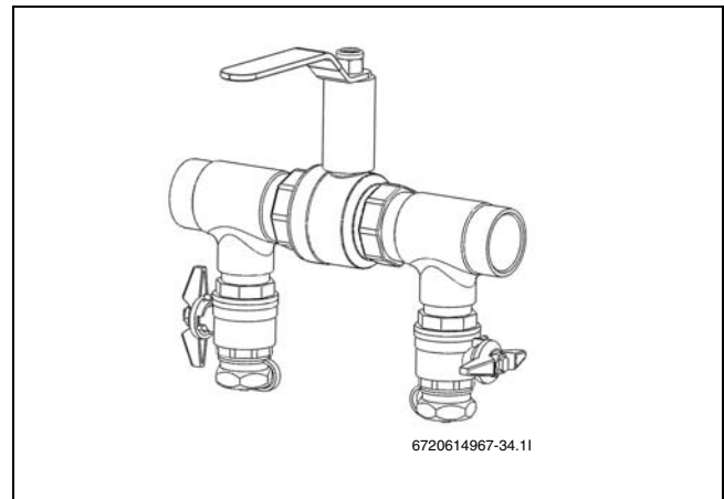
Bild 21 Befüll-einrichtung in Druckerhöhungsposition
