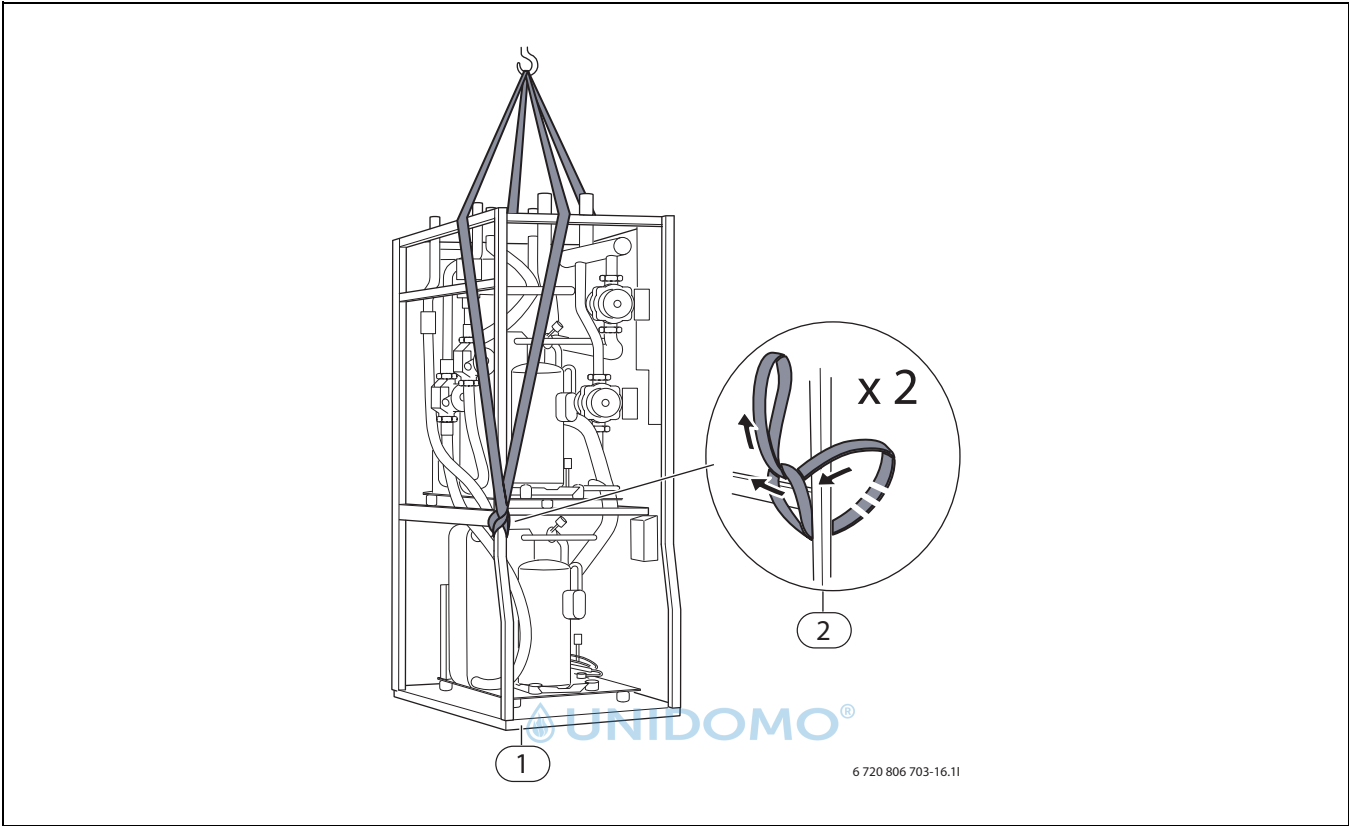
Bild 3 T 330-2 mit Hebeschlinge
