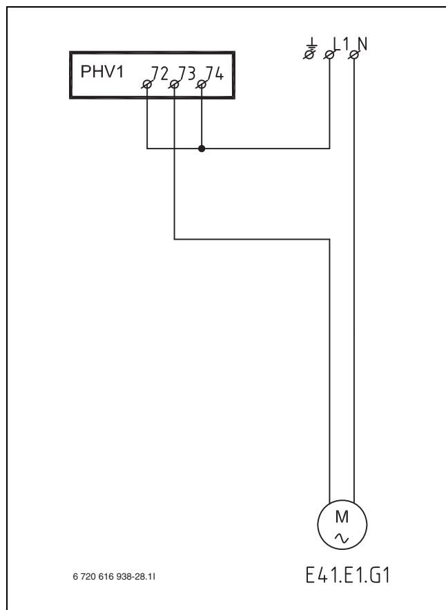
Bild 44 Anschluss der Umwälzpumpe E41.E1.G1
