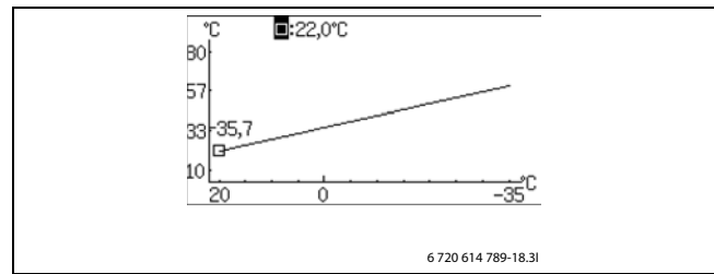
Bild 50 Einstellungsanzeige Heizkurve (Heizung)
