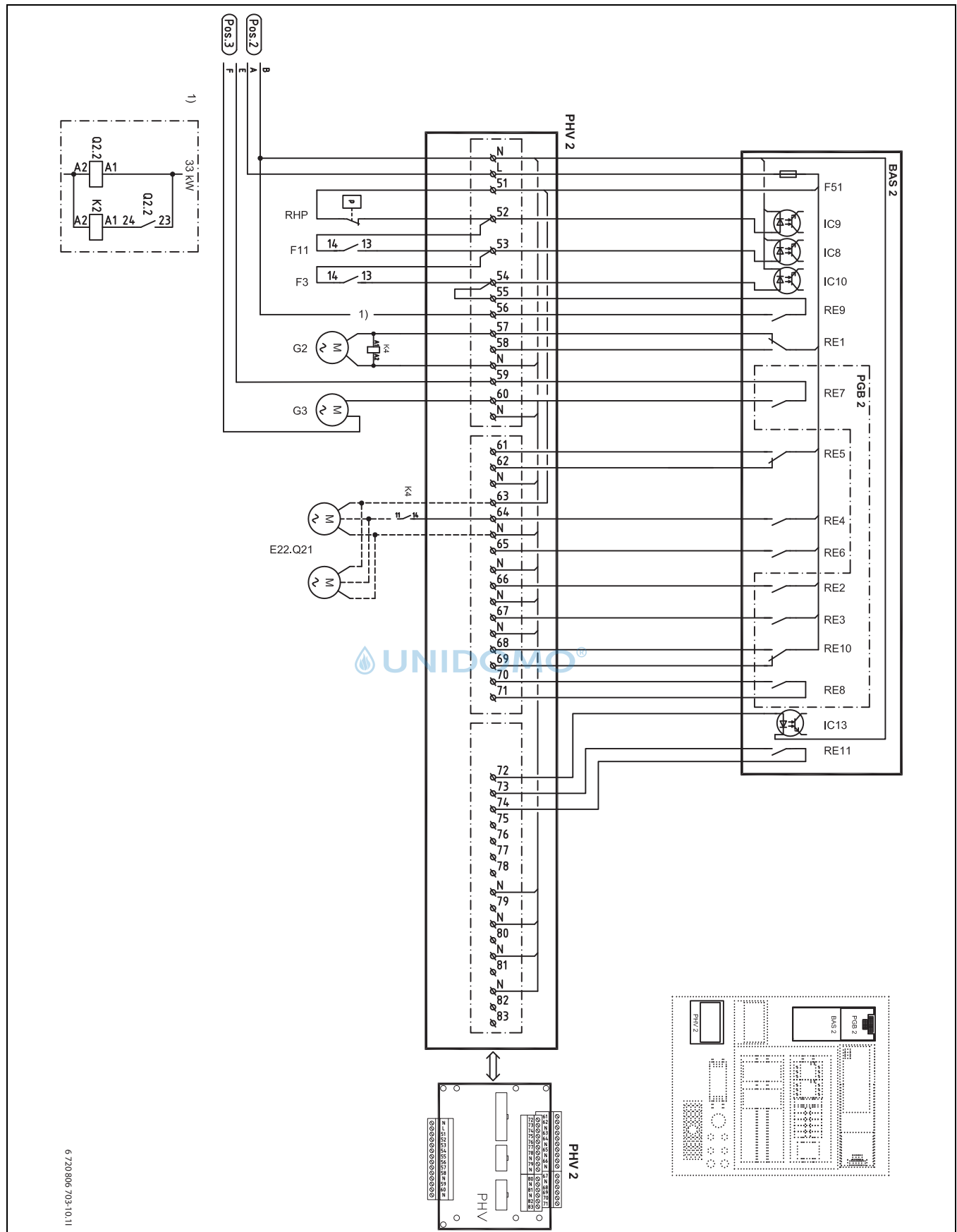
Bild 35 Schaltplan E22 Dreiphasen-Wechselstrom
