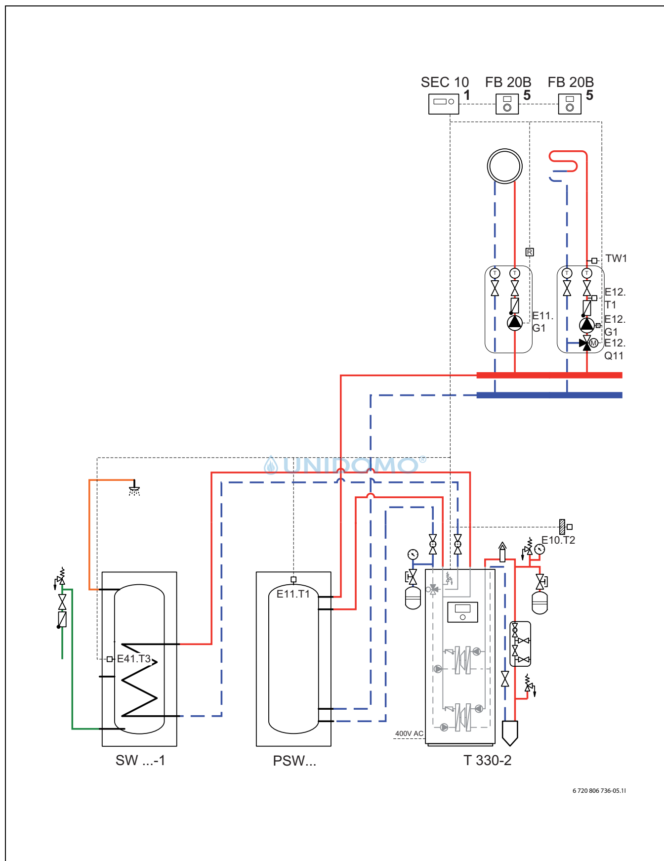
Bild 10 Heizkreis und Pufferspeicher, kein Zuheizer (→ Kapitel 9.2.1, 9.3)
