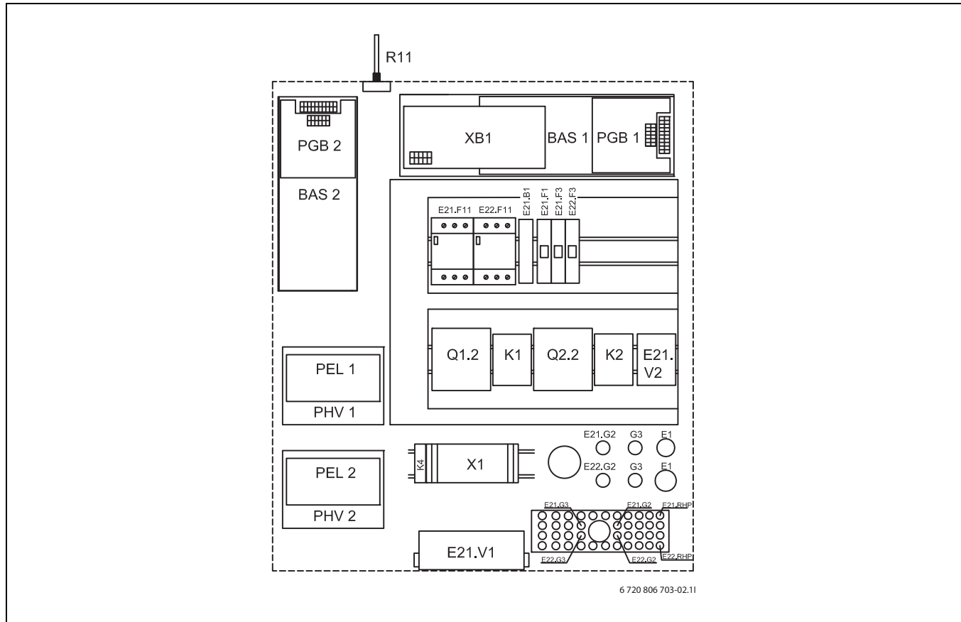
Bild 26 Übersicht Schaltkasten
