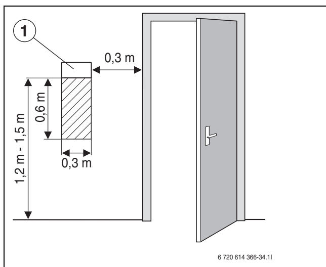
Bild 15 Empfohlener Montageplatz für Raumtemperaturfühler T5
