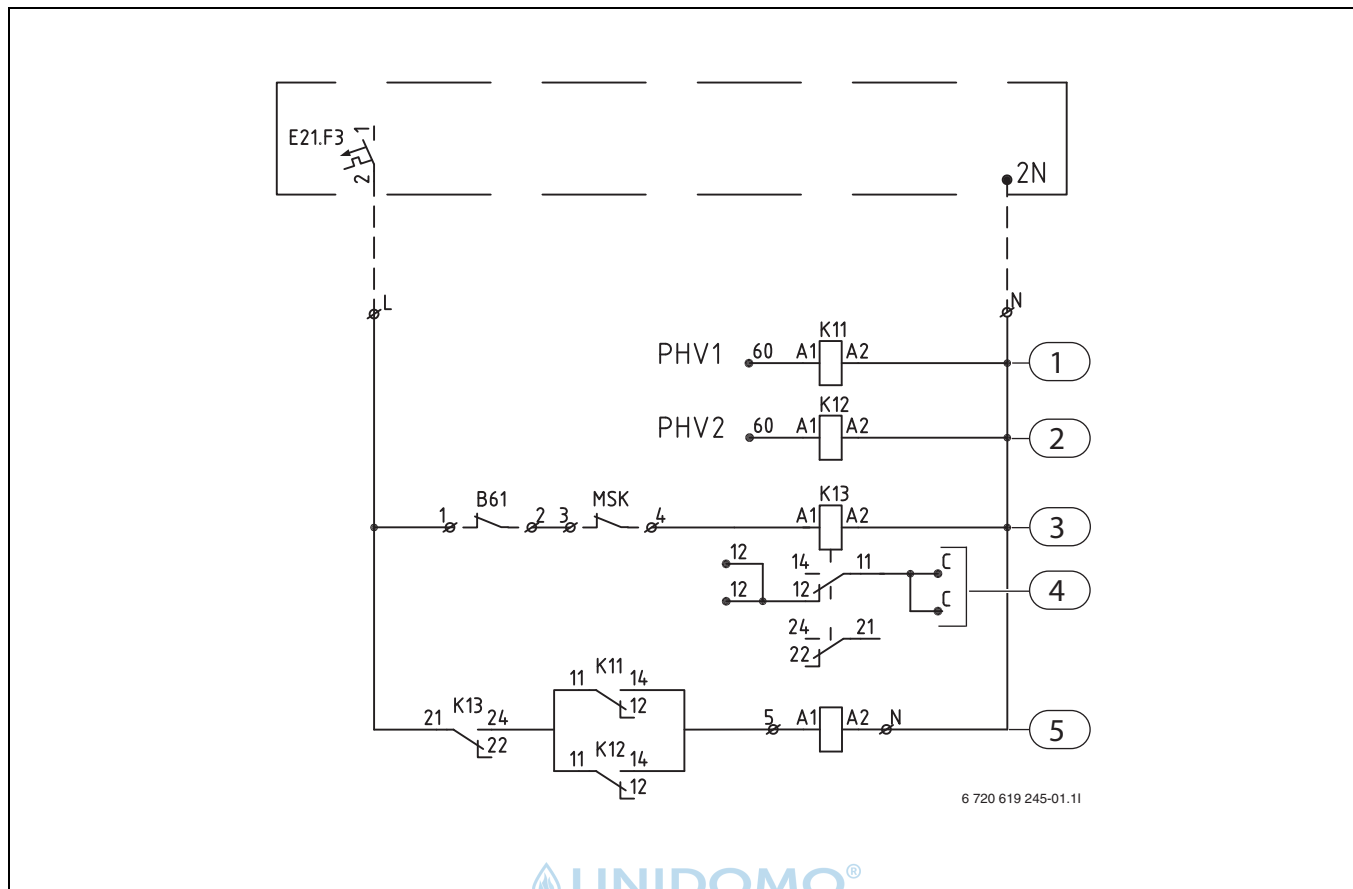
Bild 24 Übersicht Anschluss Elektroschaltschrank - Wärmepumpe
