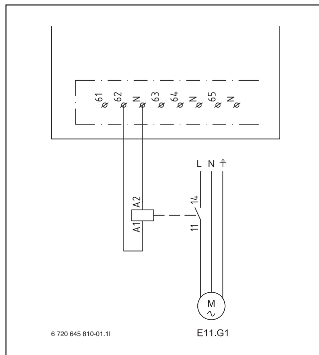
Bild 45 Anschluss einer Hocheffizienzpumpe E11.G1
