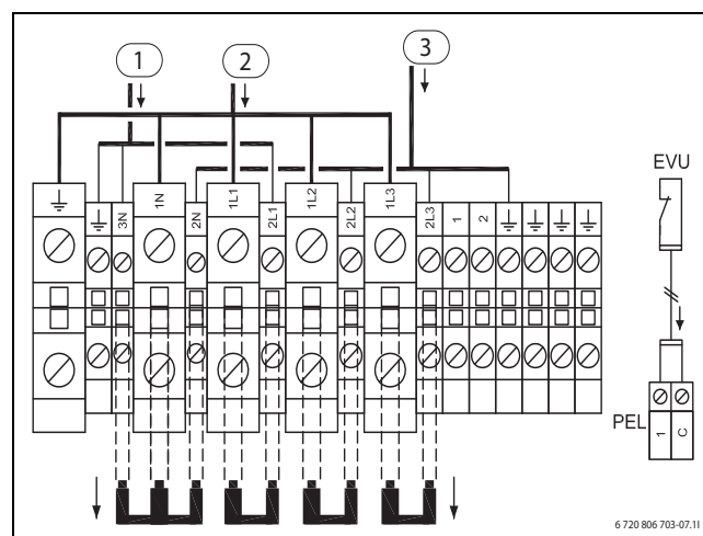
Bild 32 Anschlüsse Alternative B
