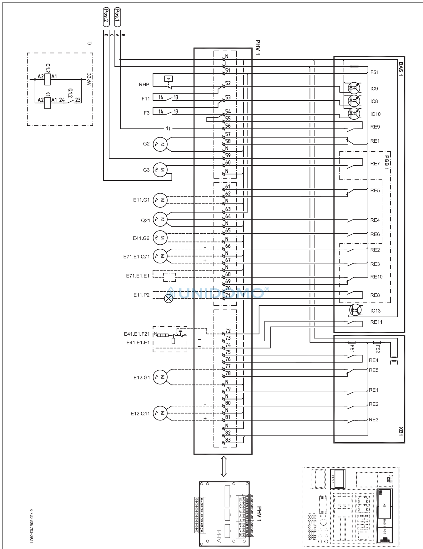
Bild 34 Schaltplan E21 Dreiphasen-Wechselstrom
