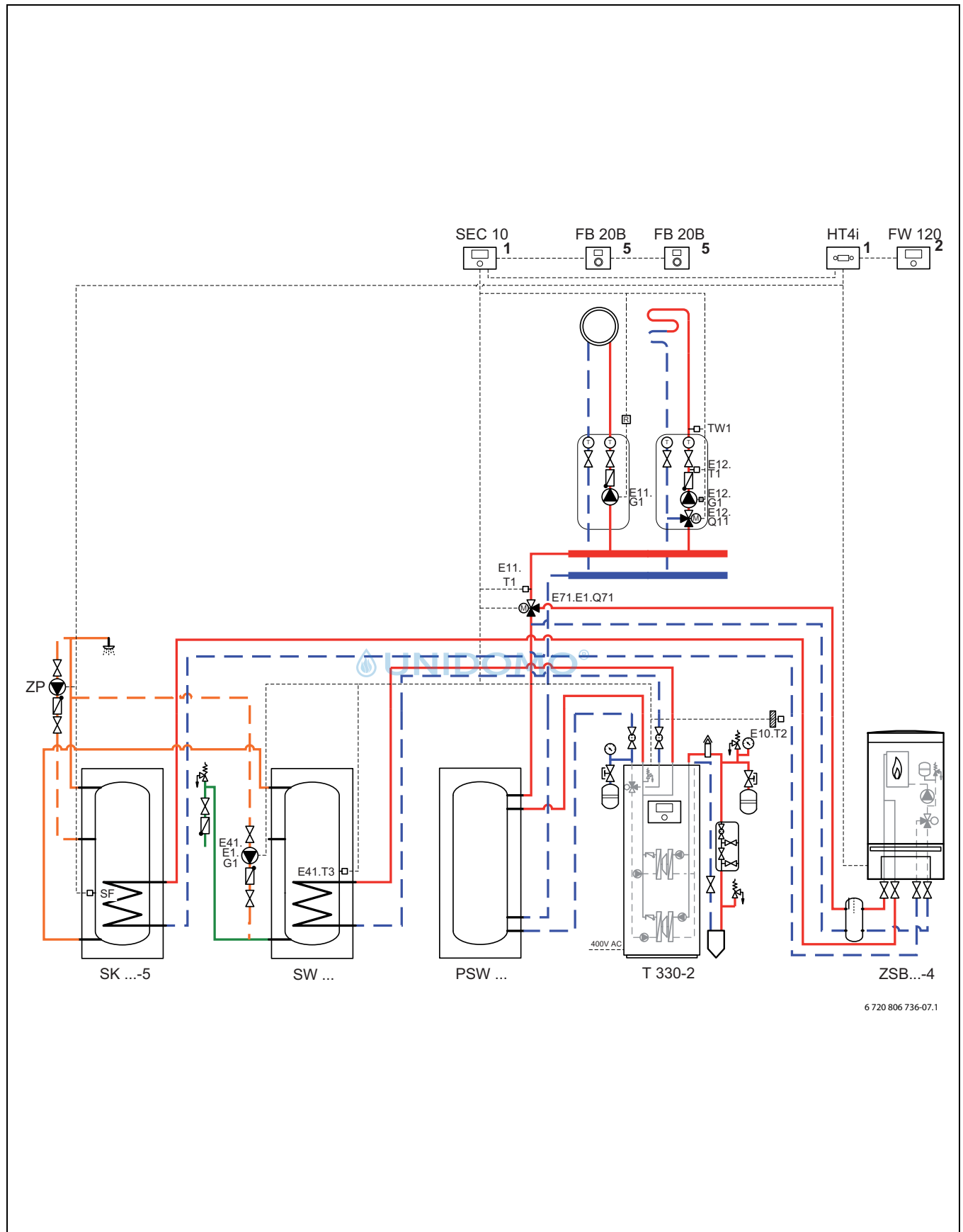
Bild 11 Heizkreis, Zuheizer mit Mischer und Pufferspeicher (→ Kapitel 9.2.1, 9.3)
