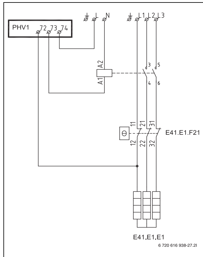
Bild 43 Anschluss elektr. Zuheizers Warmwasser
