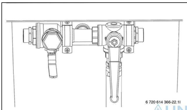
Bild 19 Befüllstation in Mischposition
