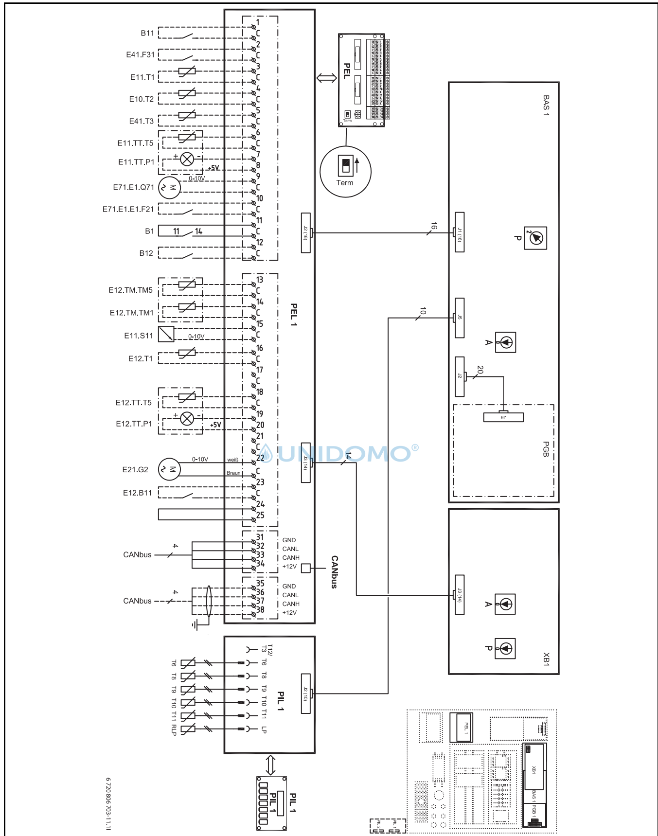
Bild 36 Schaltplan E21 Niederspannung
