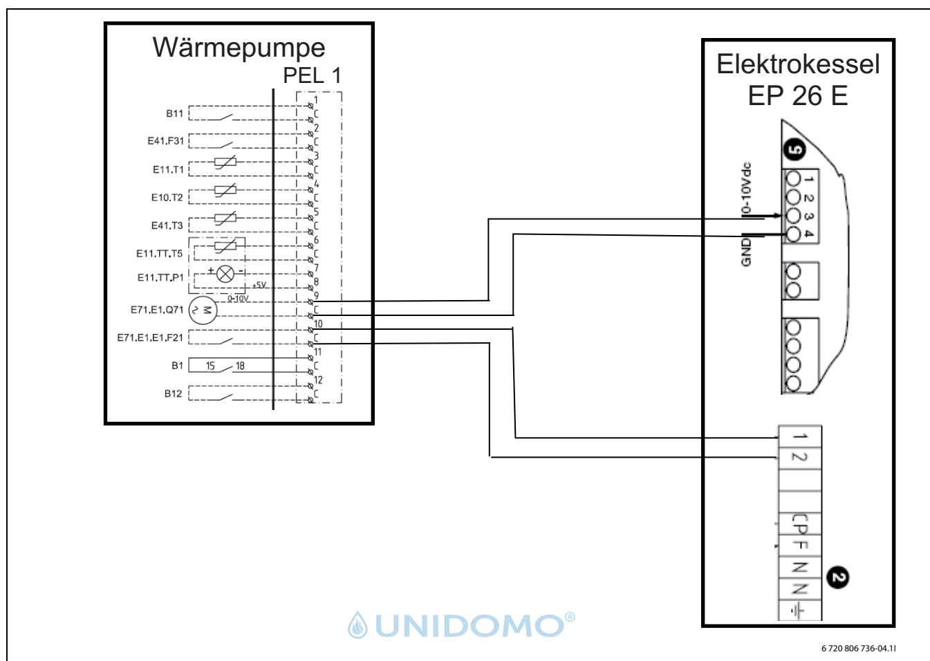
Bild 41 Anschluss der Wärmepumpe zum externen Elektroheizer EP 26 E
