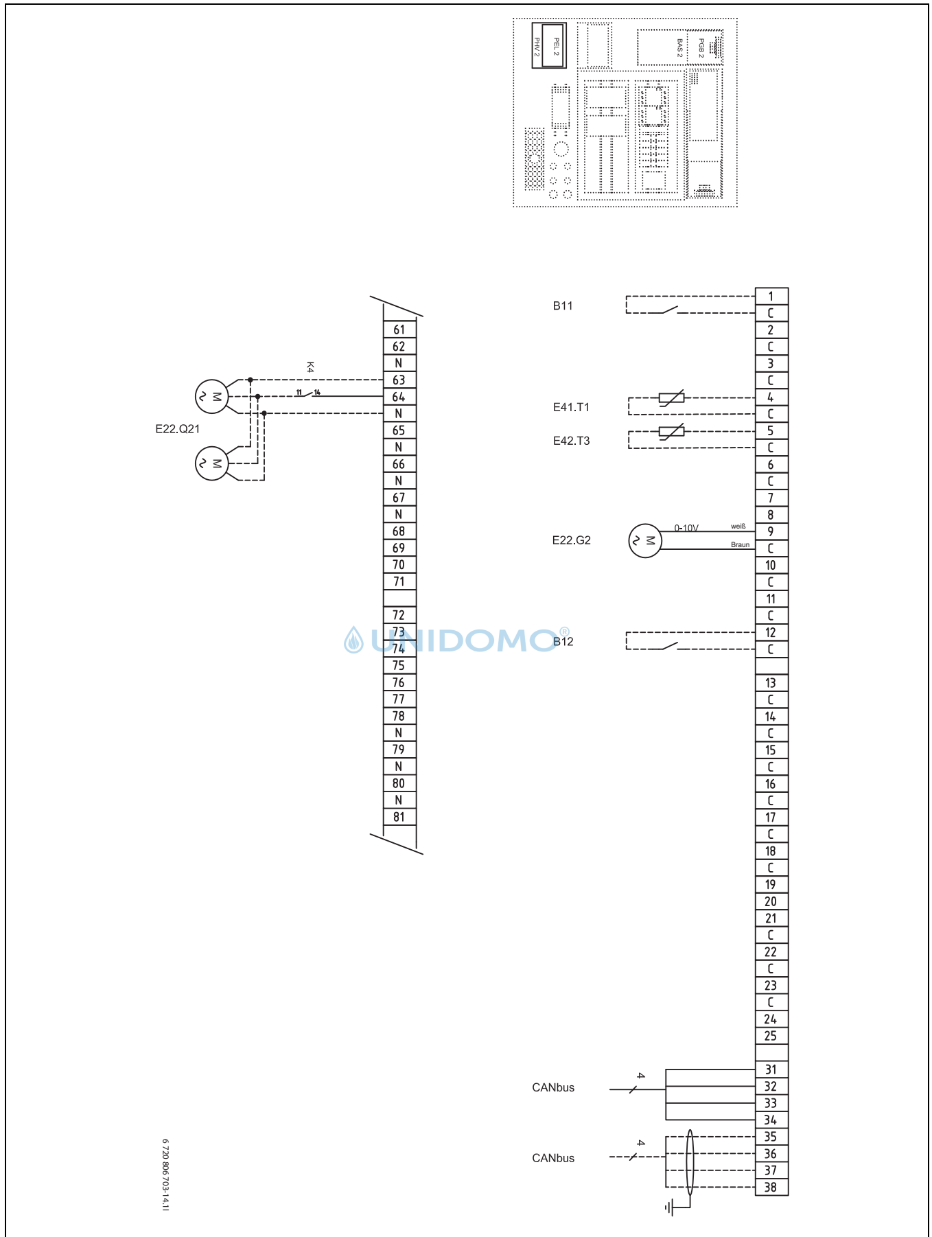
Bild 39 Externe Anschlüsse E22
