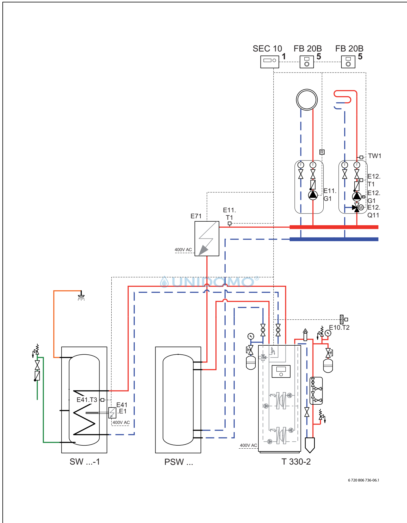
Bild 12 Heizkreis, elektrischer Zuheizier und Pufferspeicher (→ Kapitel 9.2.1, 9.3)
