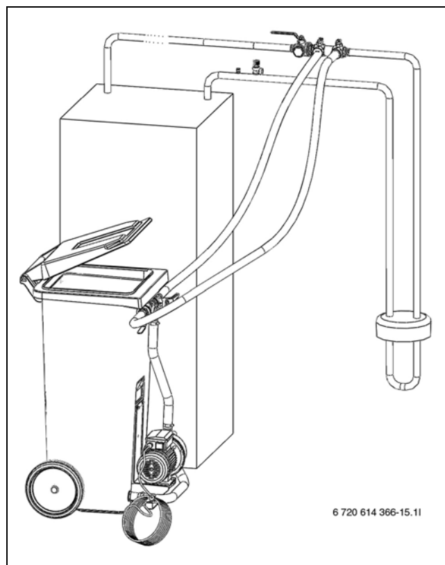
Bild 17 Befüllen mit Befüllstation
