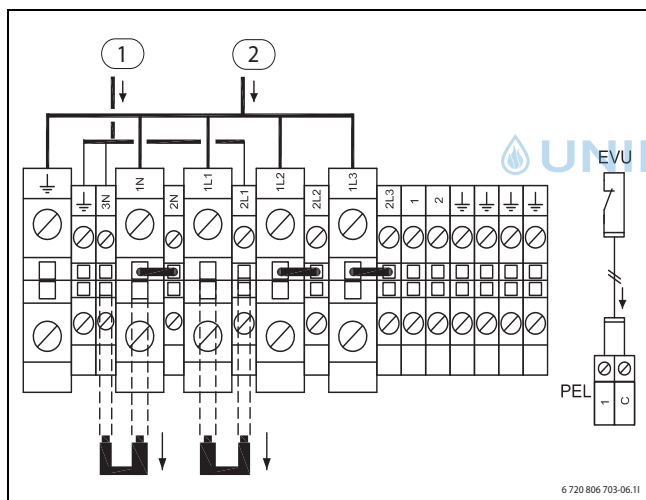
Bild 31 Anschlüsse Alternative A
