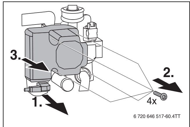
Bild 61 Heizungspumpe ausbauen
