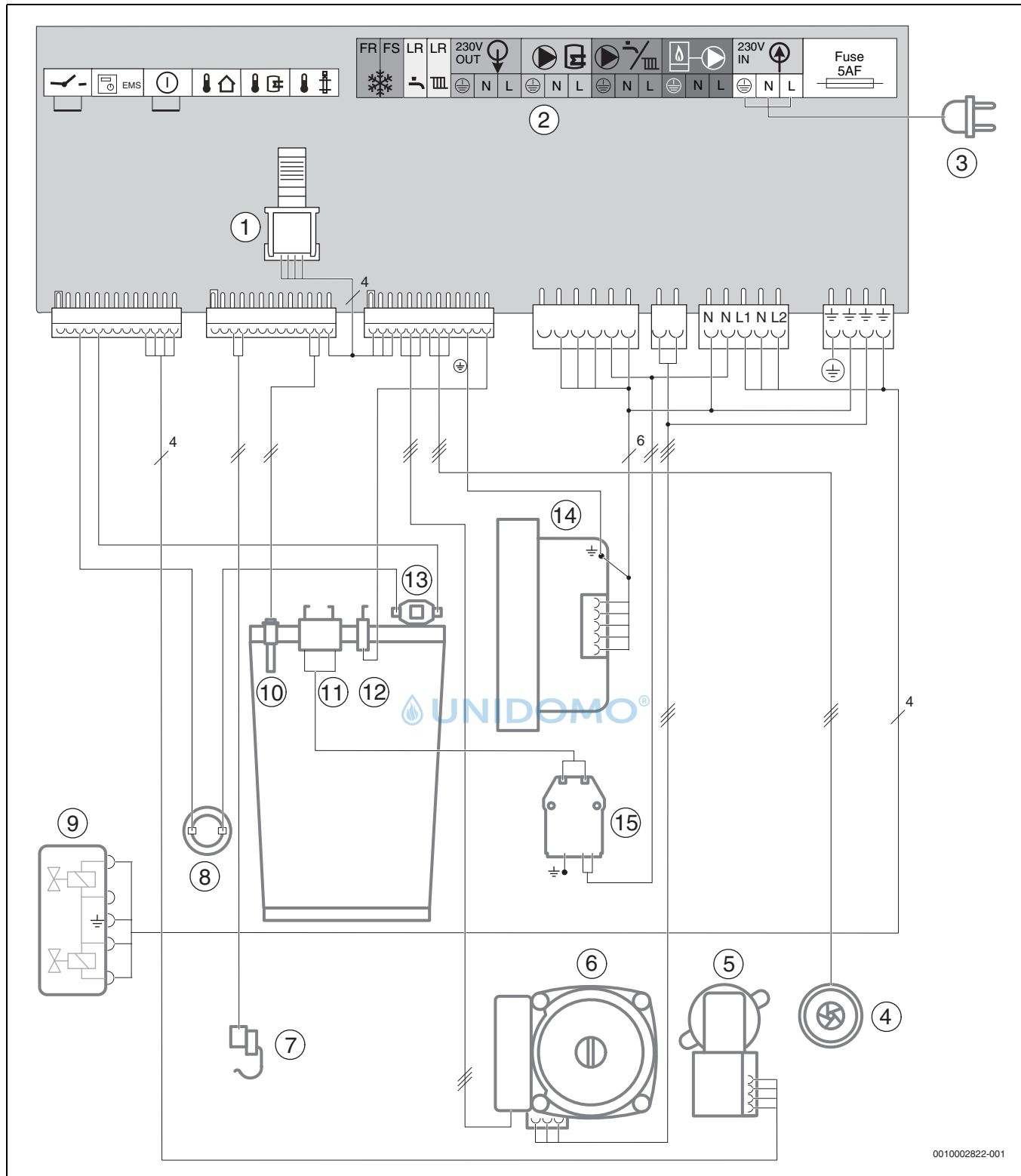
Bild 71 Elektrische Verdrahtung
