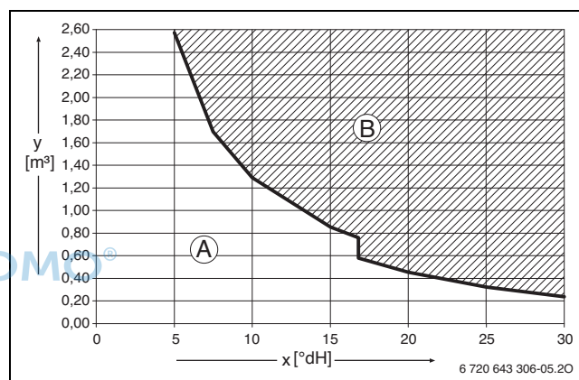
Bild 17 Anforderungen an Füll- und Ergänzungswasser Geräte < 50 kW
