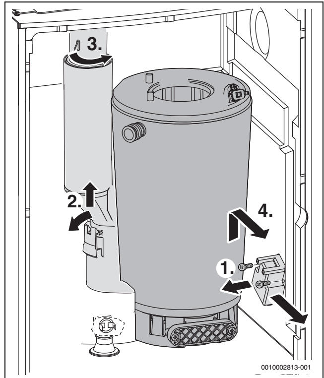
Bild 68 Wärmeblock ausbauen
