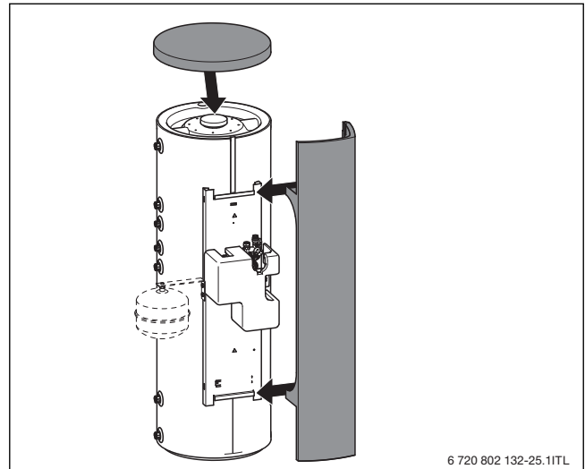
Bild 26 Verkleidung montieren und Deckel aufsetzen
