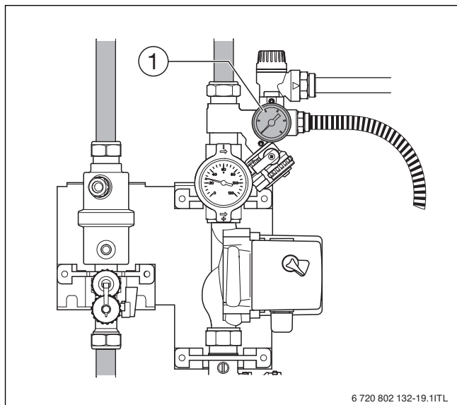
Bild 22 Manometeranzeige prüfen
