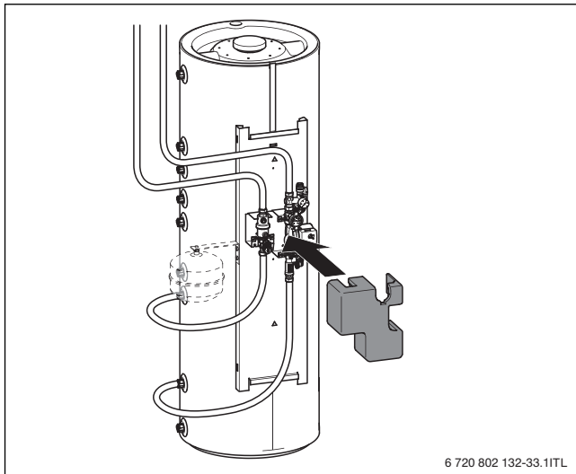
Bild 25 Isolierhaube aufsetzen
