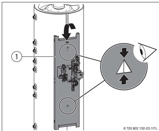
Bild 12 Montageplatte ausrichten
