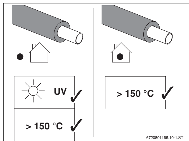
Bild 9 Mindestanforderungen der Dämmung
