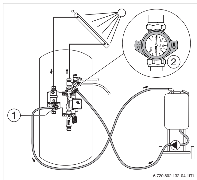
Bild 19 Befüllen oberhalb der Solarstation
