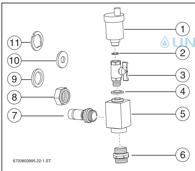
Bild 61 Lieferumfang Entlüftersatz
