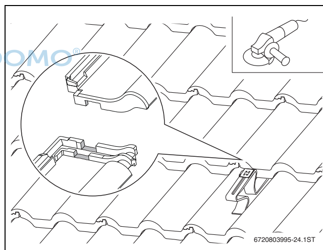
Bild 29 Profilierte Dachziegel
