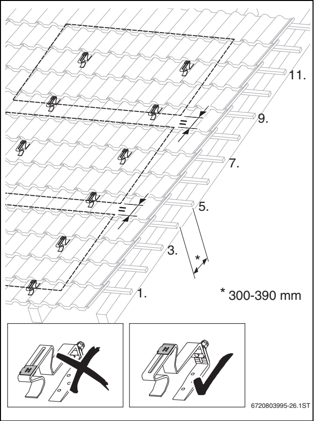
Bild 20 Abstände der Dachhaken bei 3 waagerechten Kollektoren
