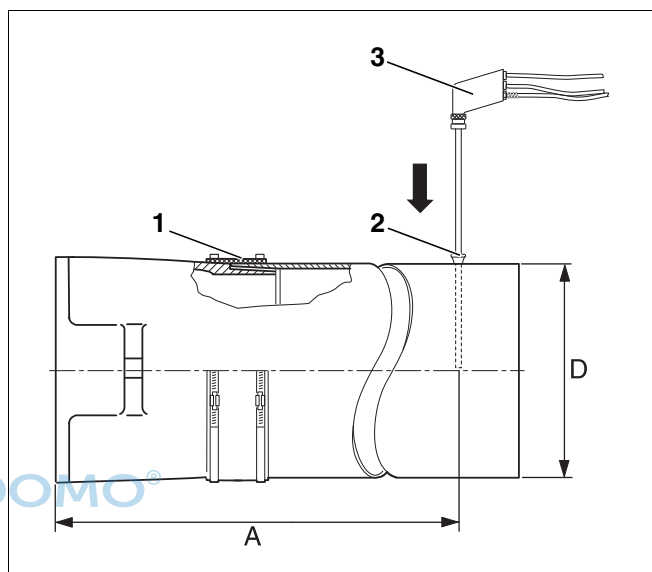
Abb. 31 Messwerte aufnehmen
