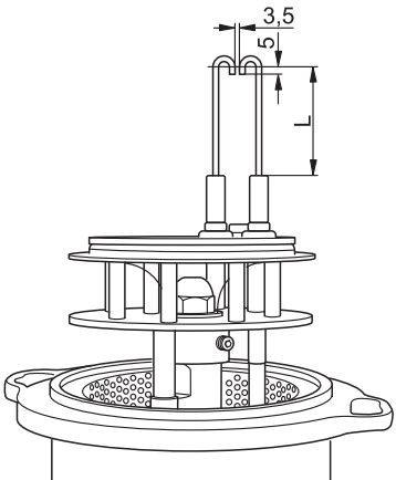
Abb. 5 Zündelektrode – Maß „L“ (Maße in mm)
