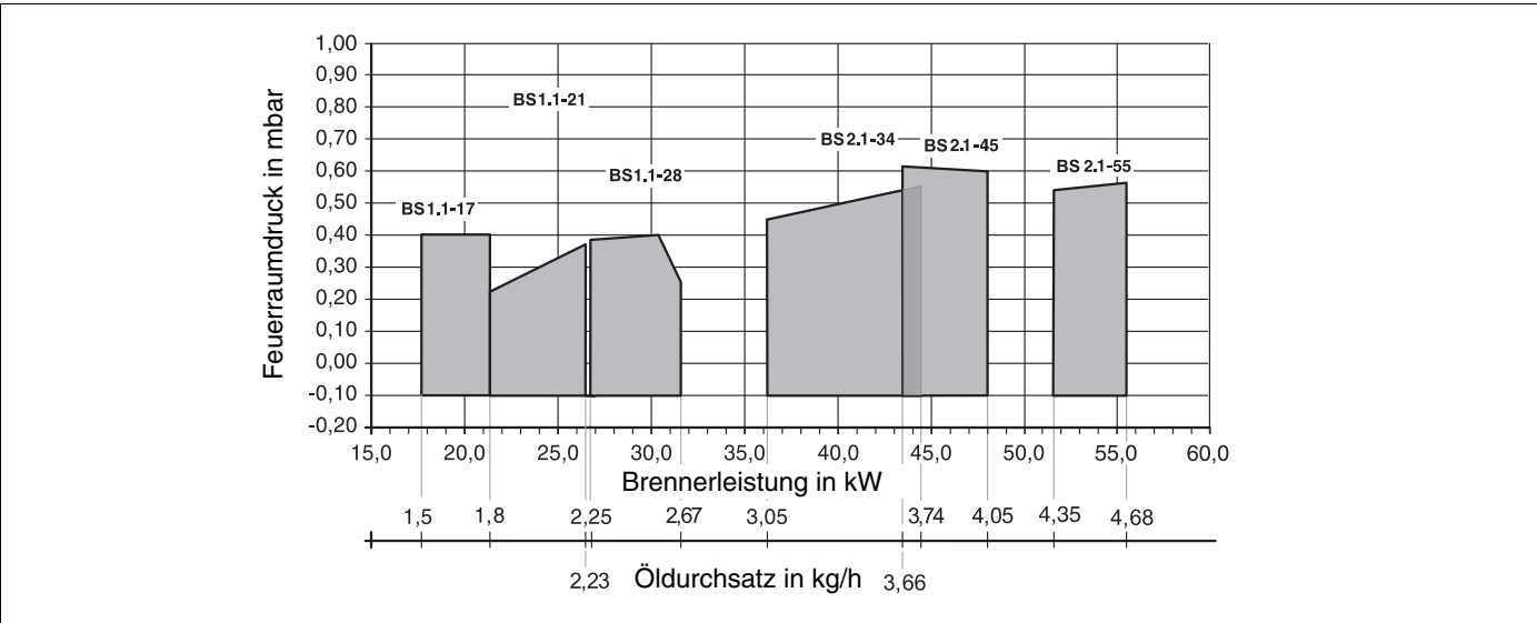
Abb. 11 Feuerdruck, Öldurchsatz und Brennerleistung
