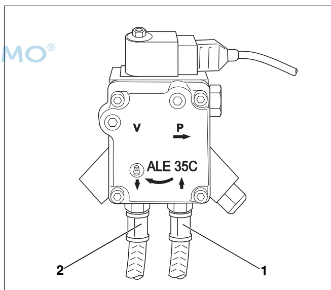
Abb. 27 Ölpumpe – Suntec
