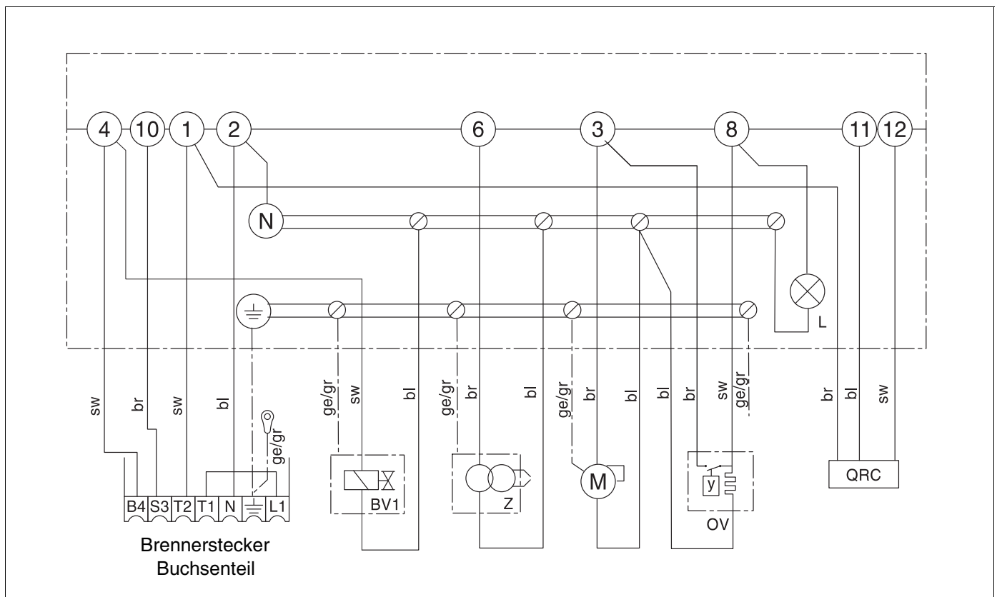
Abb. 12 Verdrahtungsplan – Sockel HG-A
