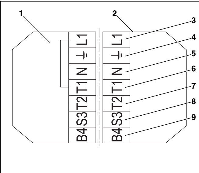
Abb. 13 Brenneranschlussleitung – 7-poliger-Brennerstecker
