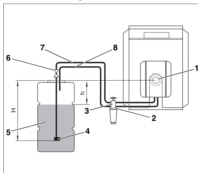
Abb. 61 Öltank unterhalb der Ölpumpe
