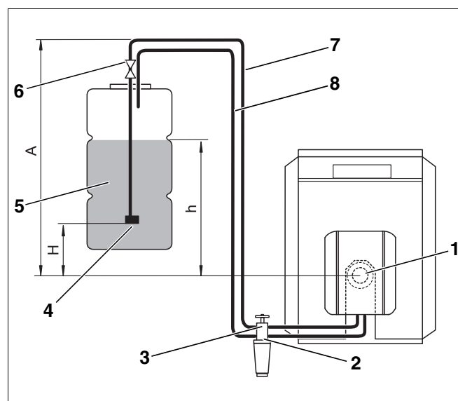
Abb. 60 Öltank oberhalb der Ölpumpe
