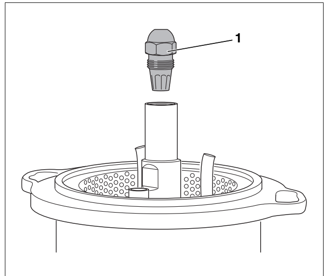
Abb. 48 Düse demontieren
