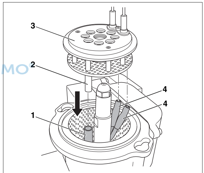
Abb. 49 Mischsystem montieren
