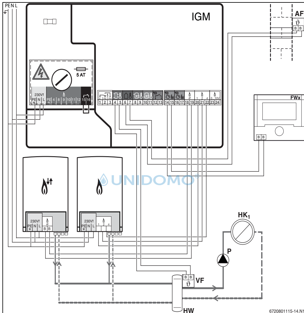
Afb. 29 Basis aansluitschema met openverdelers
