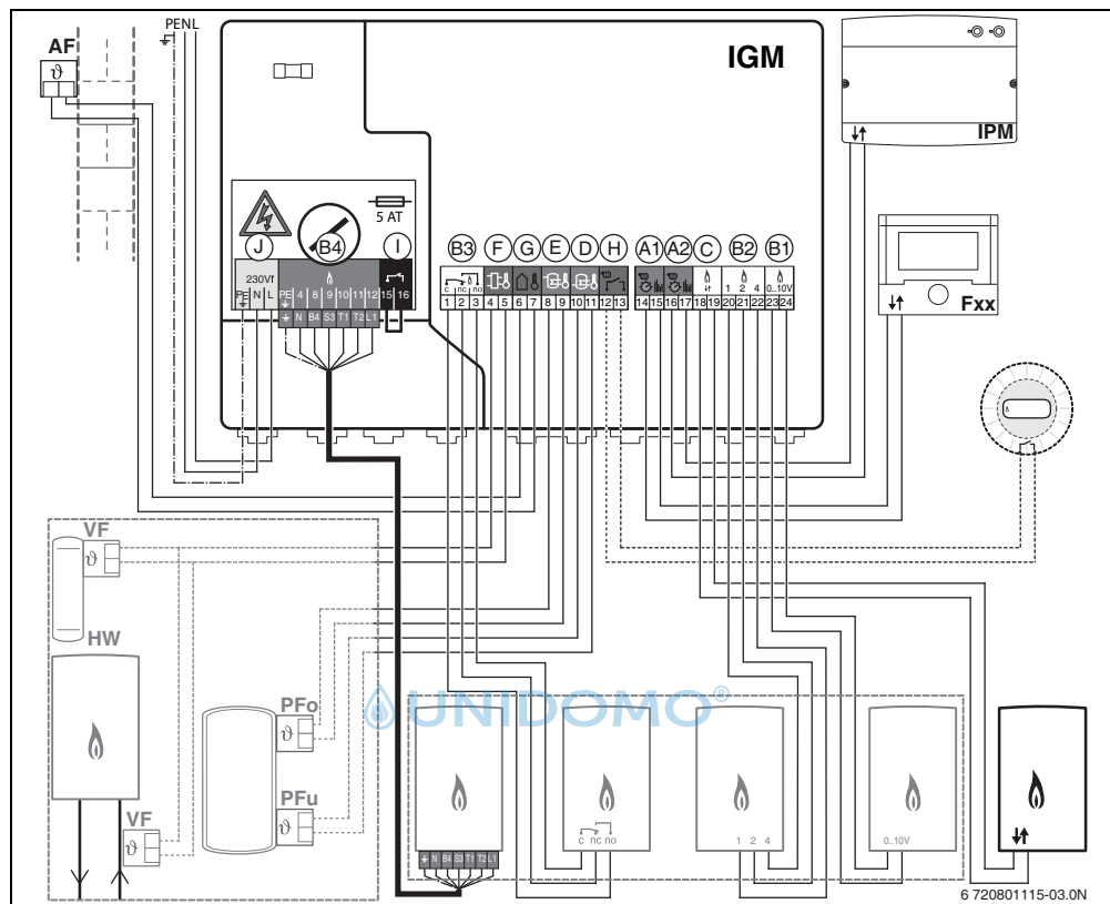
Afb. 26 Aansluitschema
