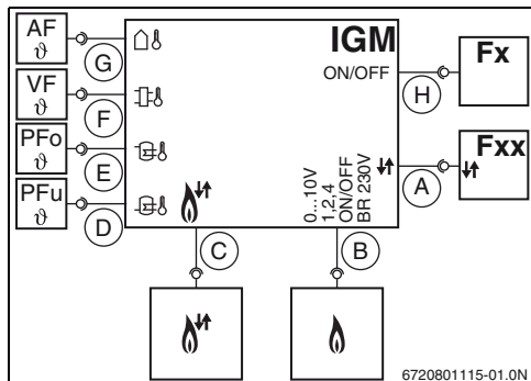
Afb. 19 Basisfunctie schema
