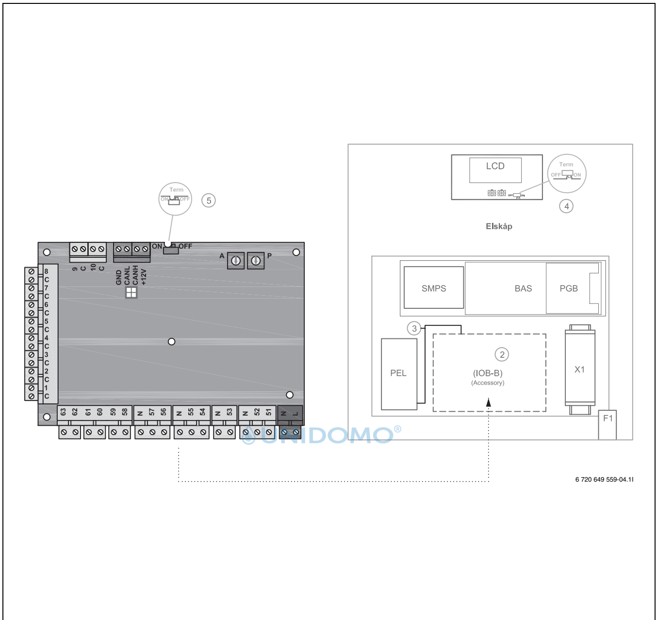
Bild 17 IOB-B-Anordnung im Schaltkasten SEC10-1
