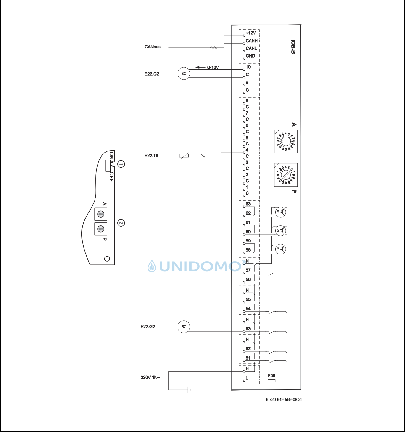
Bild 21 Schaltplan bei Kaskadenschaltung
