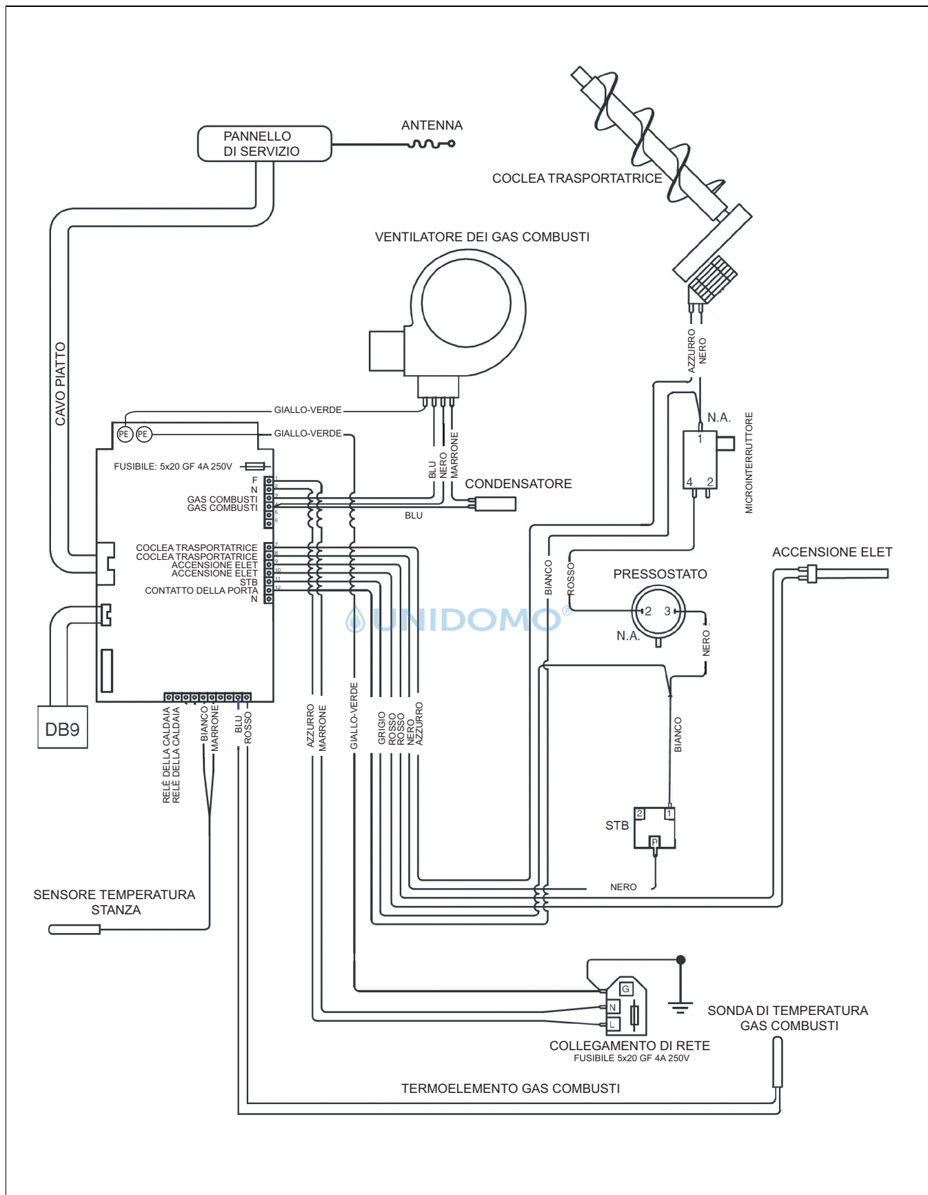
Fig. 15 Schema elettrico
