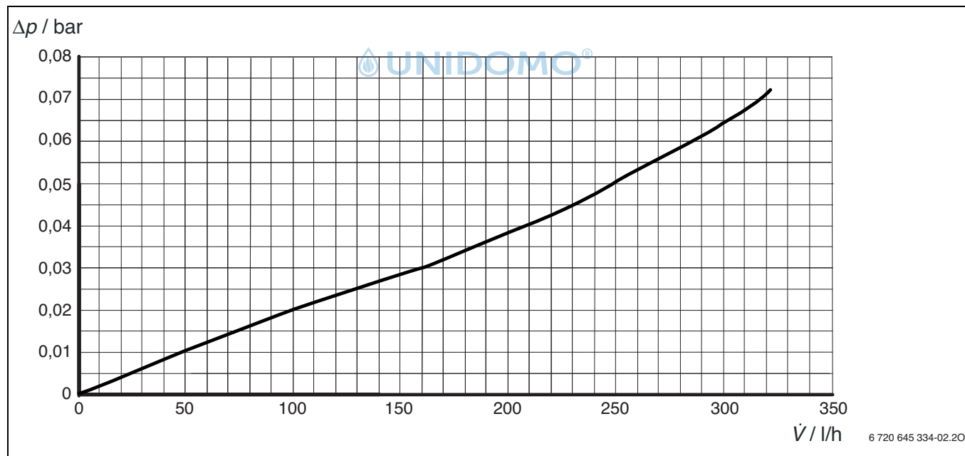
Bild 11 Warmwasserseitiger Druckverlust
