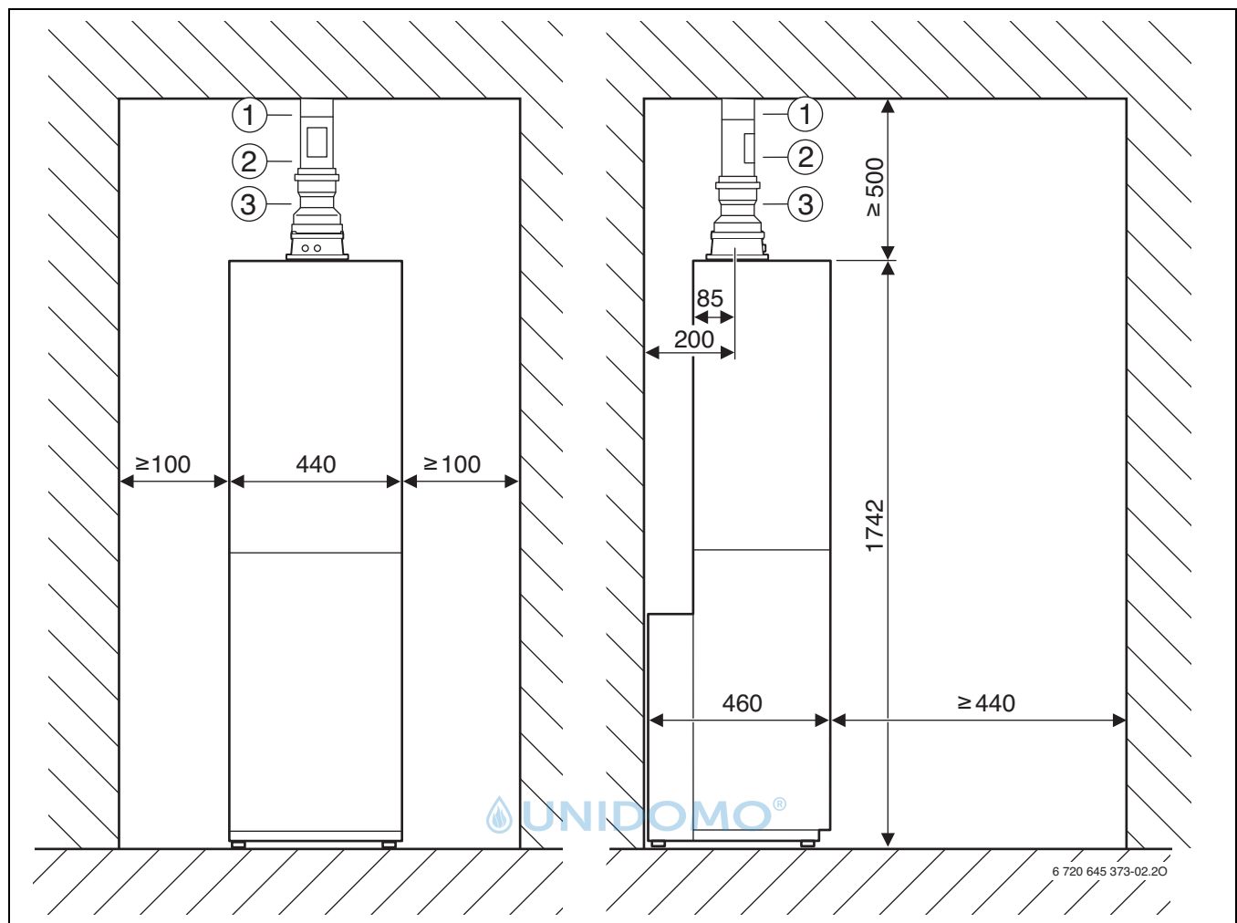
Bild 7 Flachdach
