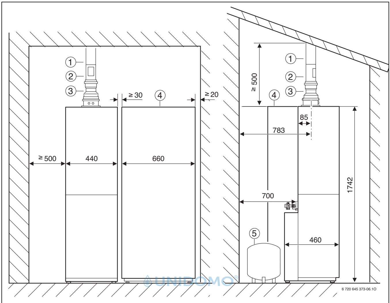
Bild 10 Flachdach
