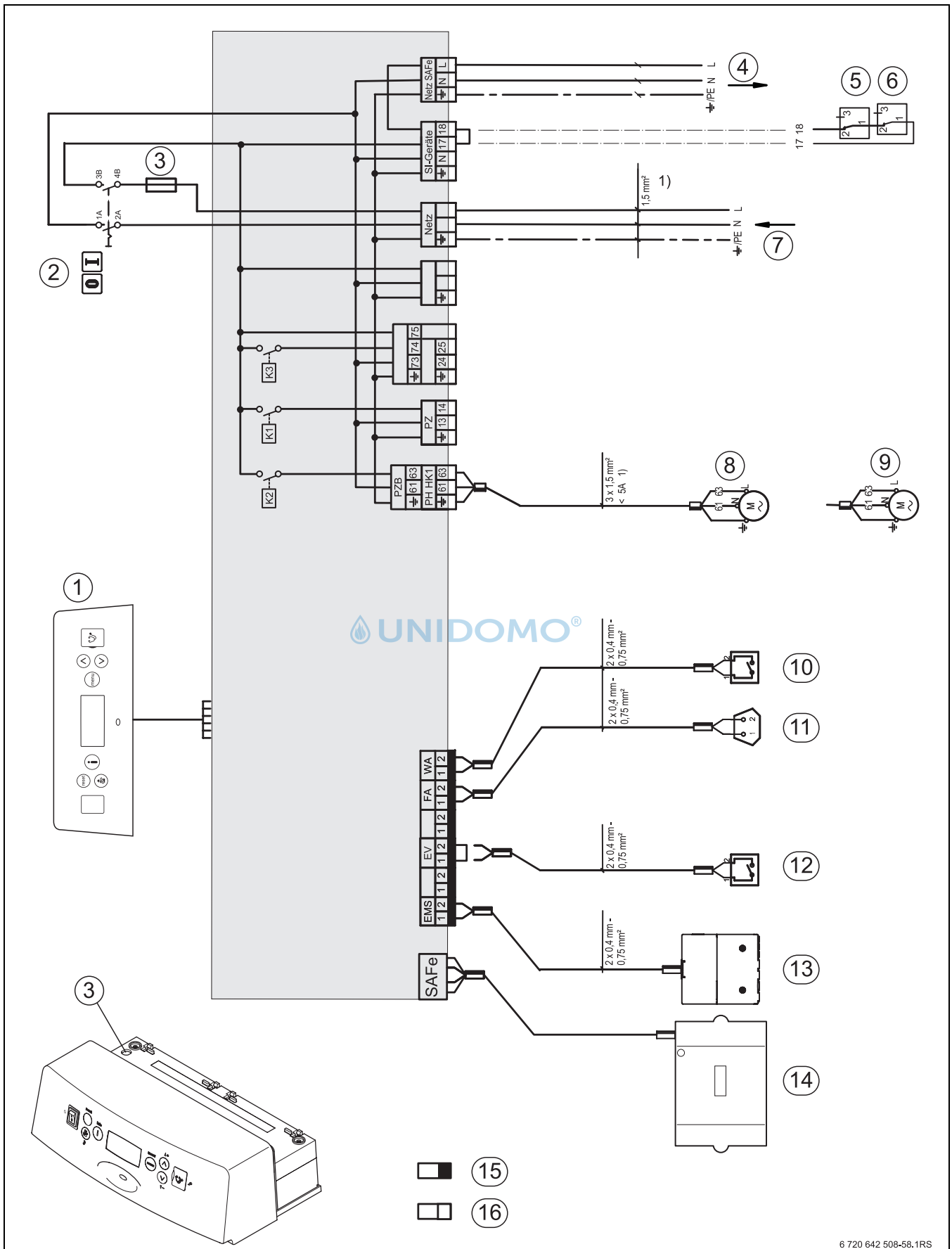
Bild 8 Anschlussplan Hauptleiterplatte
