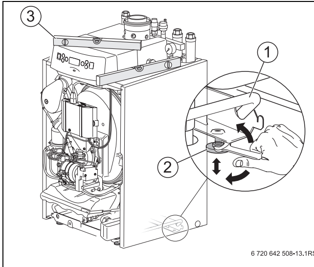
Bild 20 Heizkessel ausrichten
