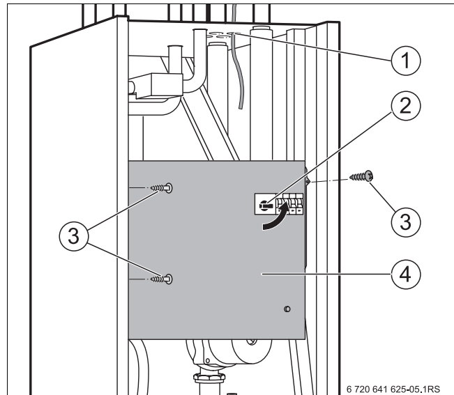
Bild 4 Schaltkasten
