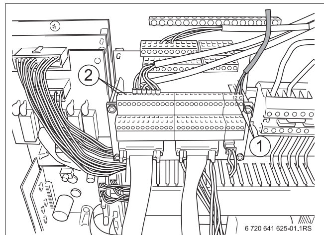
Bild 5 Klemmleiste
