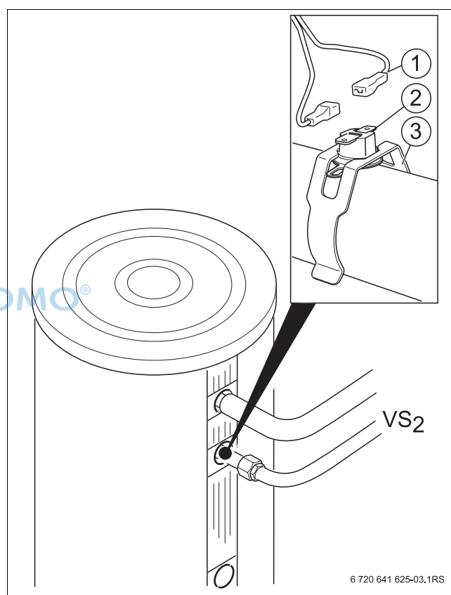
Bild 2 Anschlussstelle Temperaturschalter
