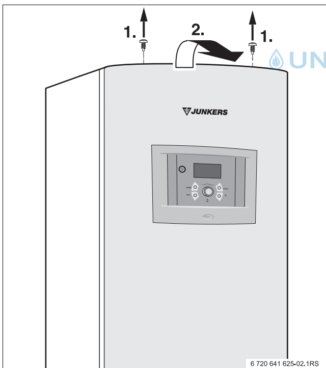
Bild 3 Frontverkleidung
