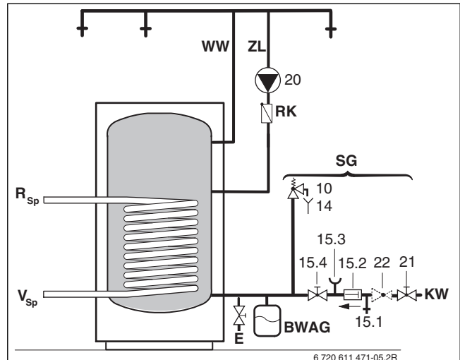
Bild 6 Trinkwasserseitiges Anschluss-Schema
