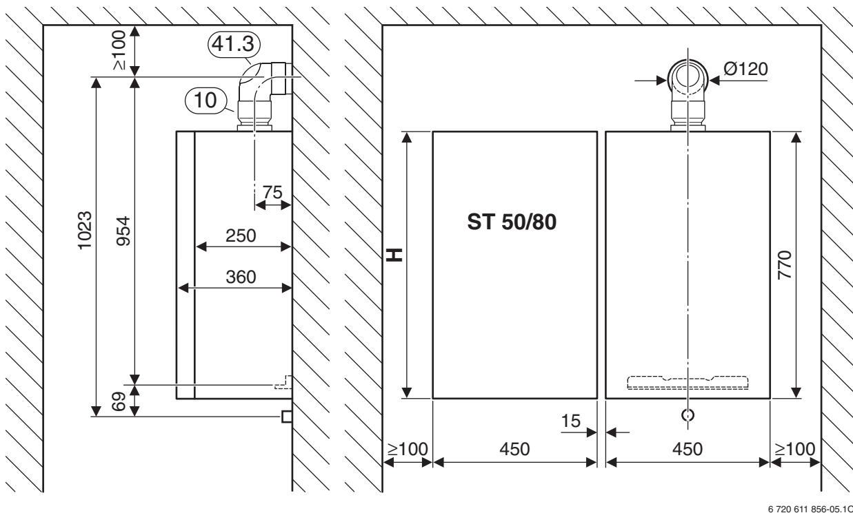
Bild 4 Gas-Kesseltherme neben Speicher ST 50/80
