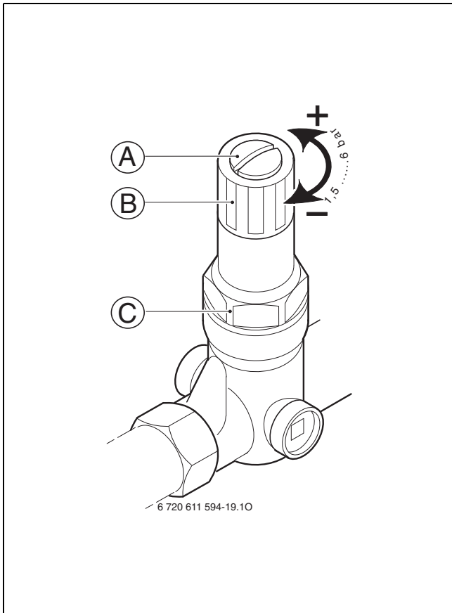
6 Nr. 430 - P 2 = 4 bar (1,5...6 bar)
