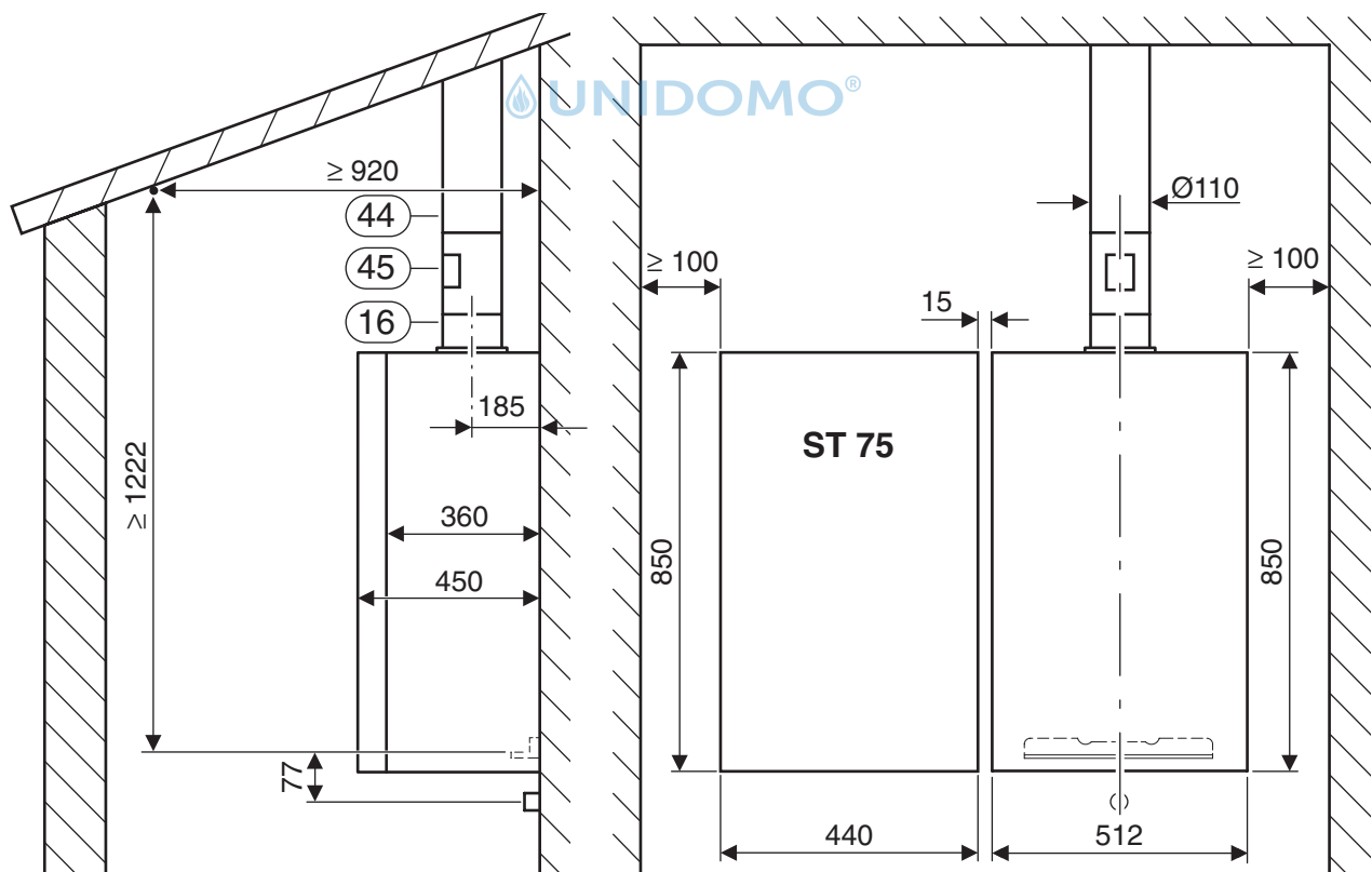
Bild 5 Schrägdach
