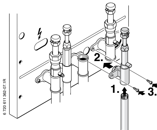
Bild 6 Kaltwasseranschluss montieren
