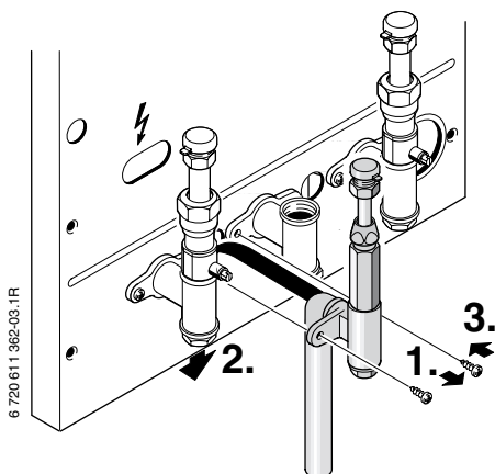
Bild 2 Warmwasseranschluss montieren
