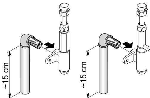
Bild 1 Anschlüsse vormontieren
