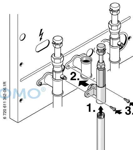
Bild 5 Warmwasseranschluss montieren
