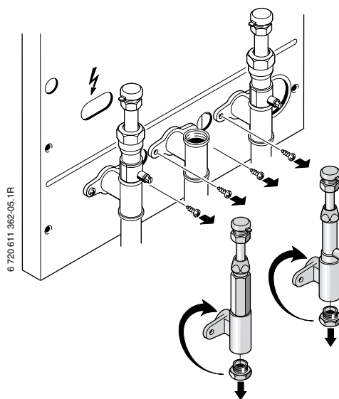
Bild 4 Verschlusschraube ummontieren
