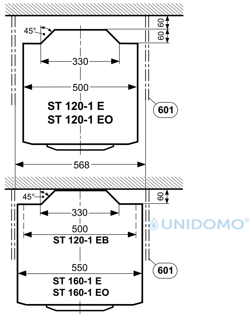
Bild 6 Maße mit Holzummantelung GWZ-1.
