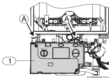
Bild 1 Steuerungskasten entnehmen
