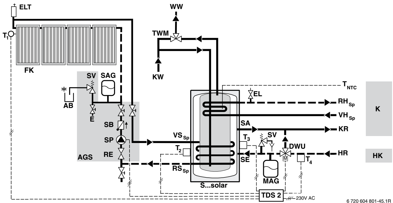
Bild 5 Solare Heizungsunterstützung mit SP... solar. Vereinfachtes Anlagenschema (montagegerechte Darstellung und weitere Möglichkeiten in den Planungsunterlagen).
