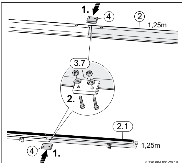
Bild 35 Erweiterung um einen Flachkollektor
