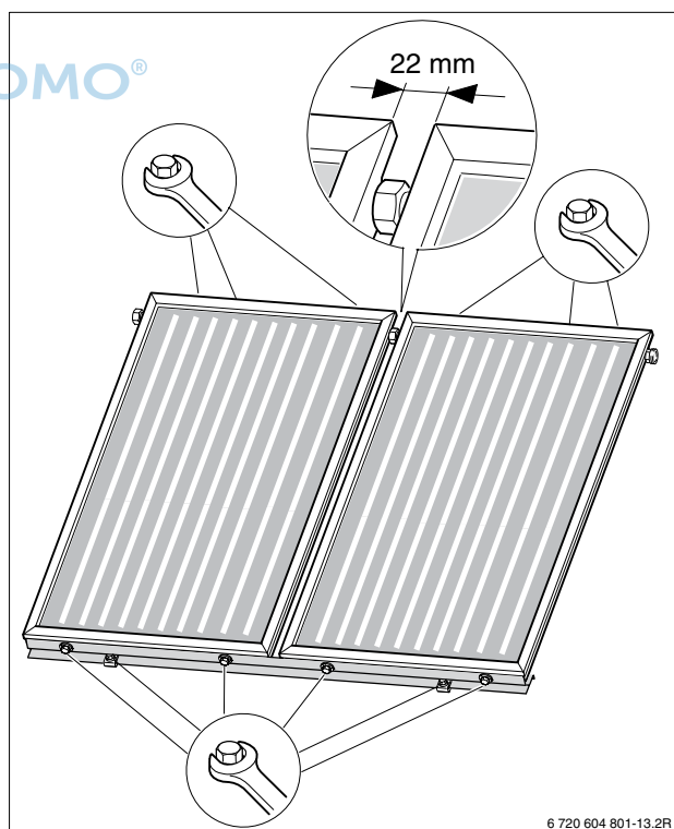
Bild 28 Flachkollektoren ausrichten und befestigen
