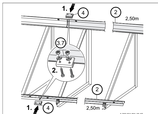
Bild 47 Erweiterung um zwei Flachkollektoren
