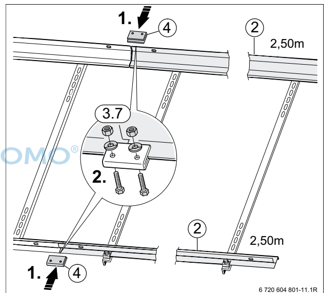
Bild 15 Erweiterung um zwei Flachkollektoren
