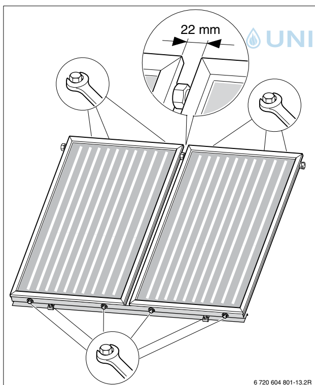
Bild 17 Flachkollektoren ausrichten und befestigen
