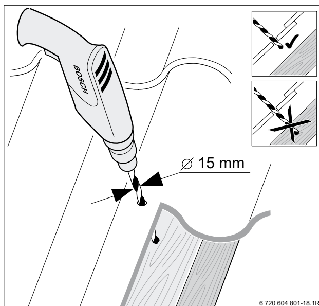
Bild 22 Dachpfanne durchbohren
