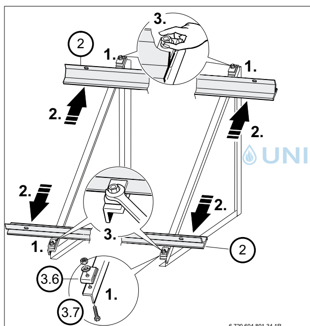
Bild 45 Trageprofile montieren
