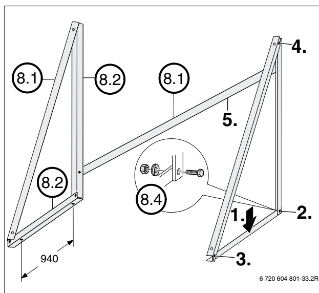
Bild 44 Flachdachgestell montieren
