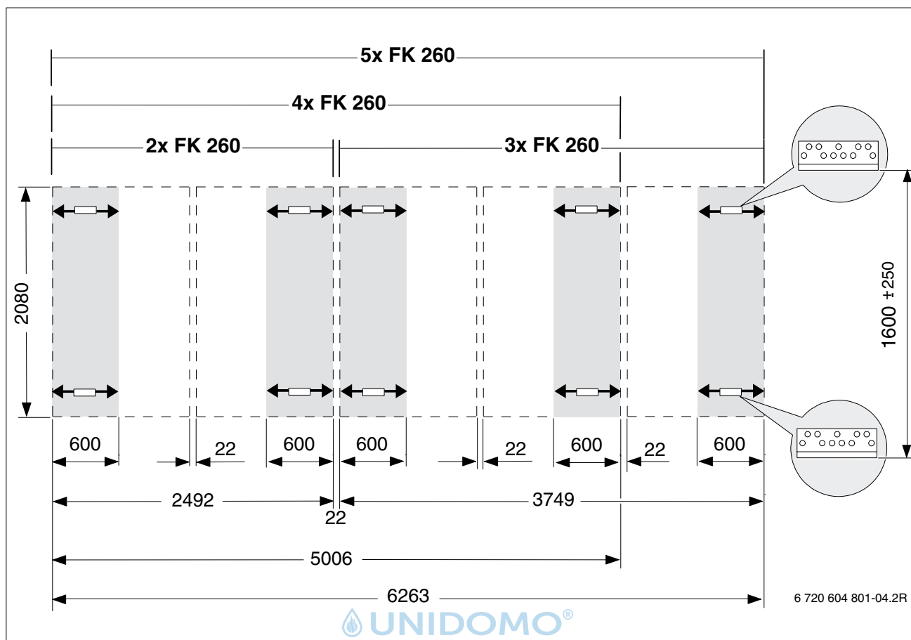
Bild 8 Kollektorfeldmaße und Toleranzbereiche für die Befestigung der Sparrenanker
