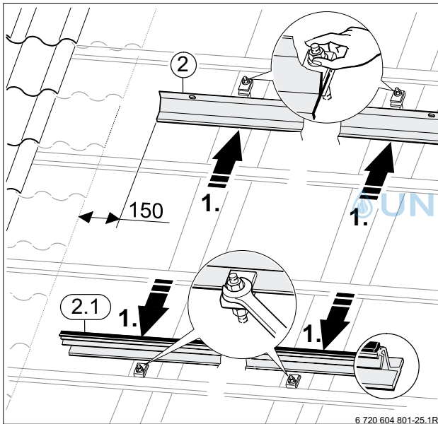
Bild 34 Trageprofile montieren
