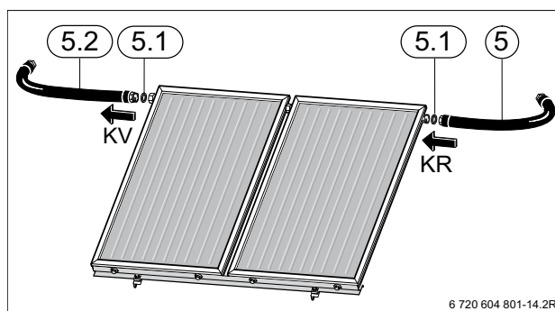
Bild 18 Flexible Schläuche anschließen
