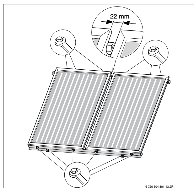
Bild 49 Flachkollektoren ausrichten und befestigen
