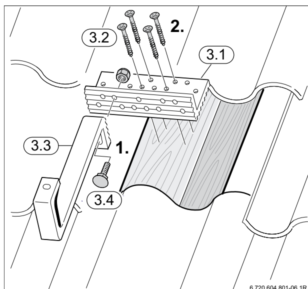
Bild 10 Sparrenanker befestigen
