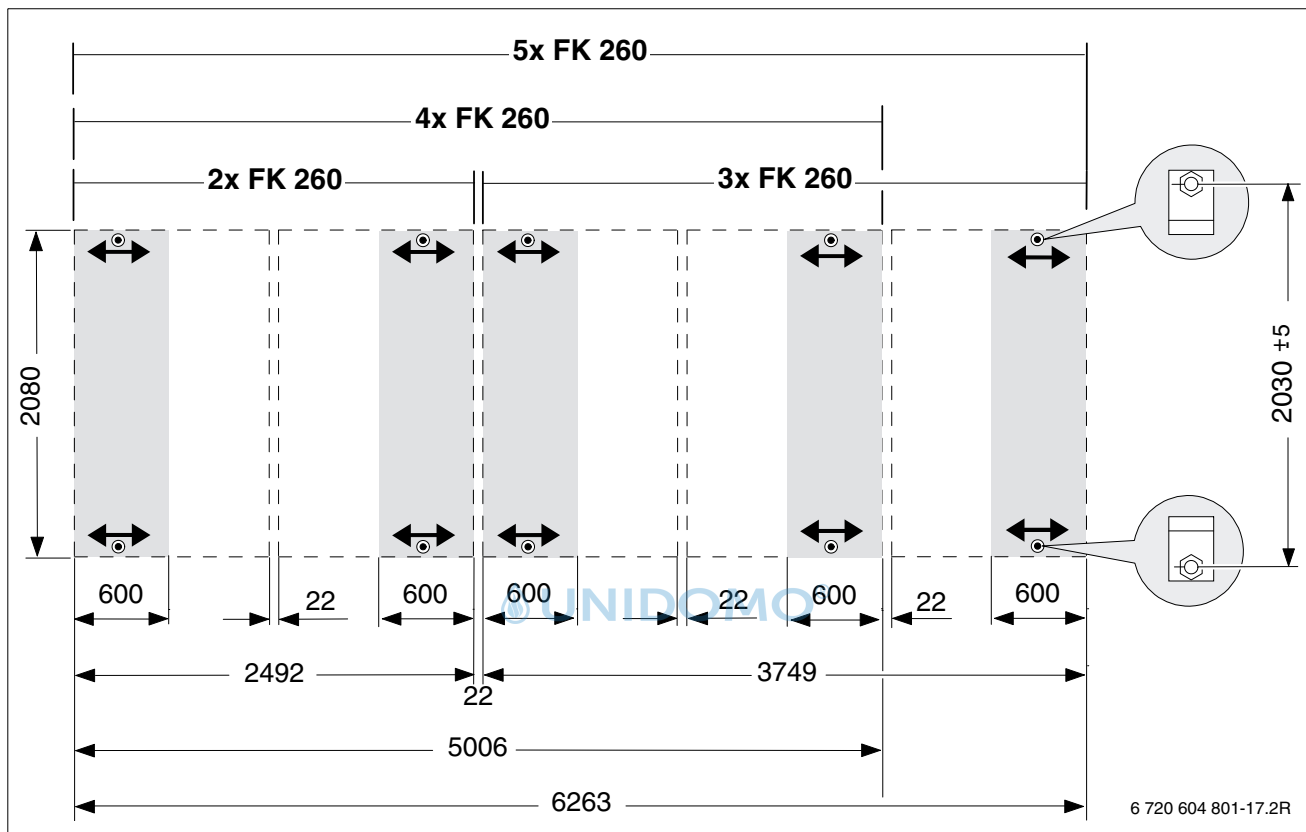
Bild 21 Kollektorfeldmaße und Toleranzbereiche für die Befestigung der Stockschrauben
