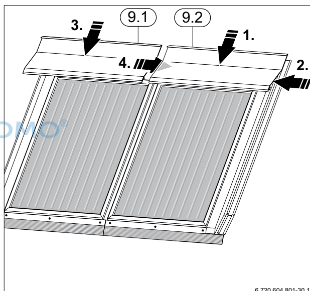
Bild 41 Blechteile oben rechts und links montieren
