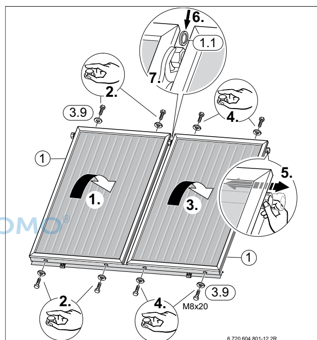
Bild 48 Flachkollektoren einlegen, mit Schrauben sichern und zusammenschließen
