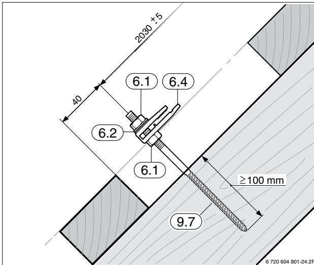
Bild 33 Stockschraube (Mindesteinschraubtiefe 100 mm) und Klemmstück Oberkante Lattung montieren
