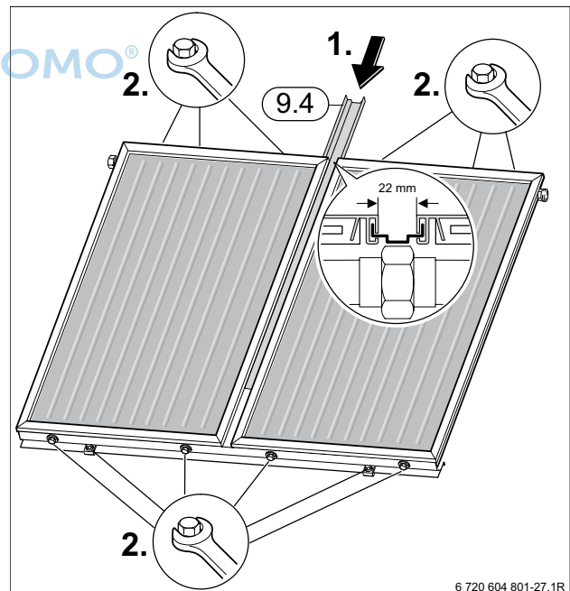
Bild 37 Flachkollektoren ausrichten, Abdeckschiene einschieben und Flachkollektoren befestigen.
