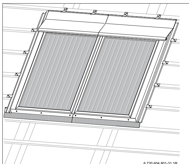
Bild 42 Blechhaften anbringen
