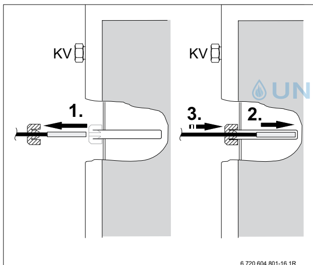
Bild 51 Temperaturfühler in Tauchrohr an der Kollektor-Vorlauf-Seite schieben
