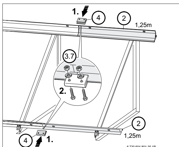
Bild 46 Erweiterung um einen Flachkollektor
