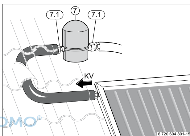
Bild 19 Entlüftertopf anschließen
