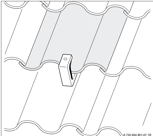
Bild 11 Dachpfanne einpassen
