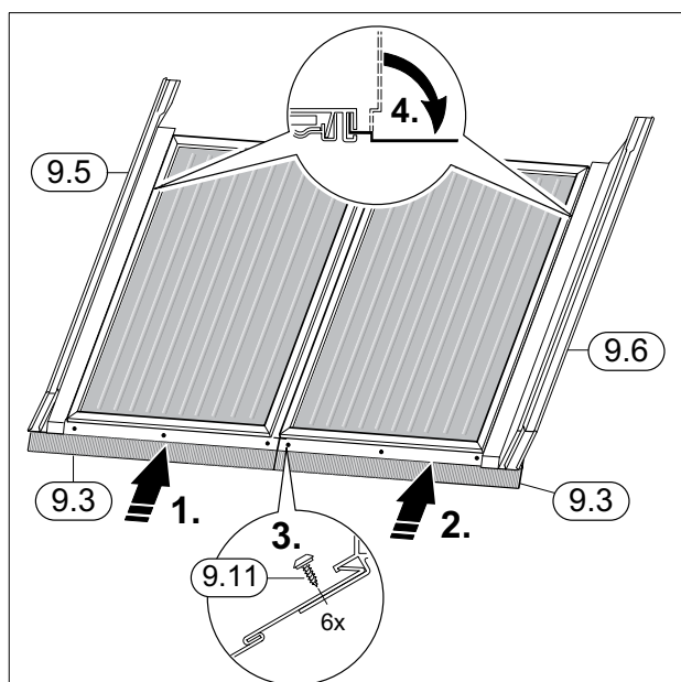
Bild 40 Blechteile unten, links und rechts montieren
