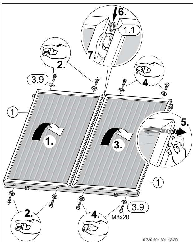
Bild 16 Flachkollektoren einlegen, mit Schrauben sichern und zusammenschließen
