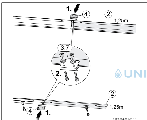
Bild 25 Erweiterung um einen Flachkollektor
