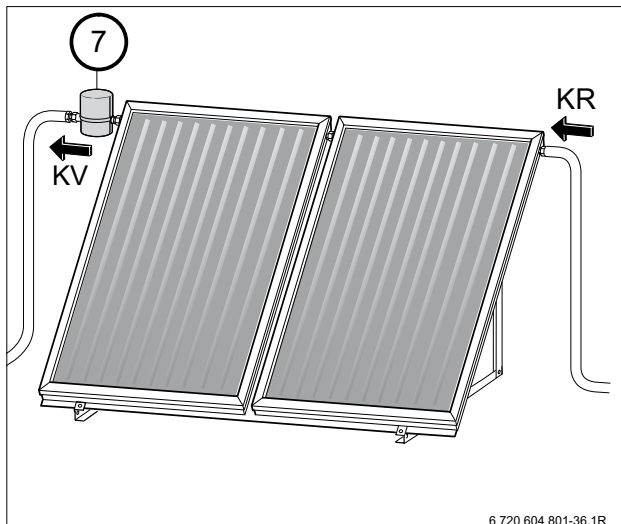
Bild 50 Entlüftertopf und isolierte Rohrleitungen anschließen
