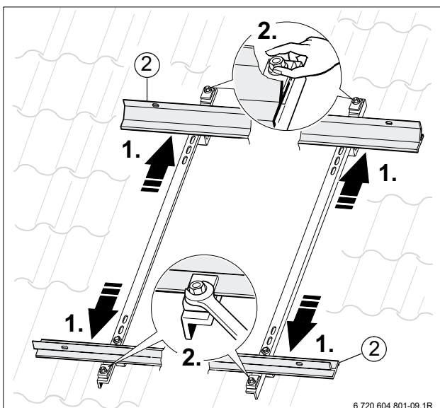
Bild 13 Trageprofile montieren
