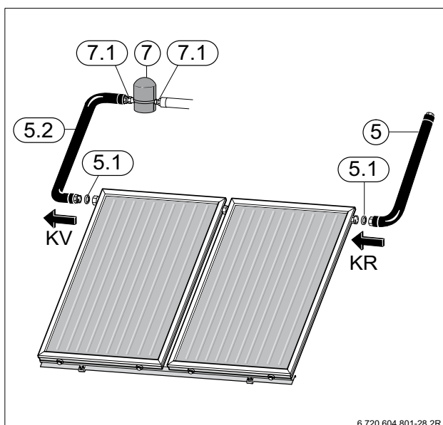
Bild 38 Flexible Schläuche und Entlüftertopf anschließen
