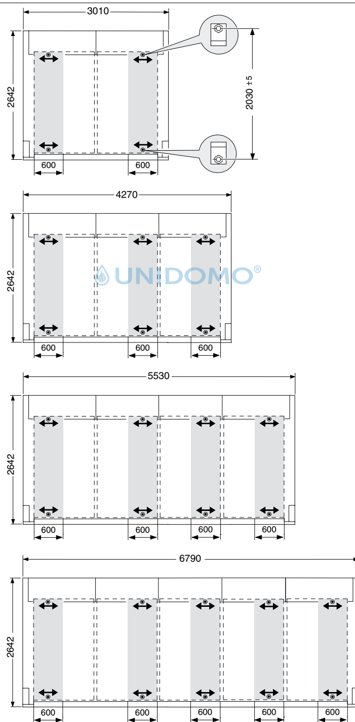
Bild 32 Außenmaße der Blecheinfassung und Toleranzbereiche für die Befestigung der Stockschrauben
