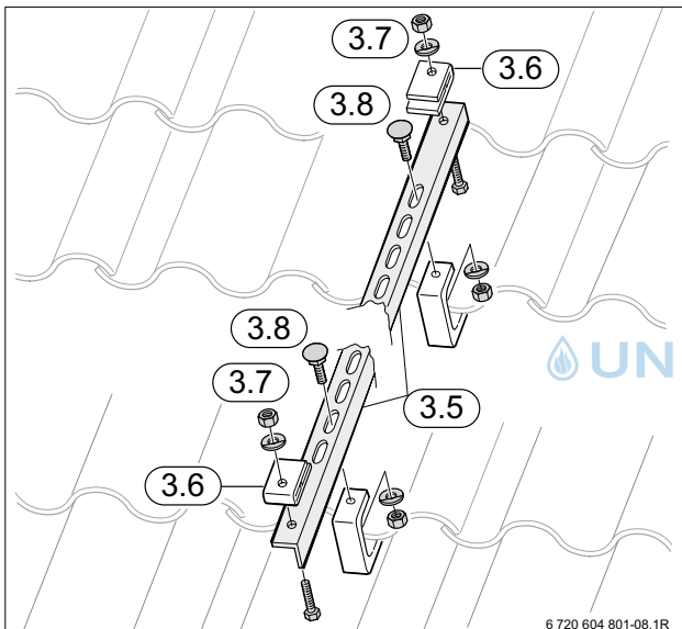
Bild 12 Senkrechte Schiene u. Klemmstücke montieren
