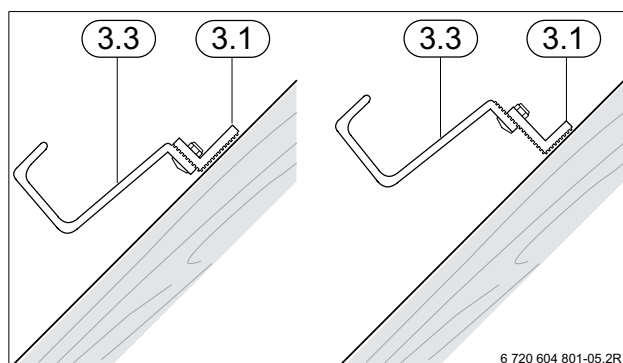
Bild 9 Befestigungsvarianten für Sparrenanker
