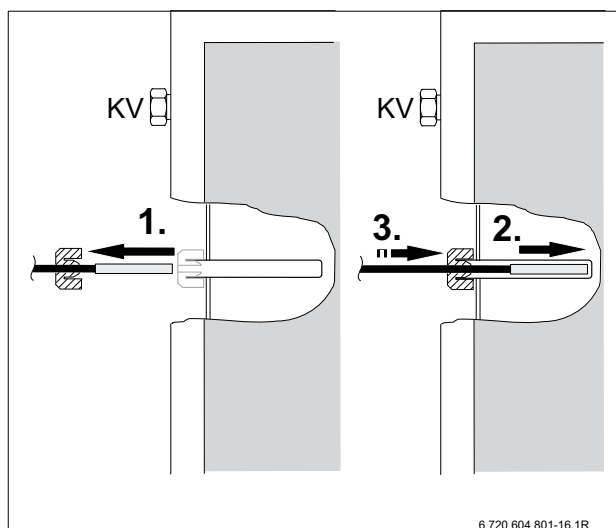
Bild 20 Temperaturfühler in Tauchrohr an der Kollektor-Vorlauf-Seite schieben
