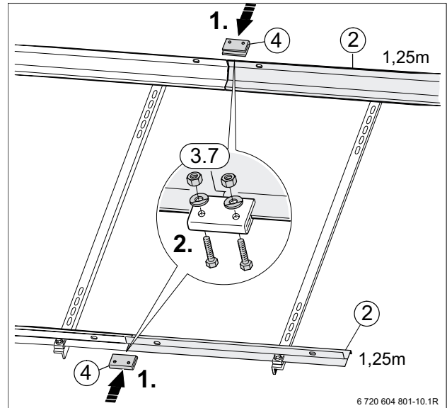
Bild 14 Erweiterung um einen Flachkollektor
