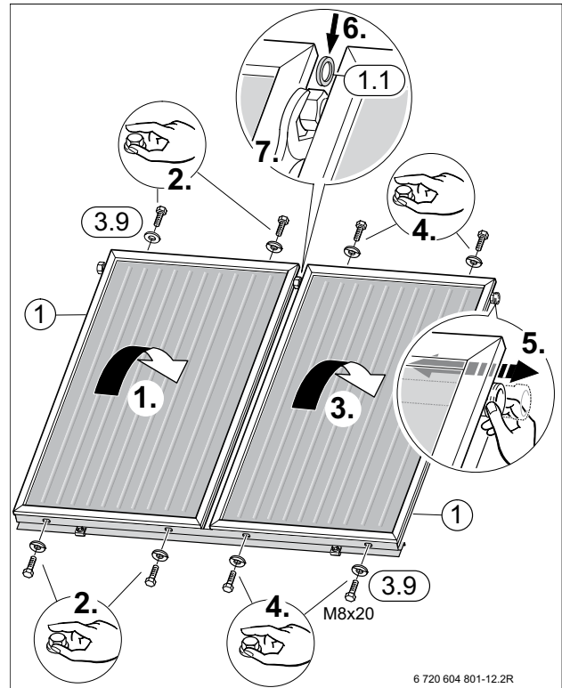
Bild 36 Flachkollektoren einlegen, mit Schrauben sichern und zusammenschließen
