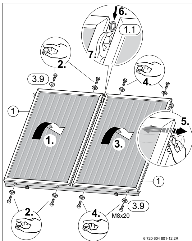
Bild 27 Flachkollektoren einlegen, mit Schrauben sichern und zusammenschließen
