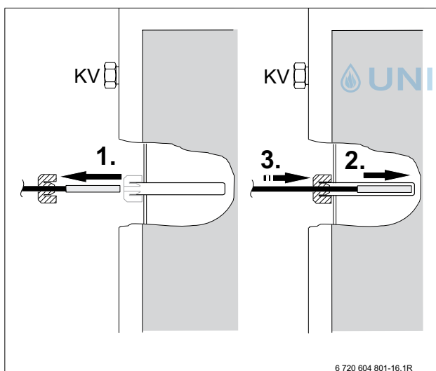
Bild 39 Temperaturfühler in Tauchrohr an der Kollektor-Vorlauf-Seite schieben
