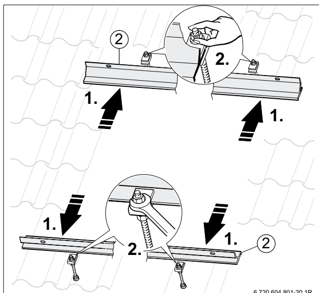
Bild 24 Trageprofile montieren
