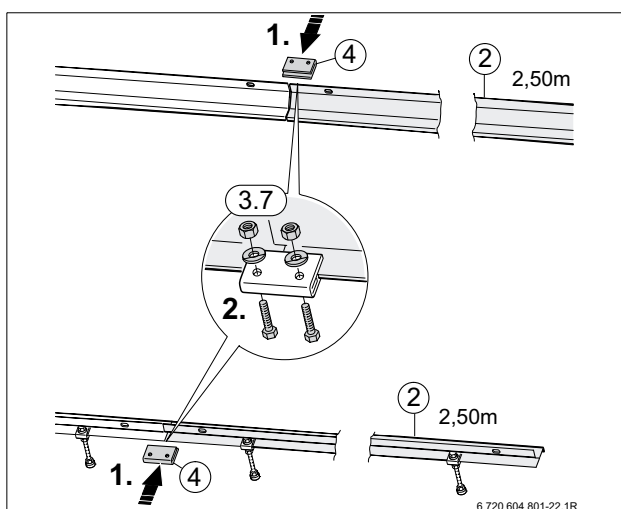
Bild 26 Erweiterung um zwei Flachkollektoren
