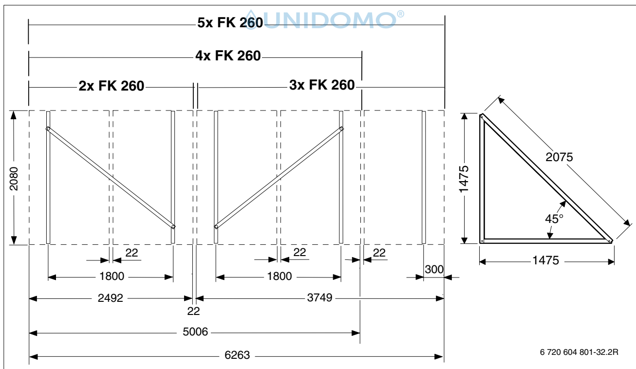
Bild 43 Kollektorfeldmaße für das Flachdachgestell
