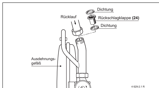
Bild 2: Einbau Rückschlagklappe RK 1 (24)
