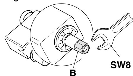
Einstellung 2. Stufe
