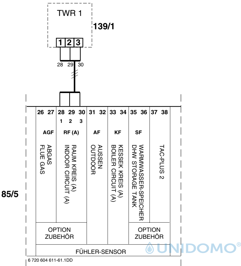
Bild 54 Anschluss ohne Zusatzleiterplatte
