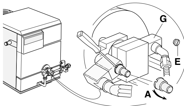
Einstellung 2. Stufe
