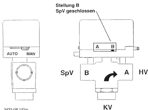
Bild 8: Umsteuerventil an Spannung 24 V AC
