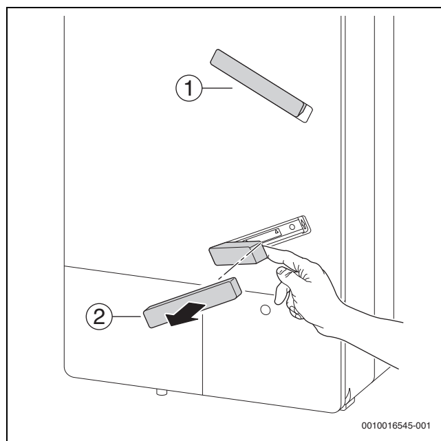
Bild 4 Filterabdeckung abnehmen
