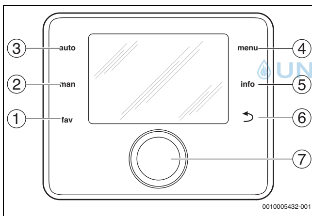
Bild 2 Bedienelemente
