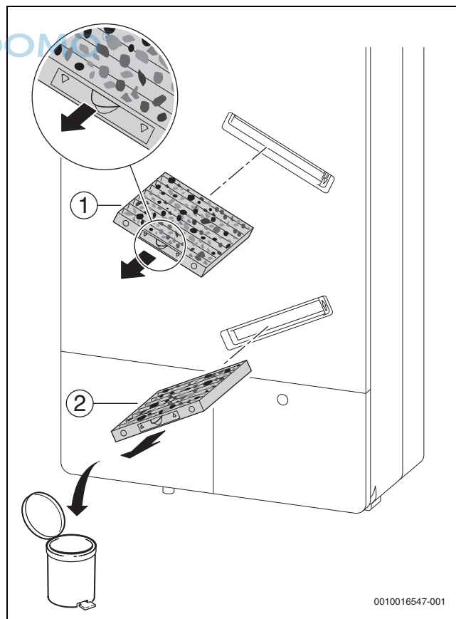
Bild 5 Filter herausziehen
