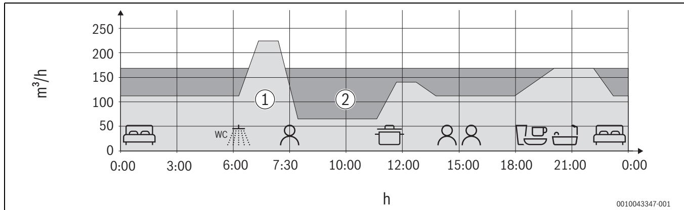
Bild 3 Beispielhafter Vergleich der bedarfsgeführten/manuellen Lüftung
