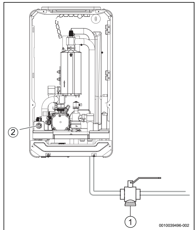
Bild 13 Inneneinheit Compress 5800/6800i 12 E
