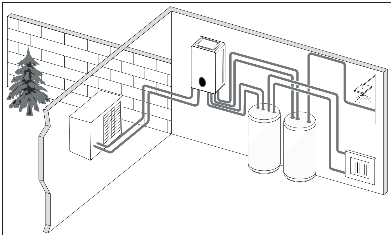
Bild 7 Wärmepumpe AW OR, Inneneinheit Compress 5800/6800i 12 E mit elektrischem Zuheizter und externem Warmwasserspeicher
