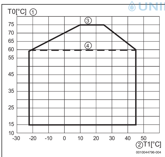
Bild 4 Wärmepumpe im Heizbetrieb ohne Zuheizung
