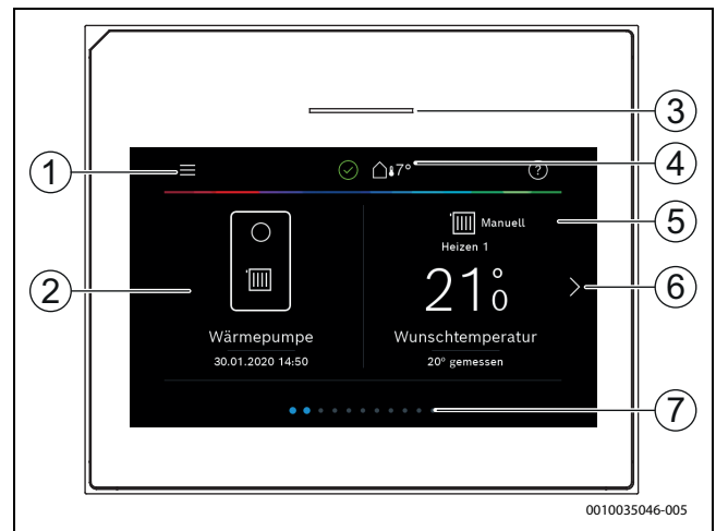
Bild 8 Bedienfeld
