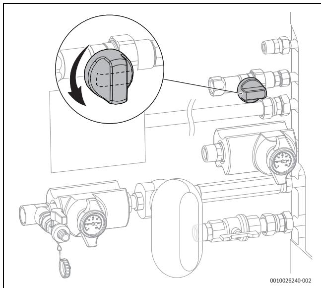
Bild 4 Gashahn öffnen
