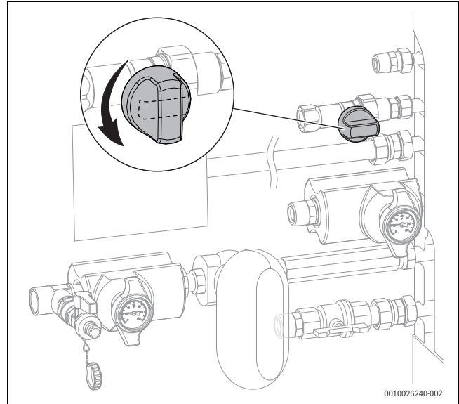
Bild 5 Gashahn öffnen
