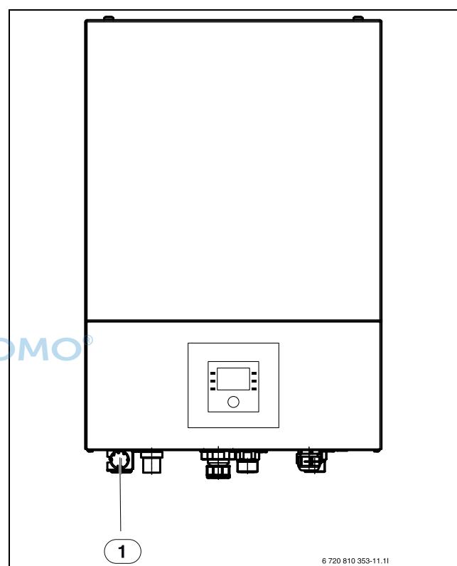
Bild 5 Inneneinheit ASB
