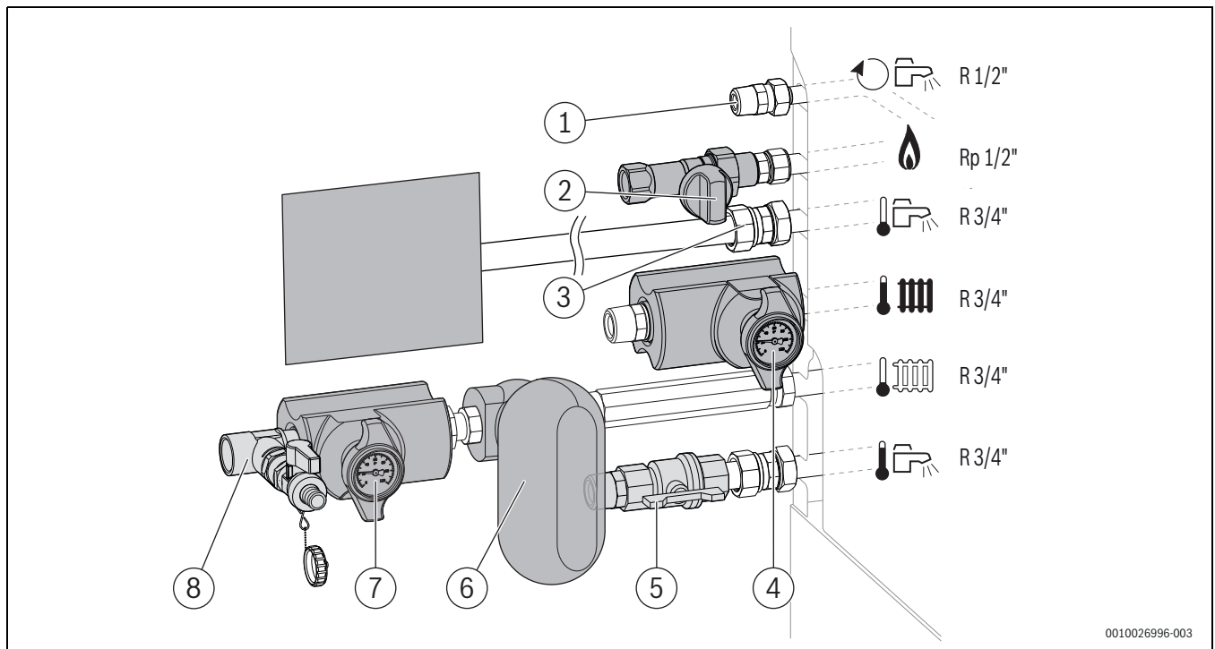
Bild 11 Beispiel: Gas- und wasserseitiger Anschluss mit dem Anschluss-Set Hähne (Zubehör CS 28-1) auf der linken Seite
