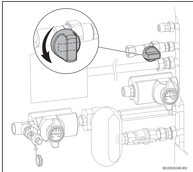
Bild 9 Gashahn öffnen
