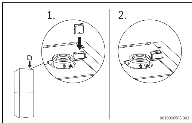
Bild 6 Control Key in den Key-Halter einstecken
