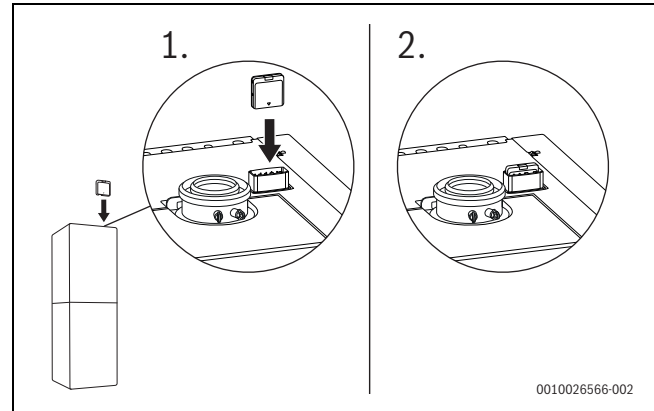
Bild 6 Control Key in den Key-Halter einstecken
