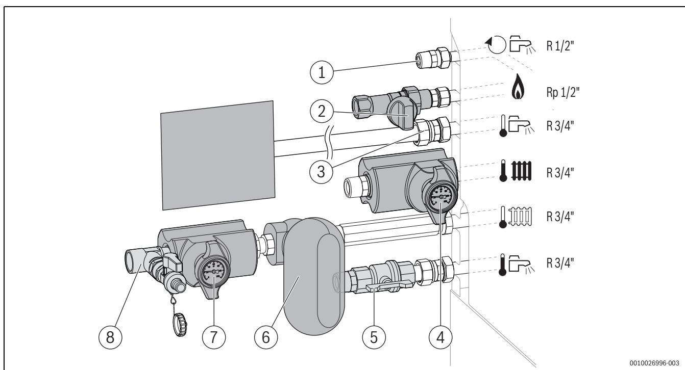
Bild 11 Beispiel: Gas- und wasserseitiger Anschluss mit dem Anschluss-Set Hähne (Zubehör CS 28-1) auf der linken Seite
