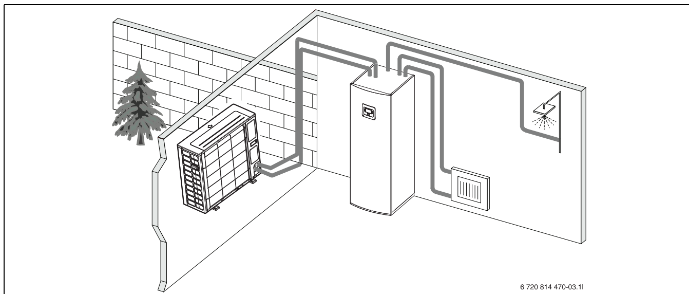
Bild 2 Wärmepumpe Ausseneinheit, Inneneinheit ASM/ASMS mit integriertem Warmwasserspeicher und elektrischem Zuheizter
