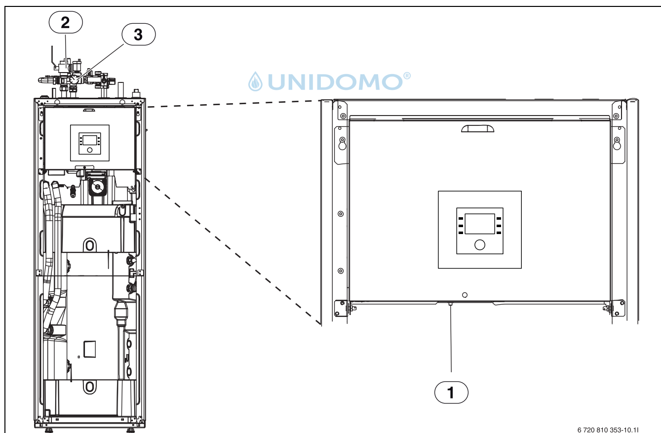
Bild 5 Inneneinheit ASM / ASMS
