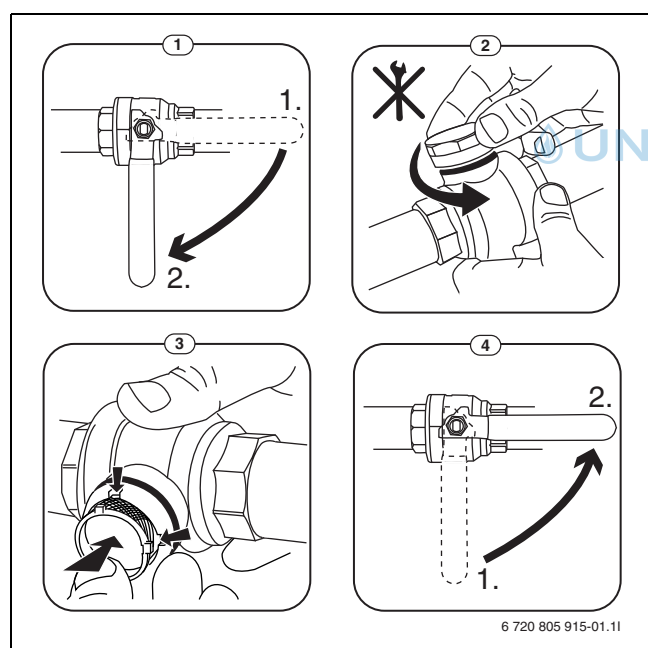
Bild 6 Siebreinigung
