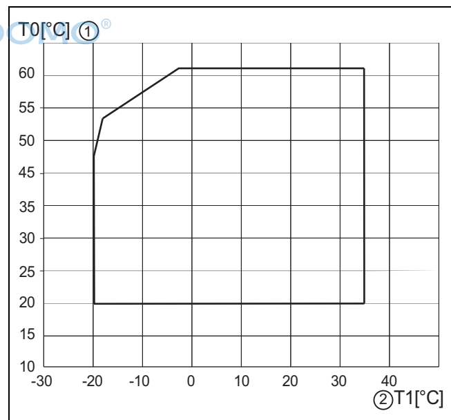
Bild 1 Wärmepumpe ohne Zuheizer
