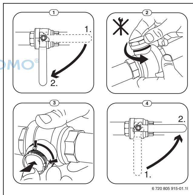
Bild 8 Siebreinigung
