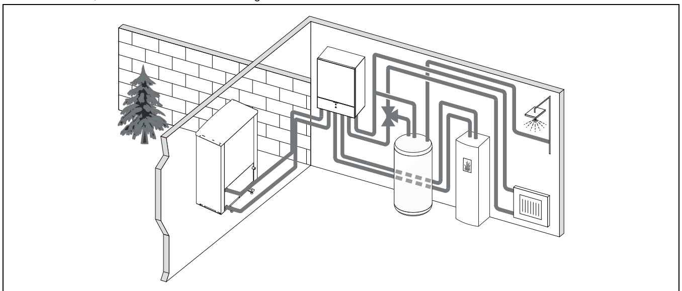
Bild 3 Wärmepumpe Compress 7000i AW, Inneneinheit AWB ohne elektrischen Zuheizung, externer Warmwasserspeicher und externer Zuheizung
