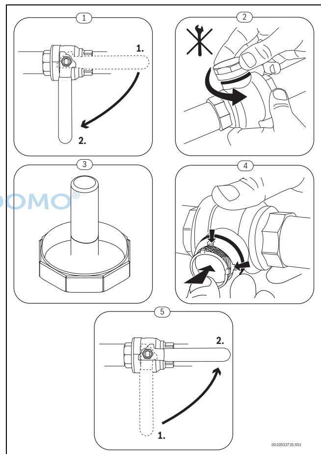
Bild 5 Siebreinigung
